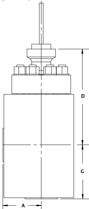
Figura 8. Dimensiones típicas de la válvula angular de fundición CL2500 de 6 etapas NotchFlo DST (consultar también la tabla 26)
