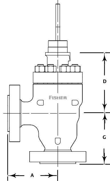
Figura 5. Dimensiones típicas de la válvula de ángulo fundido de 4 etapas CL1500 NotchFlo DST (ver también las tablas 21 y 22)
