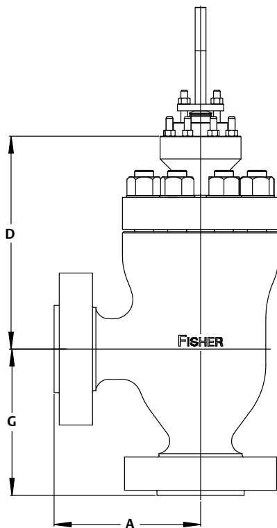
Figura 8. Dimensiones típicas de la válvula angular de fundición CL2500 de 6 etapas NotchFlo DST (consultar también la tabla 26)
