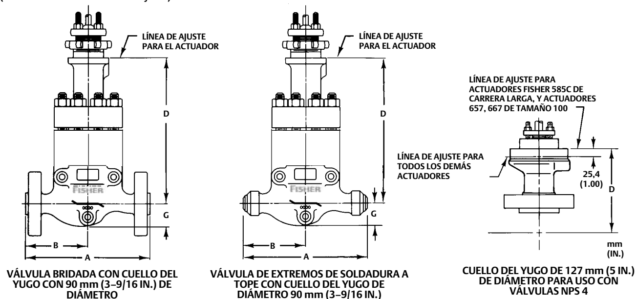
Figura 3. Dimensiones típicas de la válvula de globo CL900 y CL1500 ≤ NPS 4 de cuatro etapas NotchFlo DST (ver también las tablas 16 y 17)
