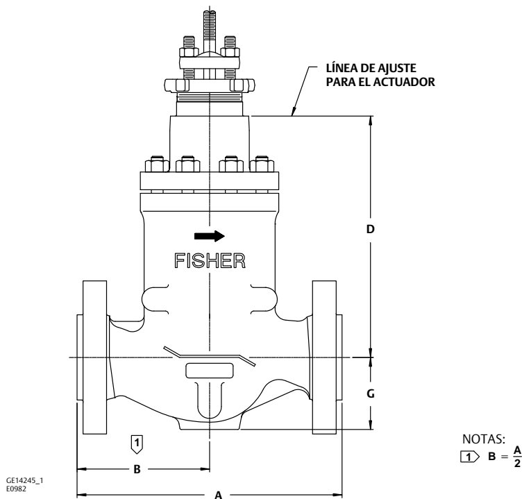
Figura 2. Dimensiones típicas de la válvula CL300 y CL600 de 3 etapas NotchFlo DST (ver también las tablas 14 y 15)
