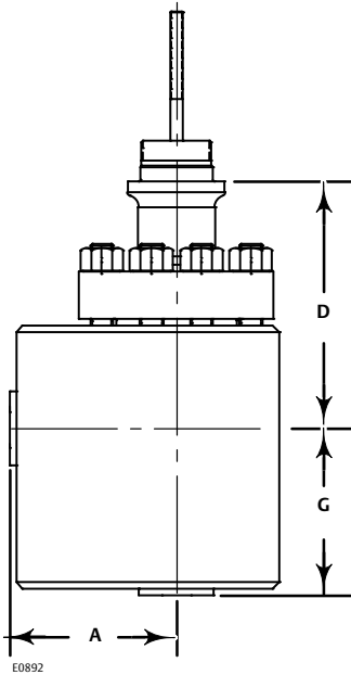
Figura 4. Dimensiones típicas de las válvulas de ángulo CL300 de 3 etapas, CL600 de 3 etapas, CL900 de 4 etapas y CL1500 de 4 etapas NotchFlo DST (ver también las tablas 18, 19 y 20)
