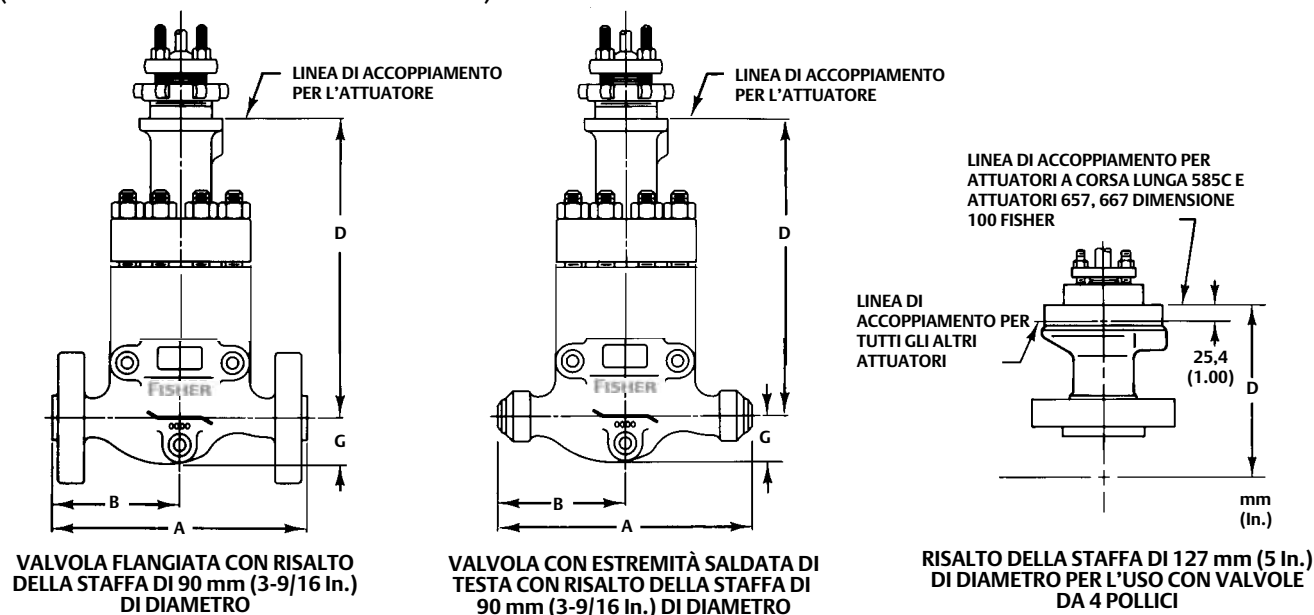
Figura 3. Dimensioni tipiche delle valvole a globo NotchFlo DST CL900 e CL1500 ≤ 4 pollici, a 4 stadi (fare riferimento anche alle Tabelle 16 e 17)
