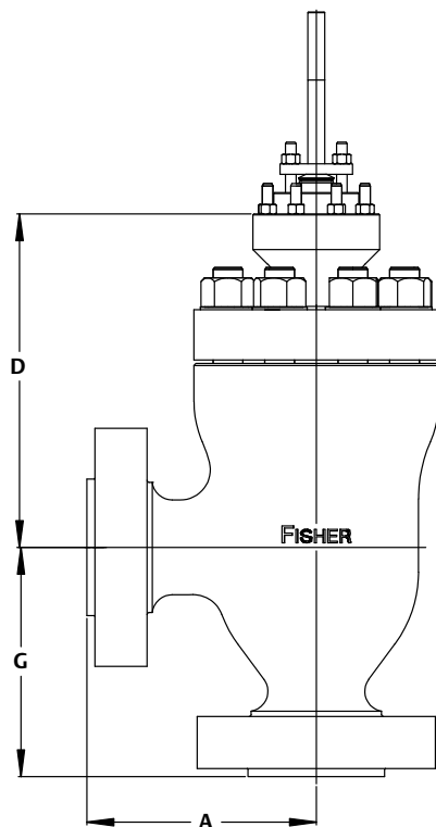
Figura 8. Dimensioni tipiche della valvola ad angolo fusa NotchFlo DST CL1500 a 6 stadi (fare riferimento anche alla Tabella 26)
