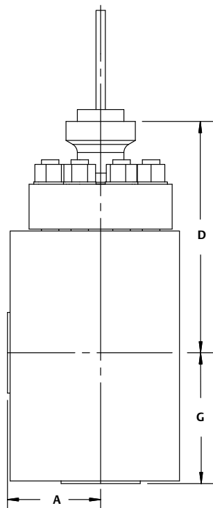
Figura 7. Dimensioni tipiche della valvola ad angolo forgiata NotchFlo DST CL1500 a 6 stadi (fare riferimento anche alla Tabella 25)
