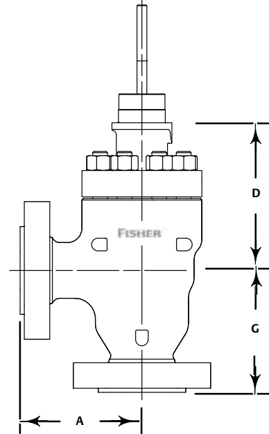
Figura 5. Dimensioni tipiche della valvola fusa ad angolo NotchFlo DST CL1500 a 4 stadi (fare riferimento anche alle Tabelle 21 e 22)
