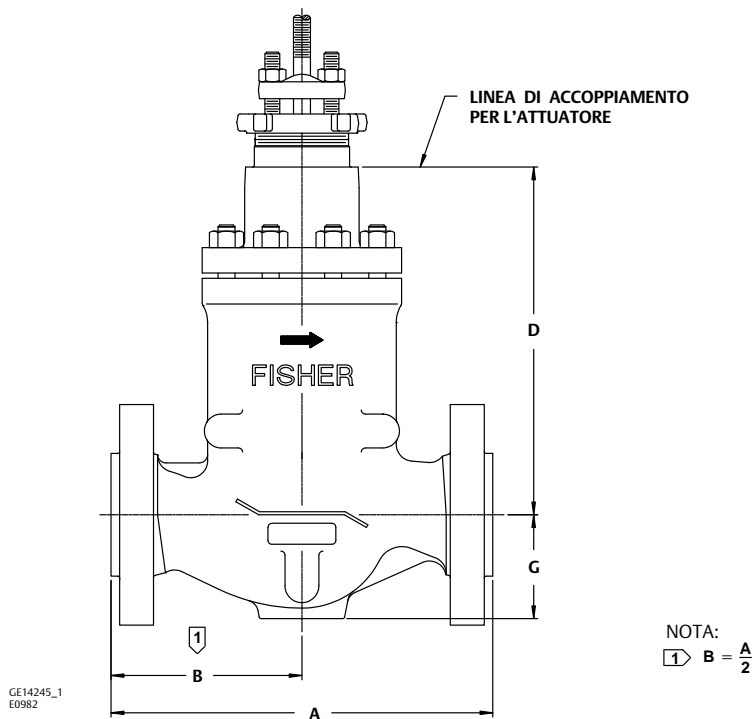
Figura 2. Dimensioni tipiche della valvola NotchFlo DST CL300 e CL600 a 3 stadi (fare riferimento anche alle Tabelle 14 e 15)
