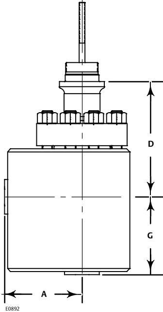
Figura 4. Dimensioni tipiche della valvola ad angolo NotchFlo DST CL300 e CL600 a 3 stadi, CL900 e CL1500 a 4 stadi (fare riferimento anche alle Tabelle 18, 19 e 20)
