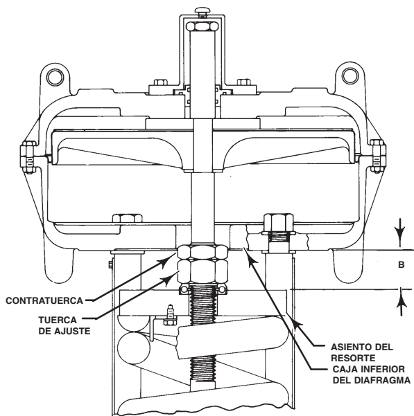
Figura 3. Dimensión B para el ajuste del resorte
