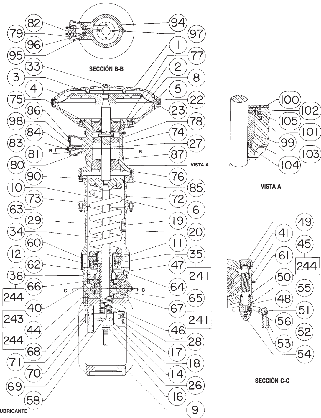
Figura 7. Actuador Fisher® 657, tamaño 80, con volante de montaje lateral y amortiguador hidráulico
