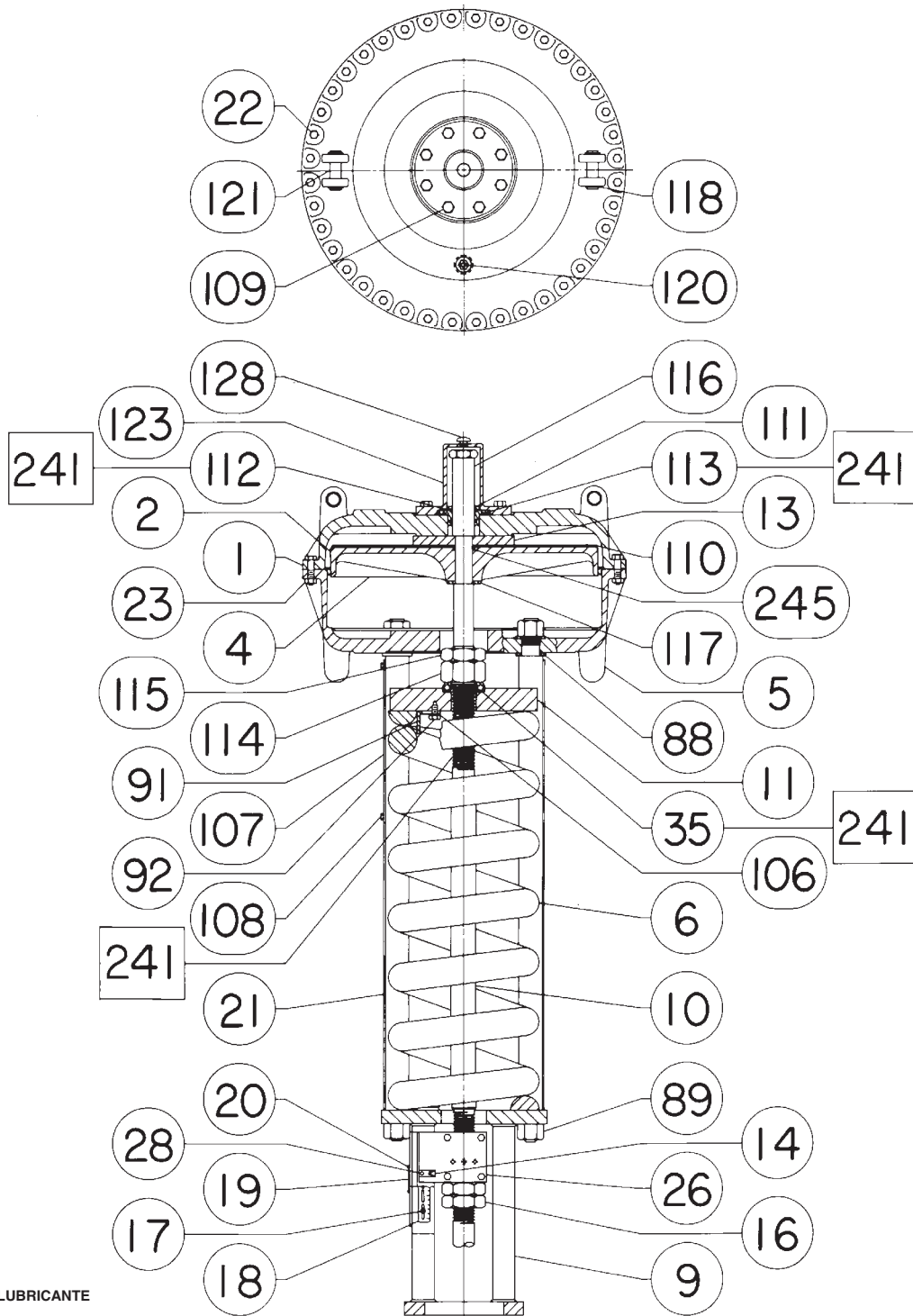
Figura 5. Actuador Fisher® 657, tamaño 100
