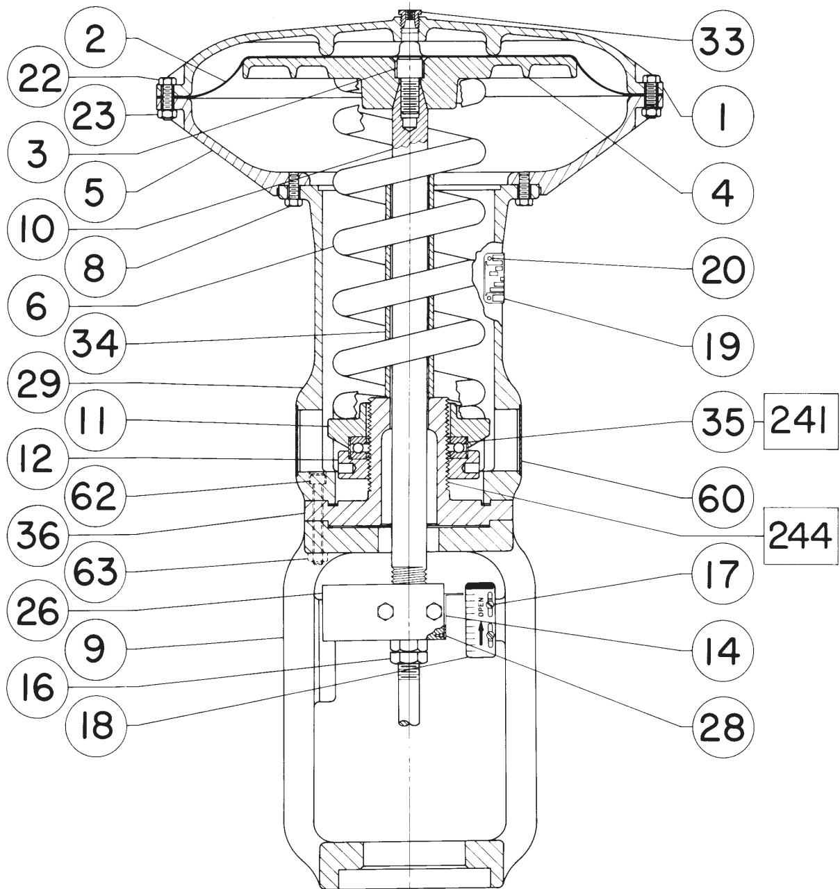
Figura 4. Actuador Fisher® 657, tamaño 80
