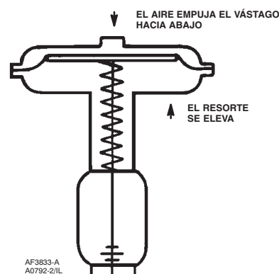
Figura 2. Representación esquemática del actuador Fisher® 657
