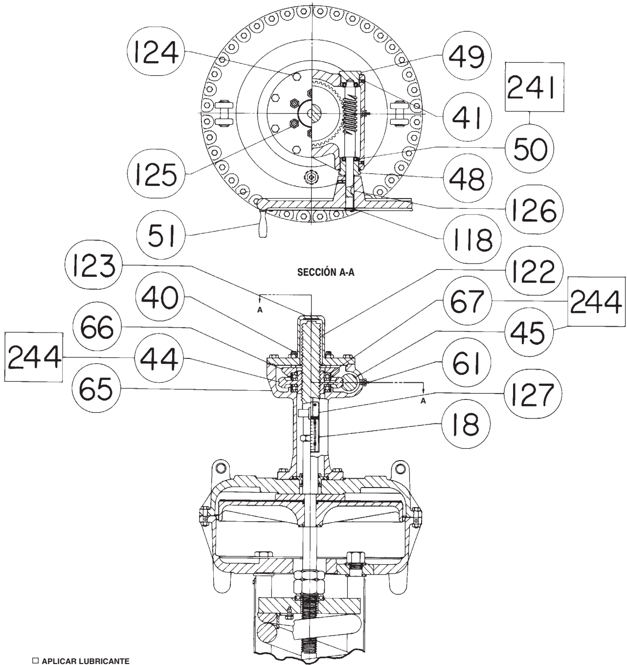
Figura 8. Volante de montaje superior para actuador tamaño 100
