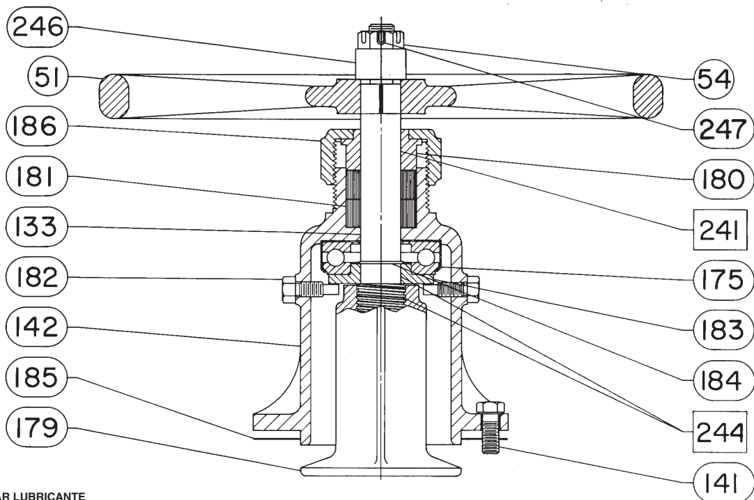
Figura 6. Volante de montaje superior para actuadores tamaño 80
