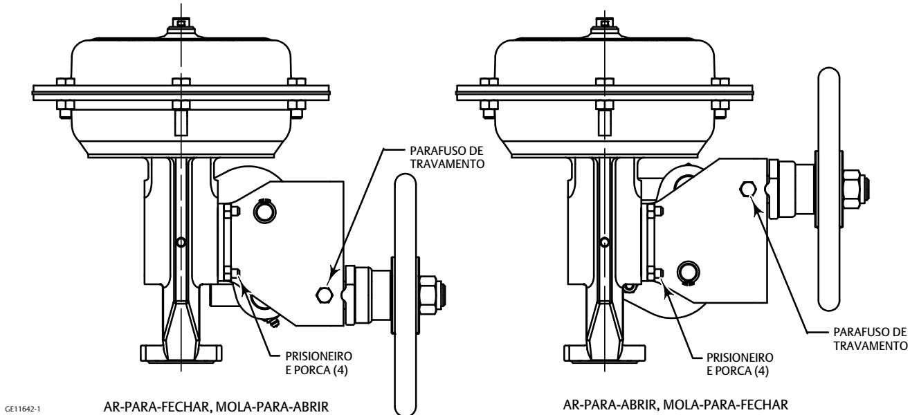
Figura 6. Montagem do Volante GX Fisher
