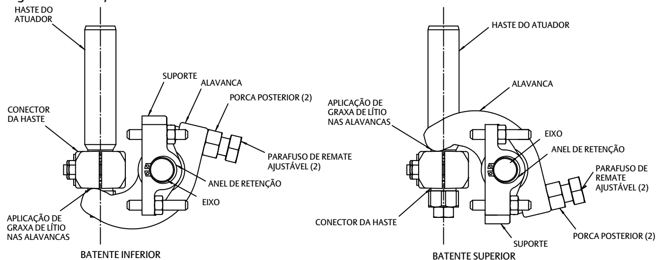
Figura 9. Orientação do Batente de Deslocamento GX Fisher
