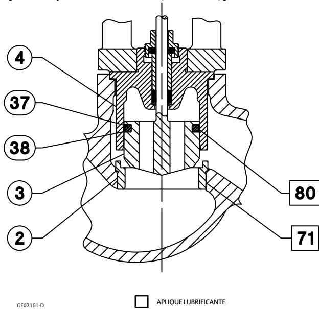
Figura 10. Interno Balanceado GX [Padrão para DN 80 e 100 (NPS 3 e 4)] Fisher
