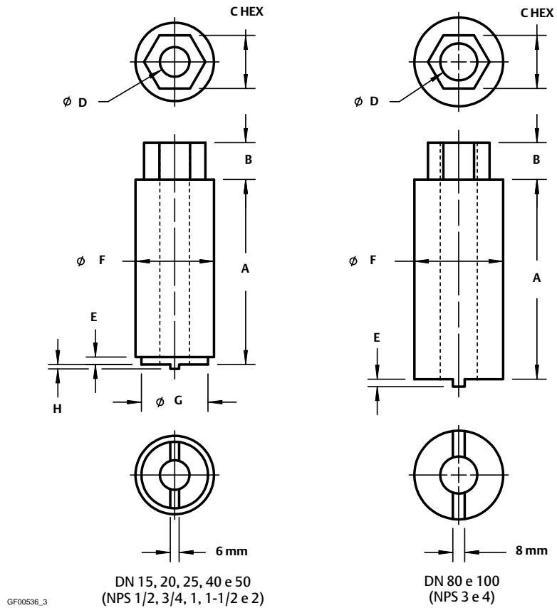
Figura 26. Remoção da Porca do Fole e Ferramenta de Instalação
