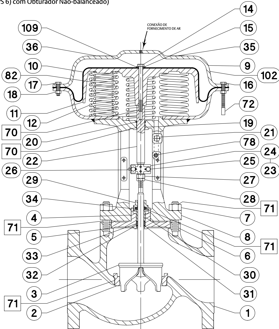
Figura 21. Conjunto do Sistema da Válvula de Controle e Atuador GX Fisher Ar-para-Fechar (Mola-para-Abri r ) (DN 150 (NPS 6) com Obturador Não-balanceado)
