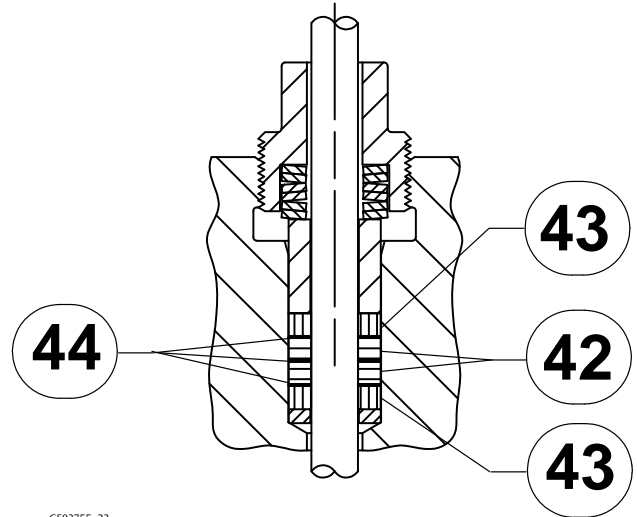
Figura 17. Gaxeta ULF Grafite ENVIRO-SEAL GX Fisher DN150 somente (NPS 6 somente)
