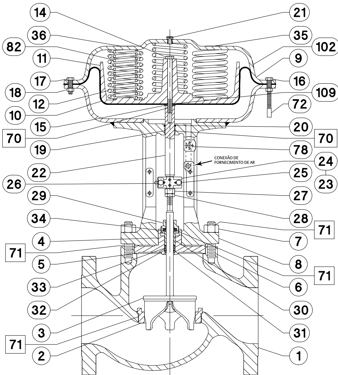
Figura 19. Conjunto do Sistema da Válvula de Controle e Atuador GX Fisher Ar-para-Abrir (Mola-para-Fechar) (DN 150 (NPS 6) com Obturador Não-balanceado)
