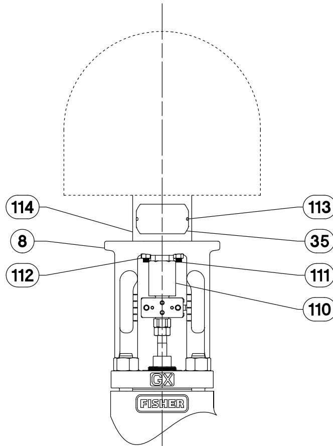
Figura 28. Montagem do Atuador Elétrico GX Fisher
