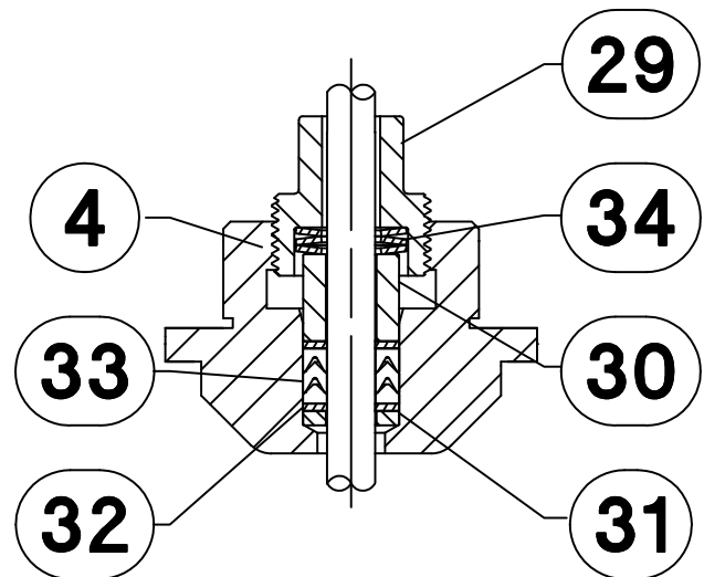
Figura 15. Gaxetas de PTFE ENVIRO-SEAL Fisher GX DN5 a DN150 (NPS 1/2 a 6)
