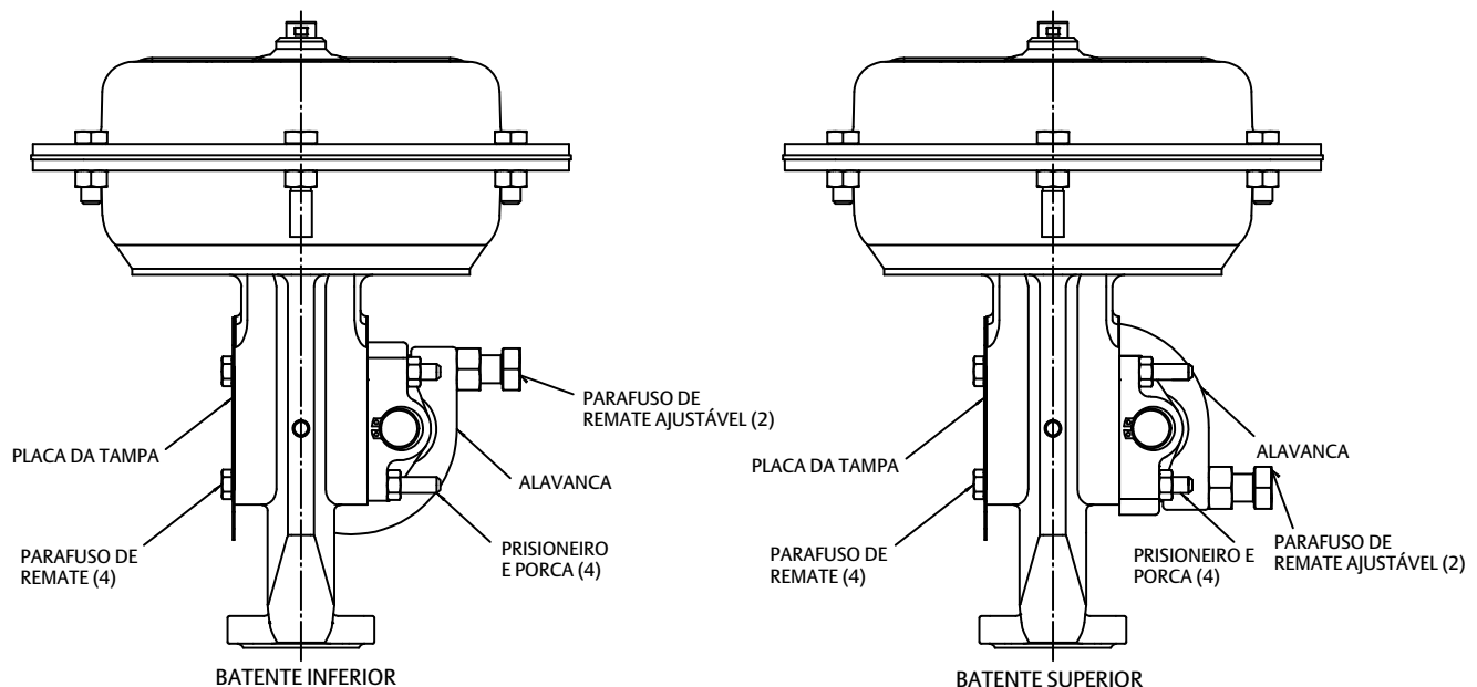
Figura 8. Conjunto do Batente de Deslocamento GX Fisher
