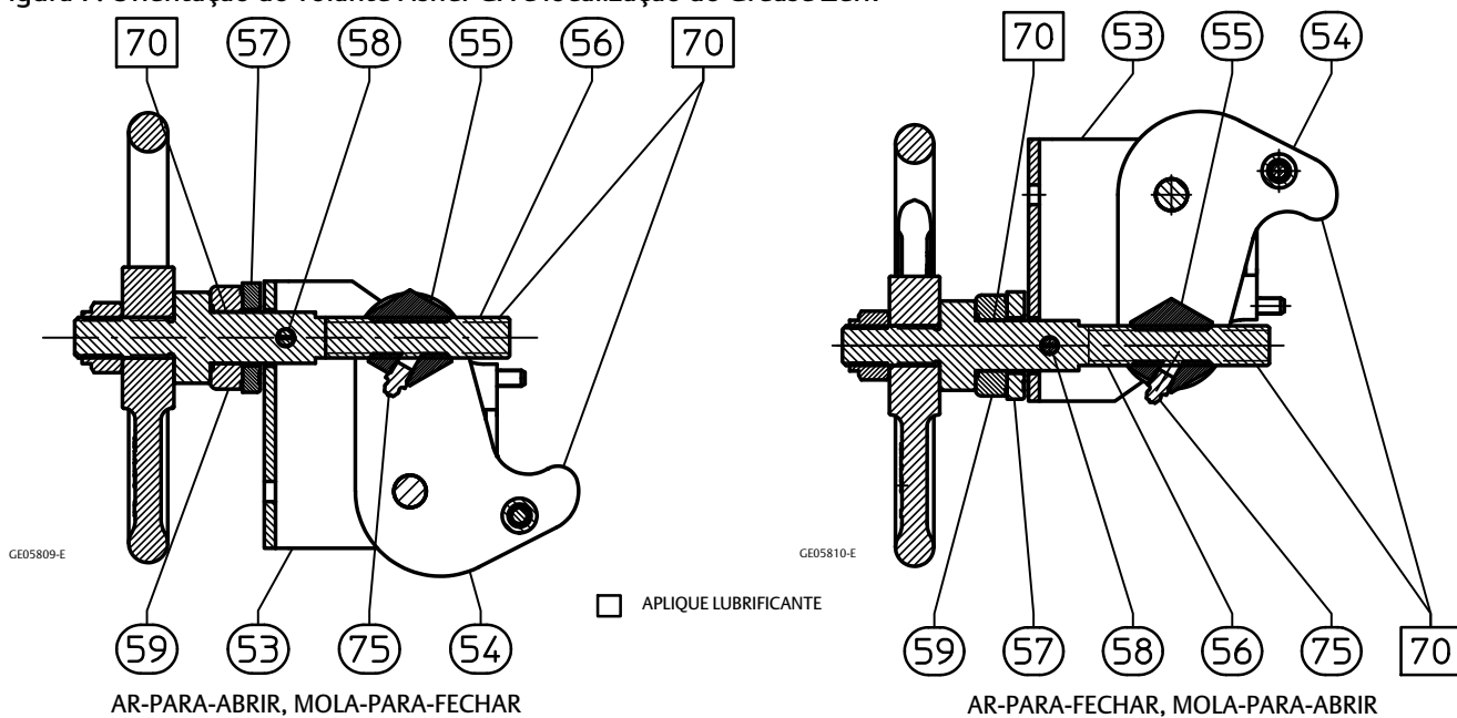
Figura 7. Orientação do volante Fisher GX e localização do Grease Zerk
