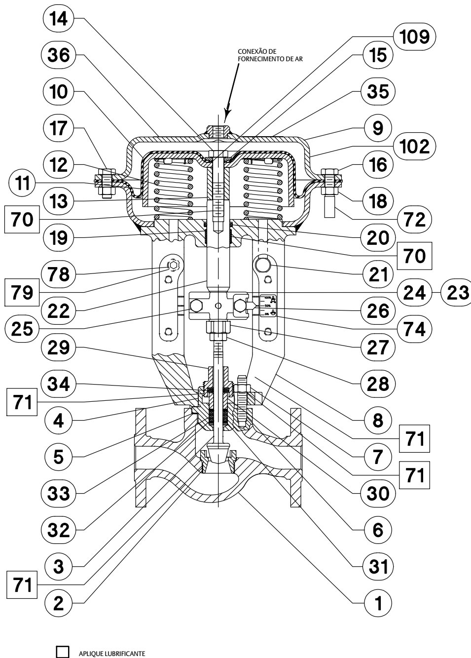
Figura 20. Conjunto do Sistema da Válvula de Controle e Atuador GX Fisher Ar-para-Fechar (Mola-para-Abriir) (DN 25 (NPS 1) com Obturador Não-balanceado)
