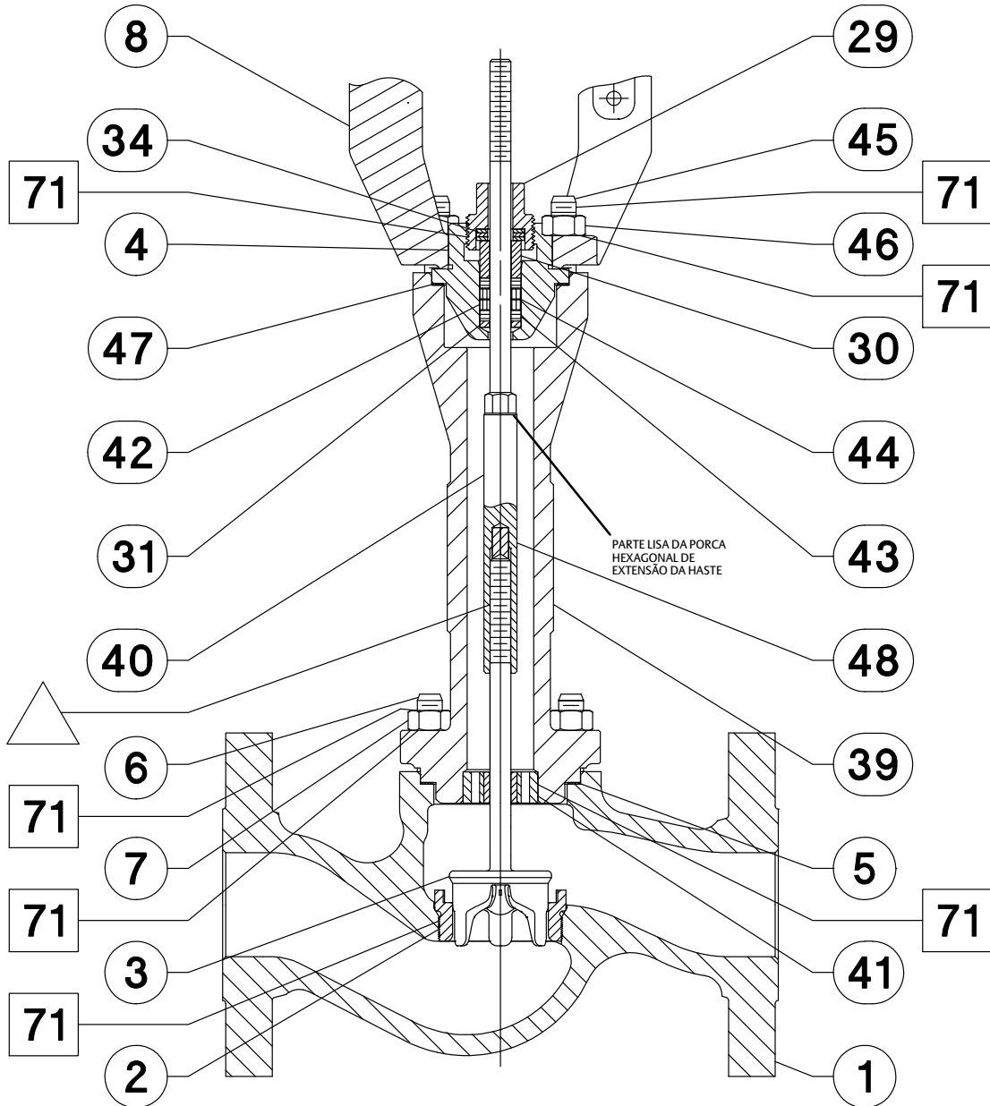
Figura 22. Cobertura de extensão com gaixetas ULF Grafite ENVIRO-SEAL
