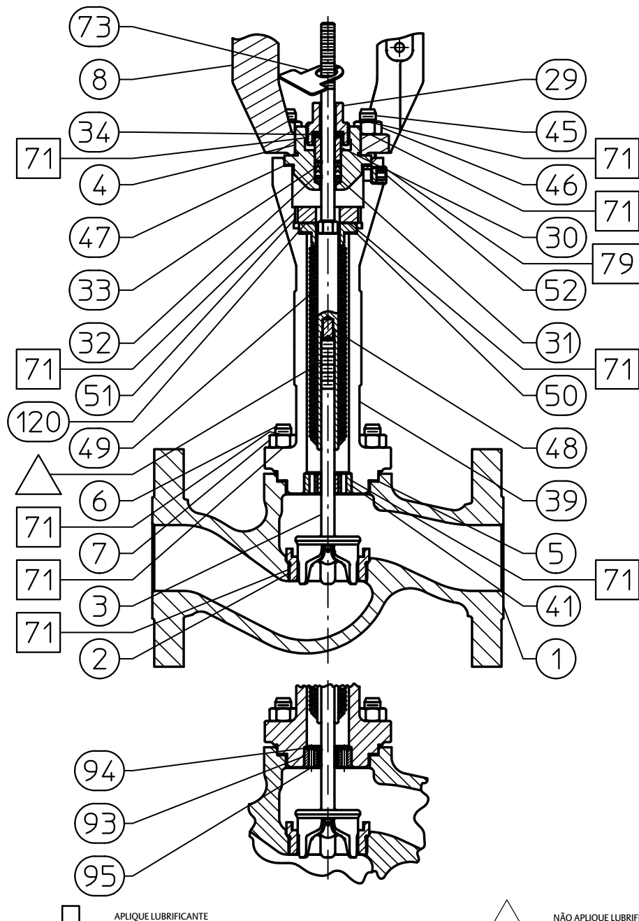
Figura 23. Cobertura de extensão de folie com empanques PTFE ENVIRO-SEAL
