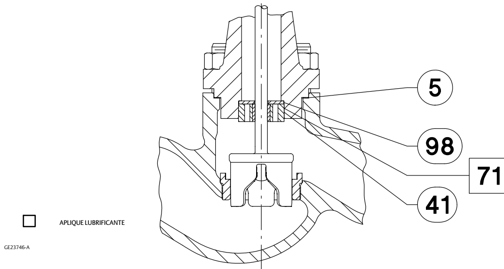
Figura 24. Cobertura de Extensão Criogênica
