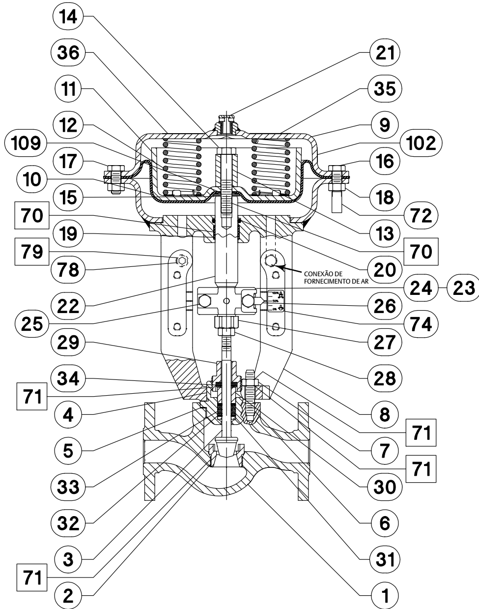
Figura 18. Conjunto do Sistema da Válvula de Controle e Atuador GX Fisher Ar-para-Abrir (Mola-para-Fechar) (DN 25 (NPS 1) com Obturador Não-balanceado)
