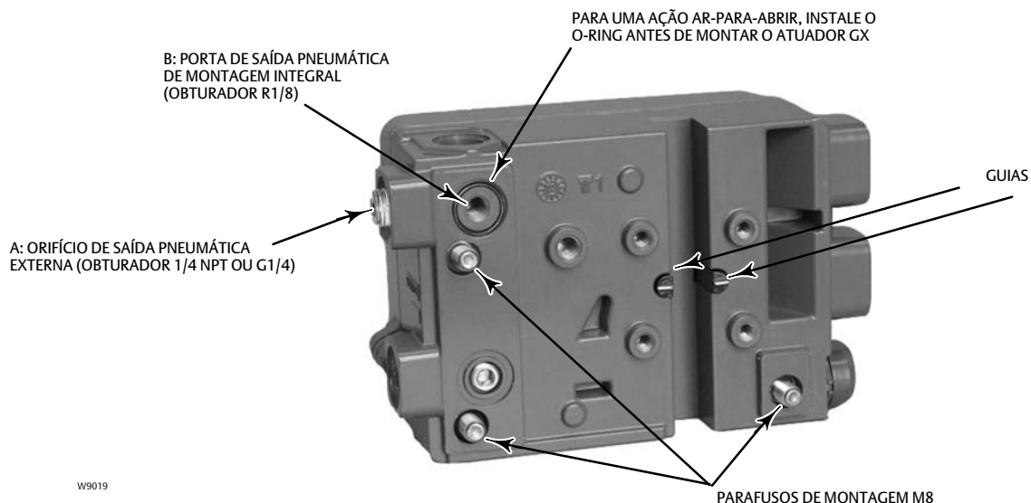
Figura 4. Detalhes de Montagem do Controlador de Válvula Digital DVC2000
