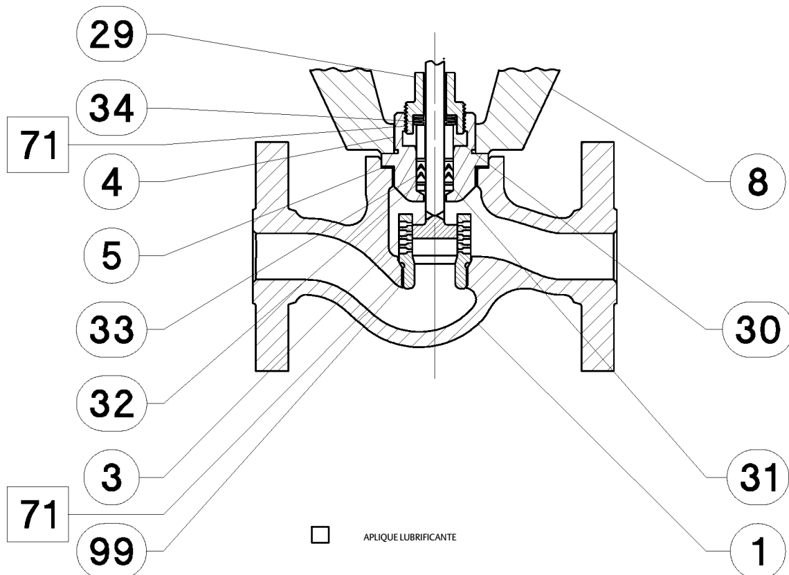
Figura 25. Guarnição Cavitol III Fisher, DN25, DN40 e DN50 (NPS 1, NPS 1-1/2 e NPS 2)
