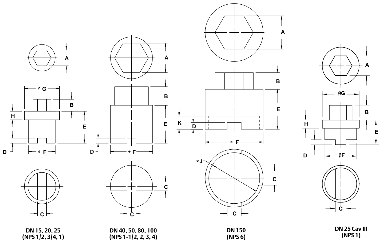
Figura 5. Remoção da Sede e Ferramenta de Instalação
