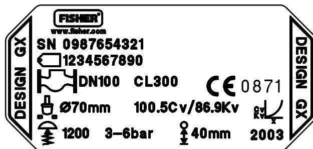
Figura 2. Exemplos de Placa de Identificação GX Fisher (peça 35)
