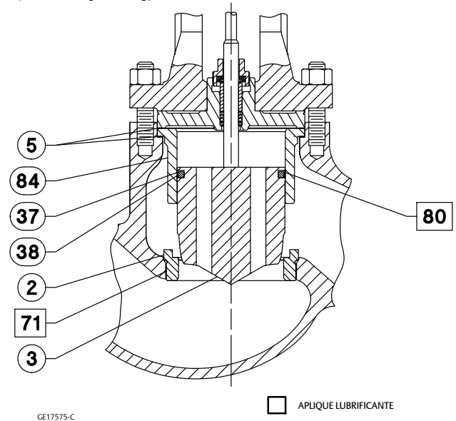
Figura 11. Interno Balanceado GX (DN 150 [NPS 6]) Fisher
