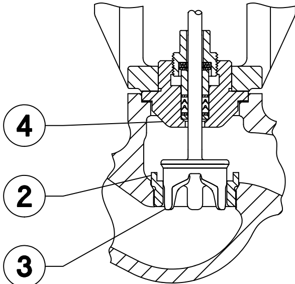
Figura 12. Interno Não-balanceado GX Fisher Guiados pela Porta (DN 40 a 150 [NPS 1-1/2 a 6])
