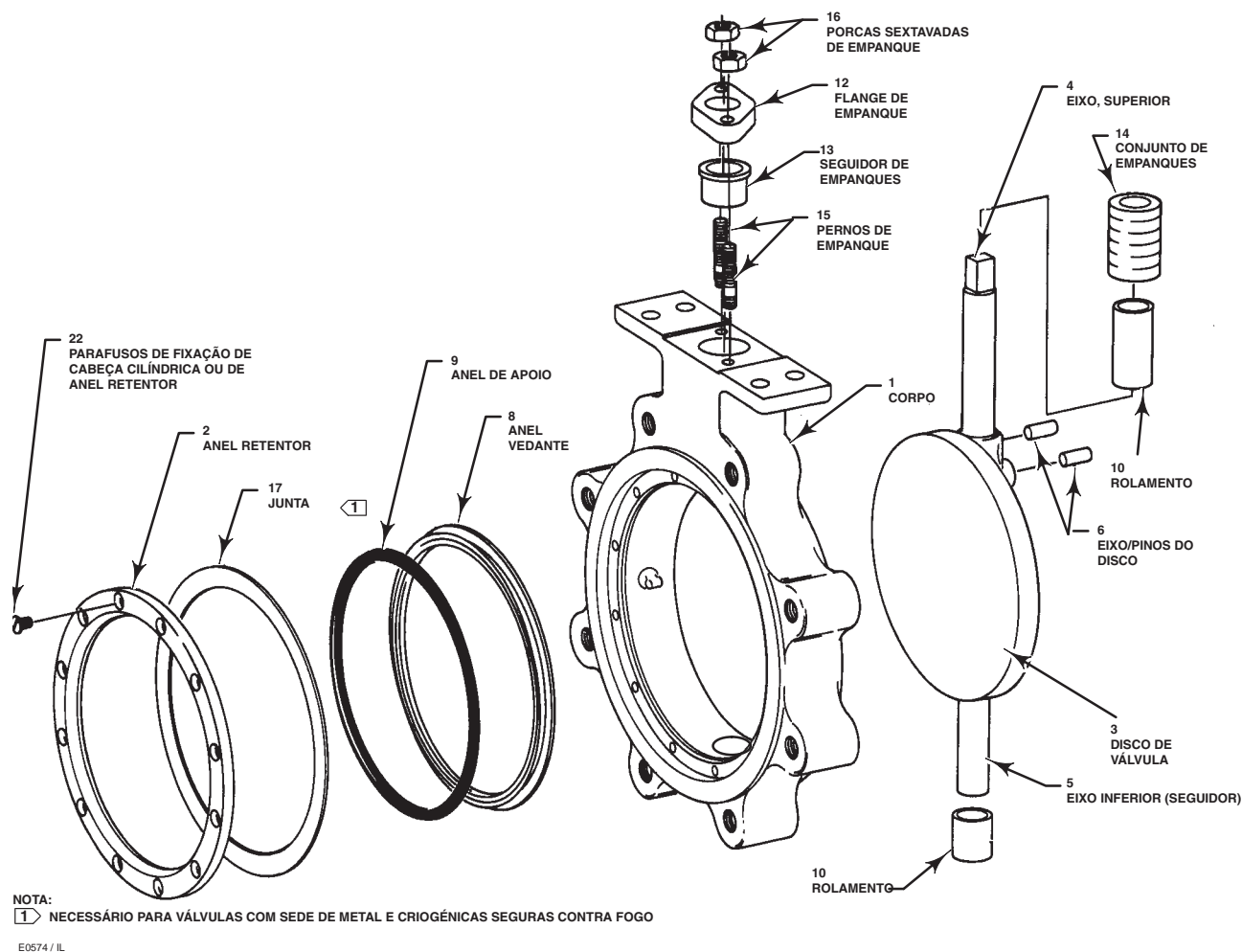
Figura 9. Montagem Típica da Válvula Tipo A11
