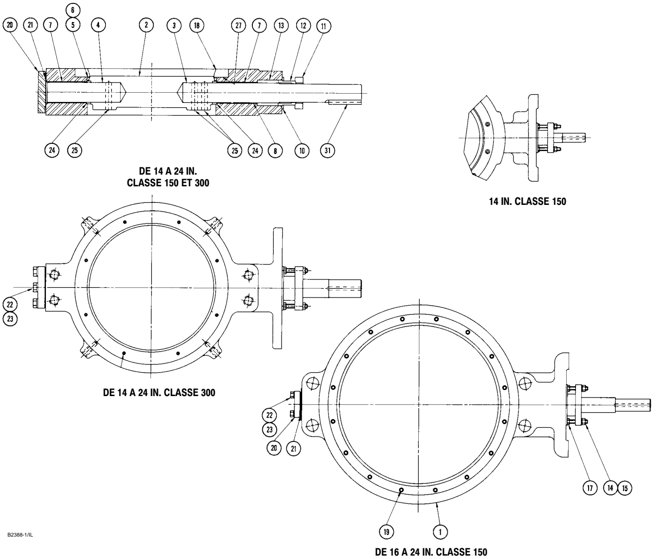
Figure 9. Ensemble de vanne type à insérer entre brides (sandwich) type A31A
