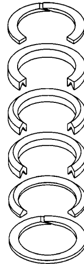
ORDRE D'EMPLAGE DES BAGUES DE GARNITURE EN PTFE
