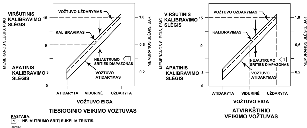
5 pav. Tipinis vožtuvo atsakas į nejautrumo sritį
