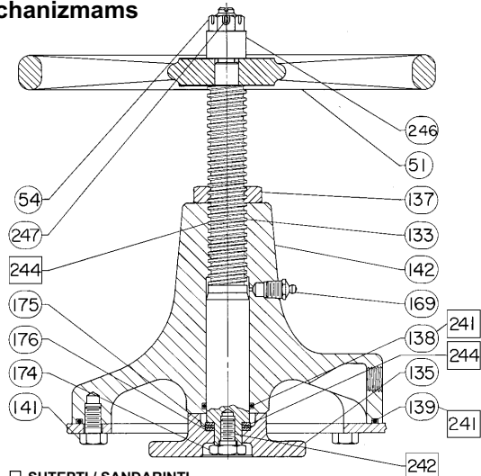
12 pav. Viršuje montuojamas rankinio valdymo blokas, skirtas 70/70i ir 87 dydžio pavarus mechanizmams
