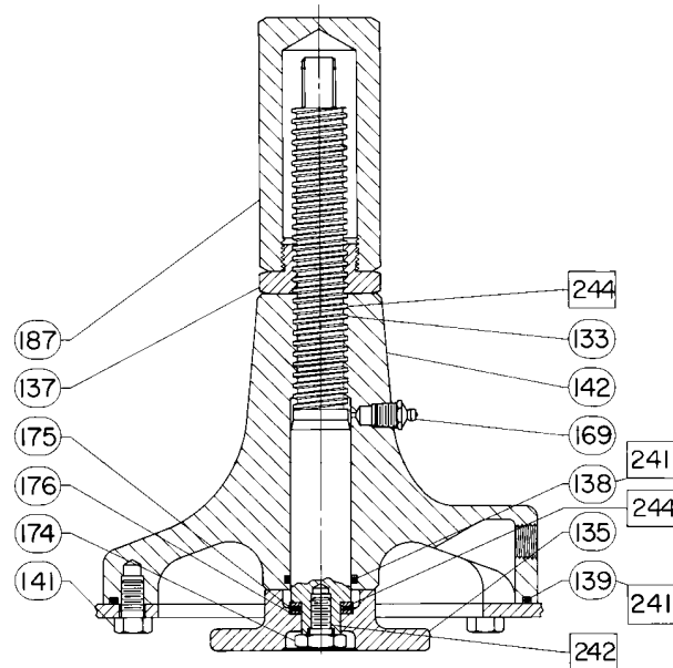
19 pav. Prie gaubto montuojamas reguliuojamasis viršutinės eigos stabdiklis, skirtas 70/70i ir 87 dydžio pavarus mechanizams (1 tipas)
