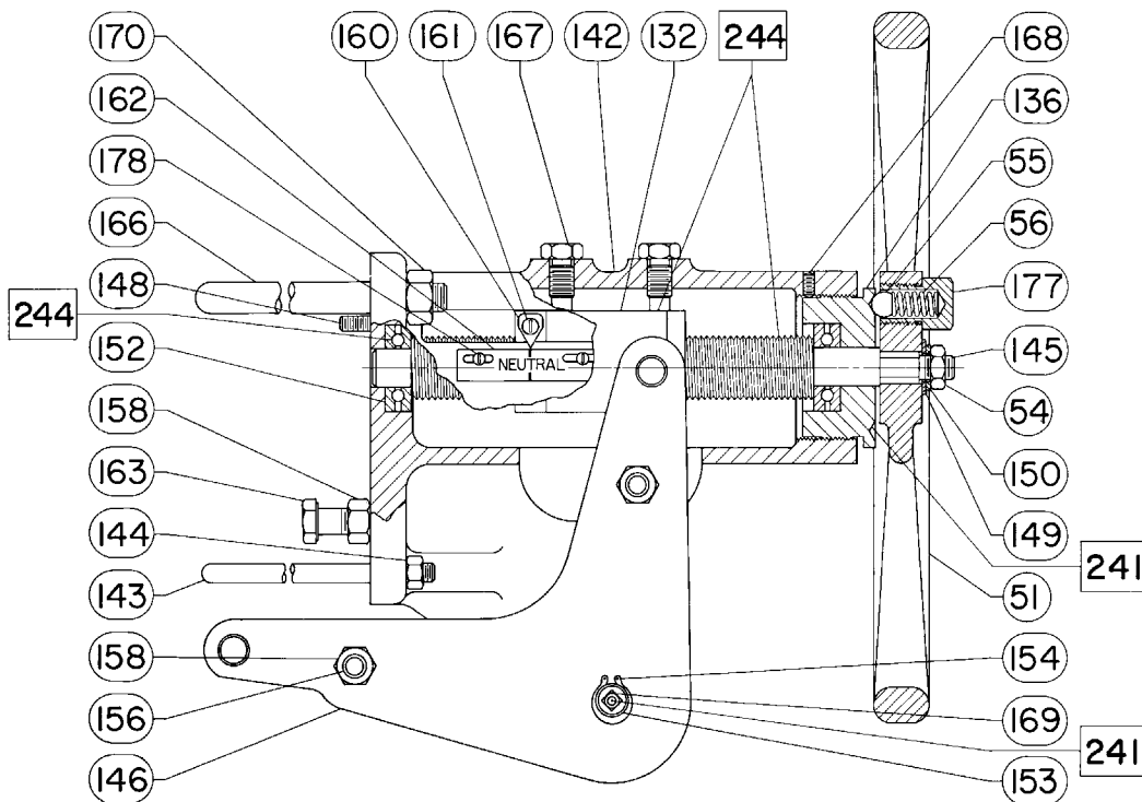
15 pav. Šone montuojamas rankinio valdymo blokas, skirtas 45, 46, 50 ir 60 dydžio pavaros mechanizmams
