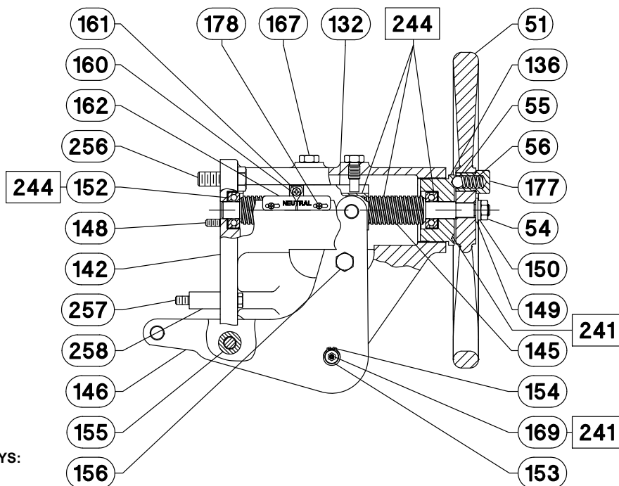
16 pav. Šone montuojamas rankinio valdymo blokas, skirtas 45i, 46i, 50i ir 60i dydžio pavaros mechanizmams
