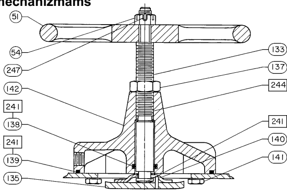
11 pav. Viršuje montuojamas rankinio valdymo blokas, skirtas 30/30i - 60/60i dydžio pavarus mechanizmams
