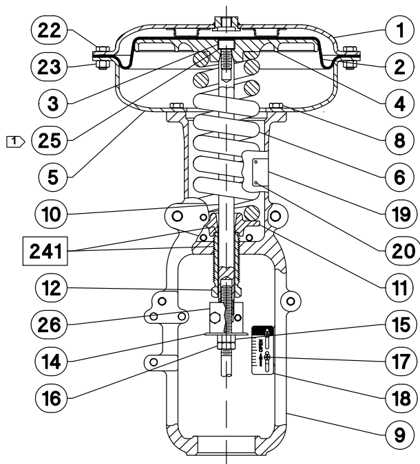
Ilustracja 7. Siłowniki Fisher 657 o wielkości od 30i do 60i
