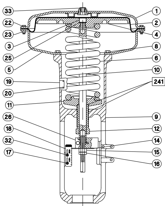
Ilustracja 9. Siłownik Fisher 657 o wielkości 70i
