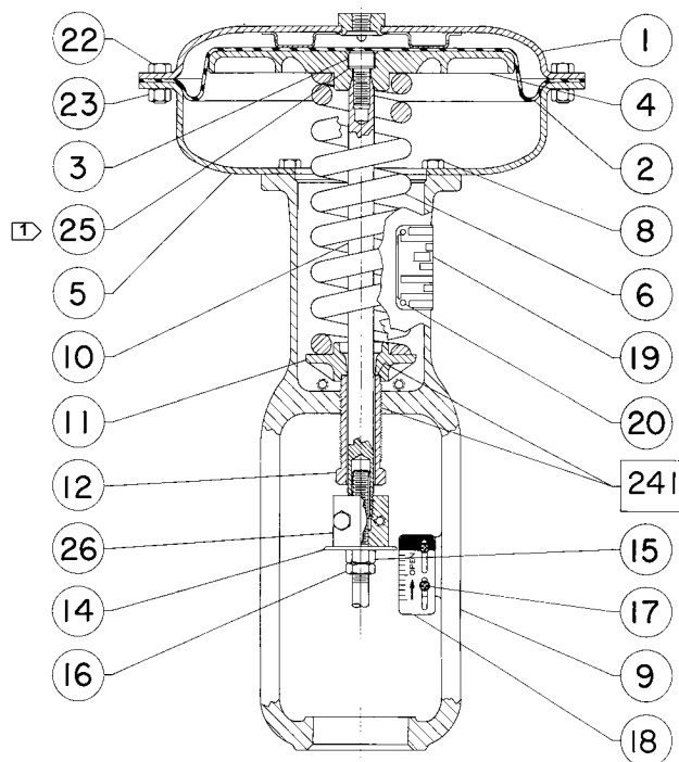
Ilustracja 6. Siłowniki Fisher 657 o wielkości od 30 do 60
