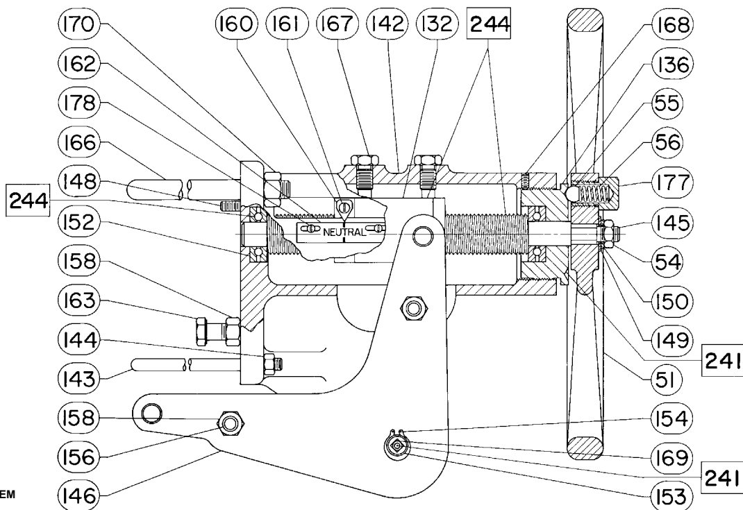
Ilustracja 15. Zespół napędu ręcznego montowany z boku na siłownikach o wielkości 45, 46, 50 i 60
