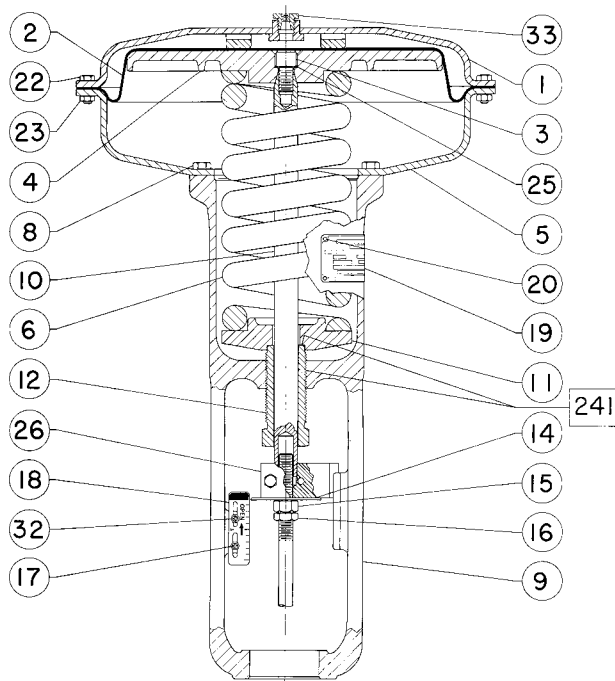
Ilustracja 8. Siłownik Fisher 657 o wielkości 70
