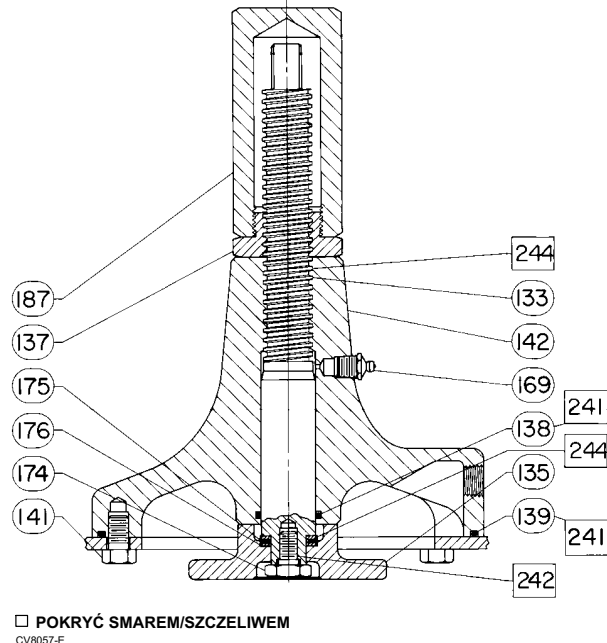
Ilustracja 19. Regulowany ogranicznik ruchu w górę montowany w obudowie do siłowników o wielkości 70/70i i 87 (styl 1)
