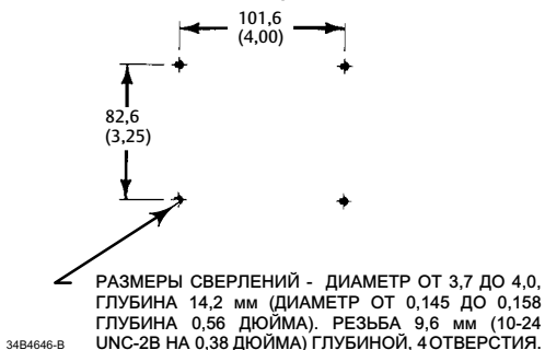
СХЕМА ВЫСВЕРЛИВАНИЯ ОТВЕРСТИЙ И НАРЕЗАНИЯ ВНУТРЕННЕЙ РЕЗЬБЫ НА ПЛИТЕ ДЛЯ ПРИВОДОВ РАЗМЕРОВ 30, 40, 60 И 68
