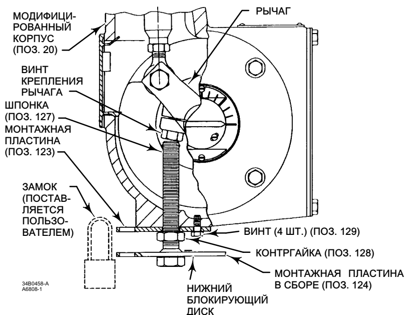
Рис. 5. Механизм блокирования (для приводов размеров 30, 40, 60 и 68)
