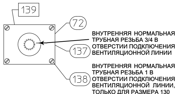
СХЕМА СВЕРЛЕНИЙ И ВНУТРЕННЕЙ РЕЗЬБЫ НА ПЛИТЕ ДЛЯ ПРИВОДОВ РАЗМЕРОВ 80 И 100
