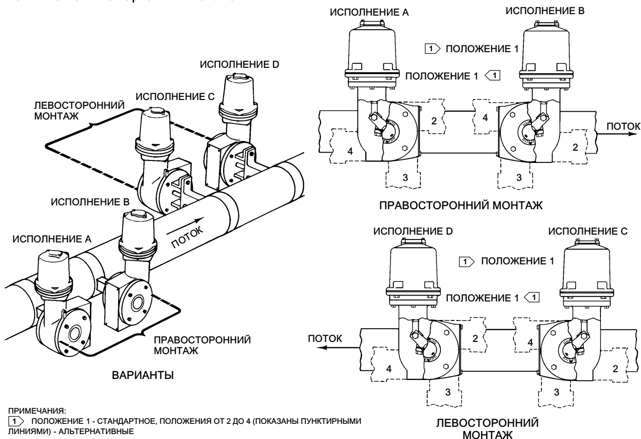
Рис. 2. Монтажные варианты и положения
