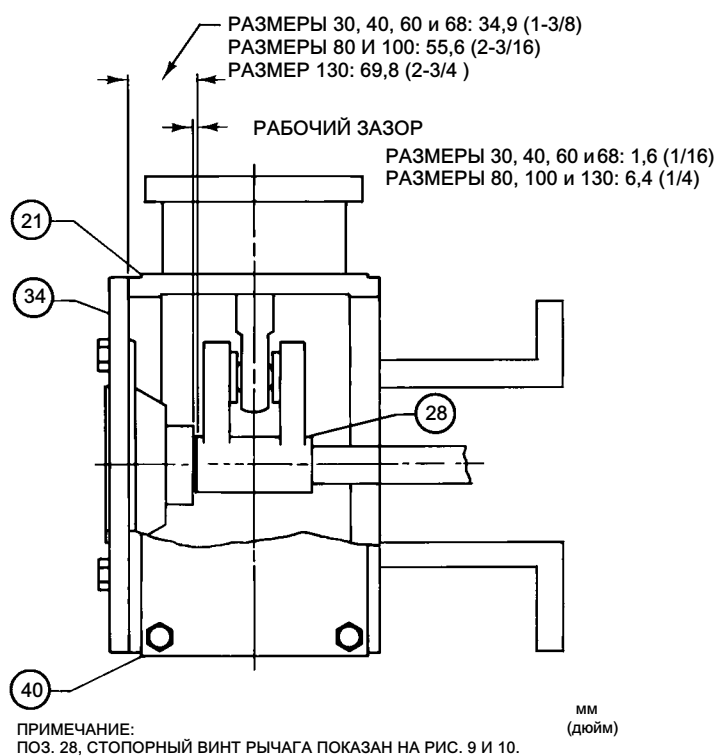
Рис. 3. Рабочий зазор рычага
