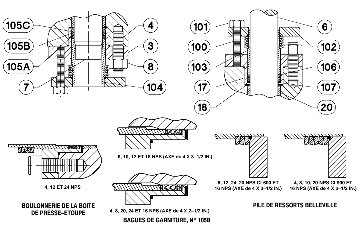
Figure 13. Garniture à faible émission fugitive
