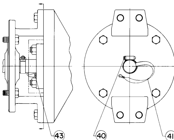
Figure 3. Tresse de conductivité axe-corps en option
