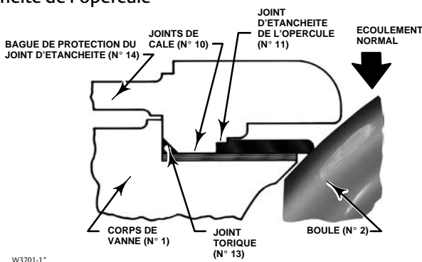
Figure 4. Détail du joint d'étanchéité de l'opercule
