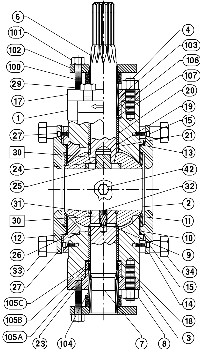
Figure 11. Vanne Fisher V250 à construction à joint double
