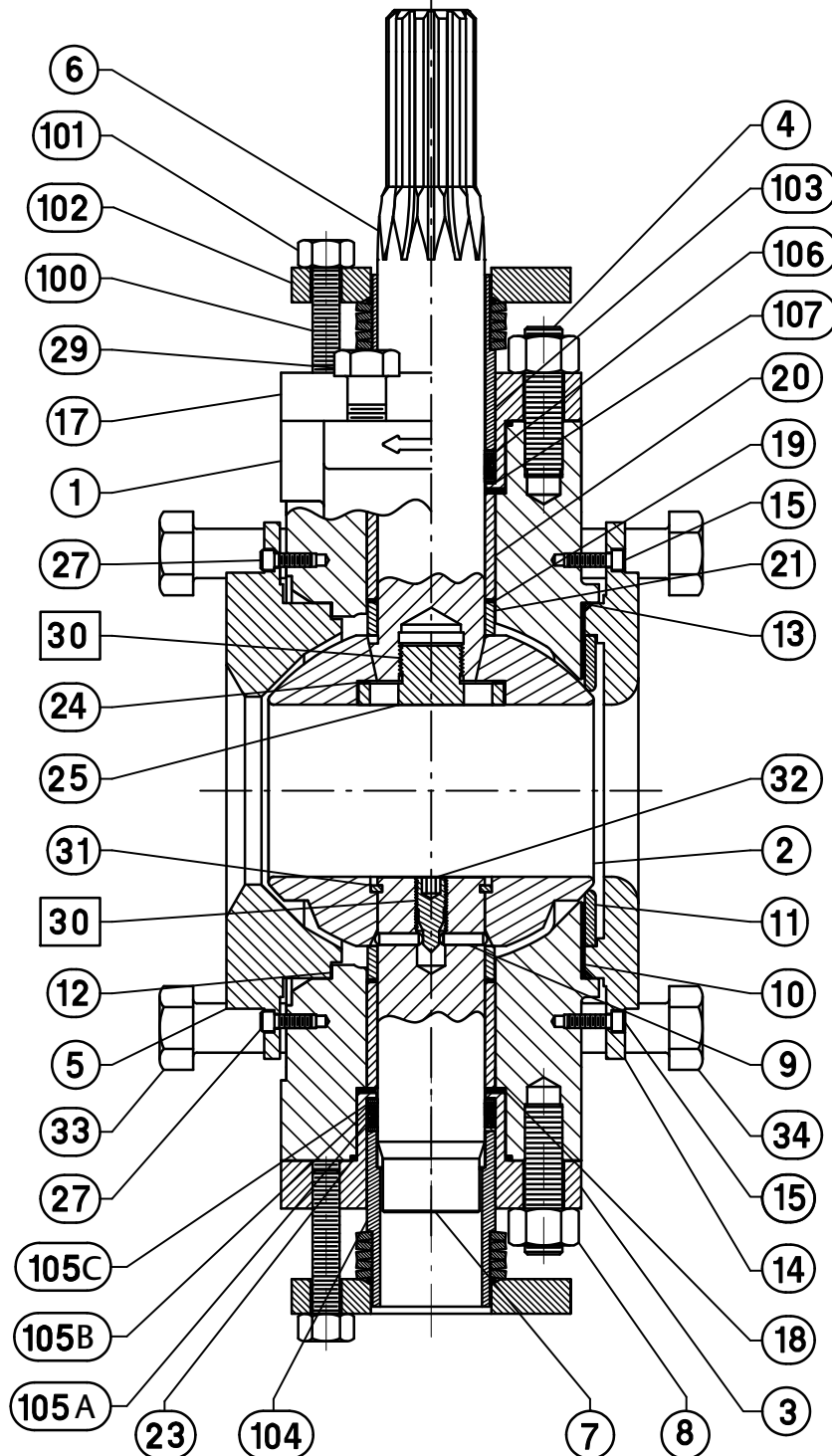
Figure 12. Vanne Fisher V250 à construction à joint simple
