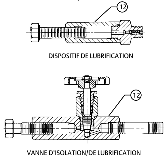
Figure 2. Dispositif de lubrification et vanne d'isolation/de lubrification
