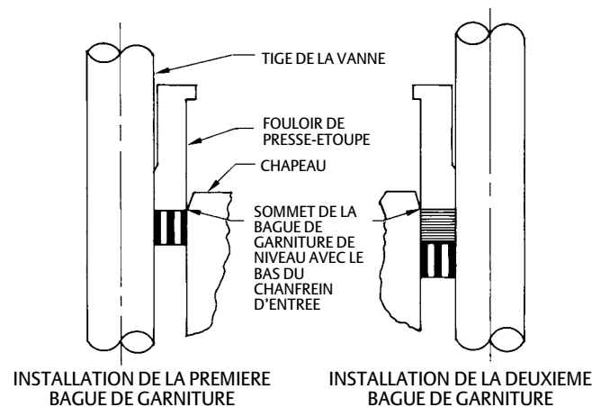
Figure 5. Installation des bagues de garniture en ruban / filament de graphite, une à la fois
