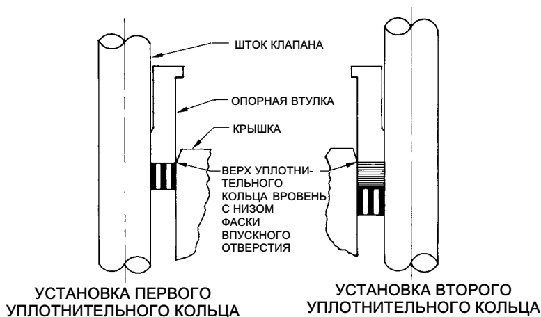
Рис. 5. Поочередная установка уплотнительных колец из графитовой ленты / нити
