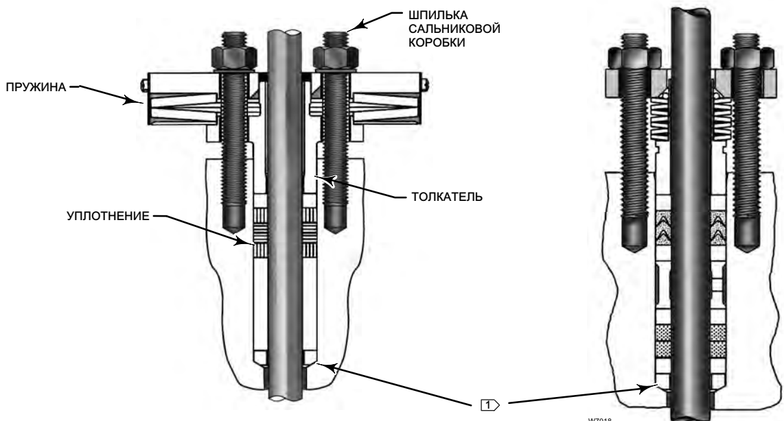
ТИПОВАЯ СИСТЕМА УПЛОТНЕНИЯ HIGH-SEAL С УПЛОТНЕНИЕМ ИЗ ГРАФИТА ULF
