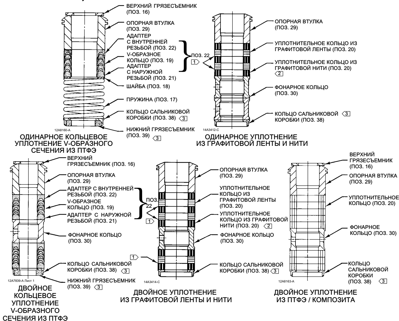
Рис. 3. Сальниковые уплотнения
