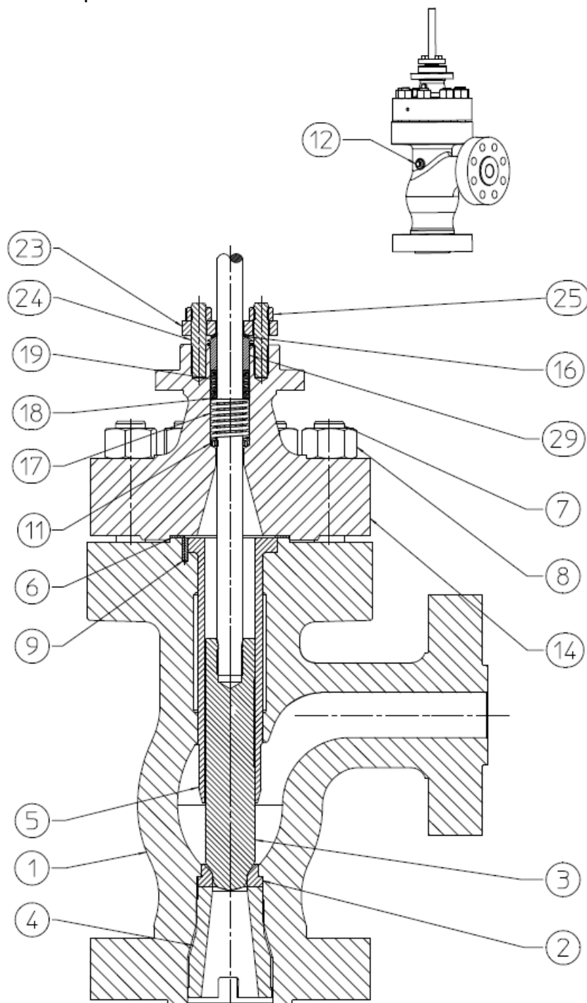
Рис. 6. Клапан Fisher 461 в сборе
