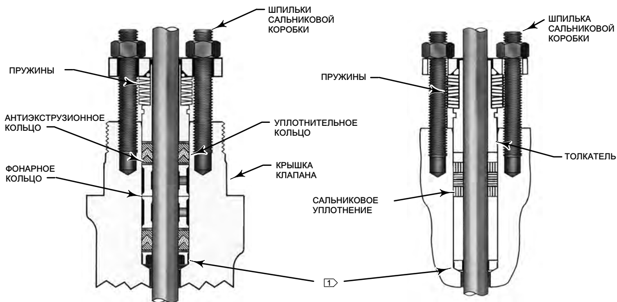
ТИПОВАЯ СИСТЕМА УПЛОТНЕНИЯ ENVIRO-SEAL С УПЛОТНЕНИЕМ ИЗ ПТФЭ
