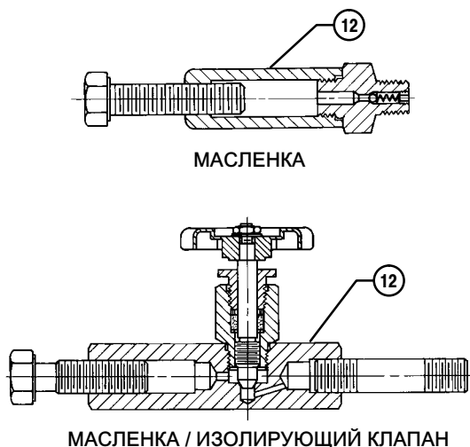
Рис. 2. Масленка и масленка / изолирующий клапан
