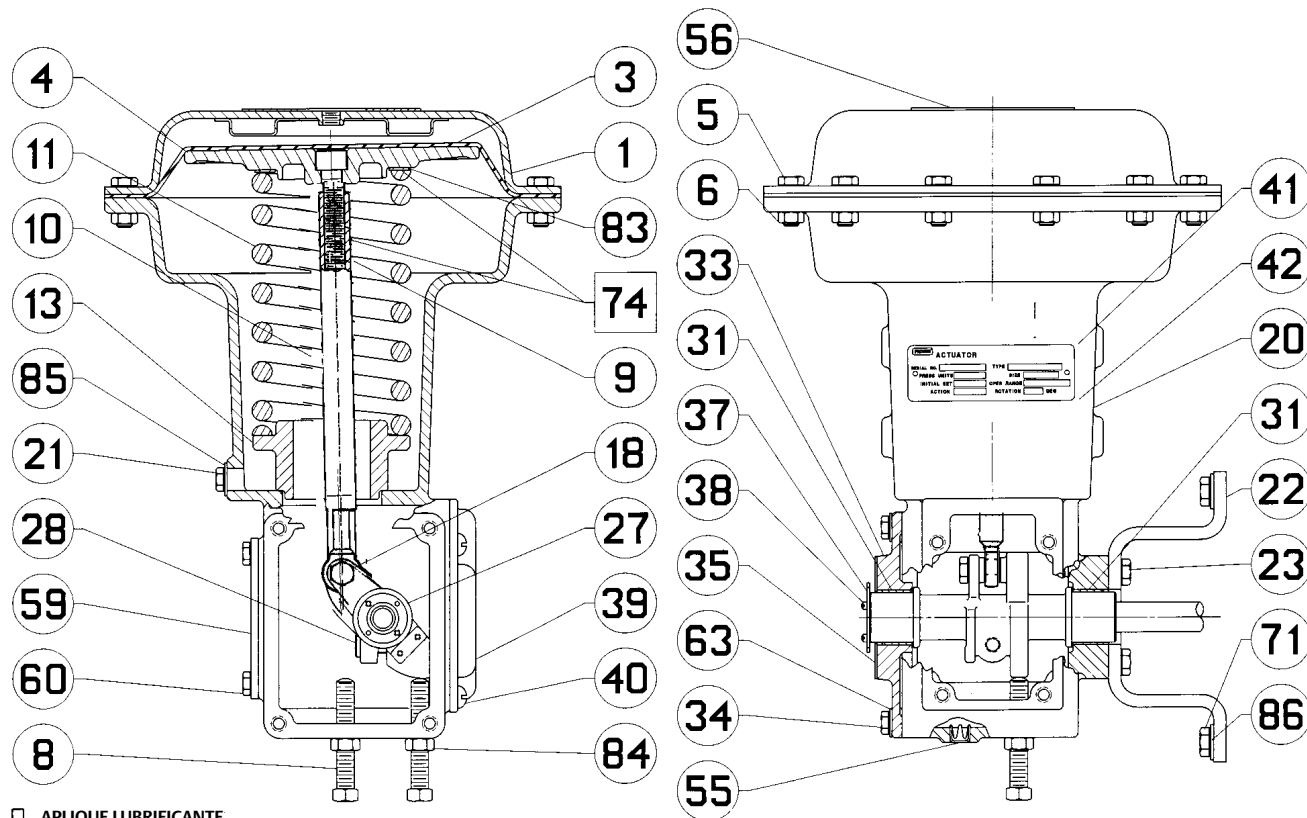
Figura 9. Actuador 1051 Tamanho 33 da Fisher com Adaptação de Montagem F ou G
