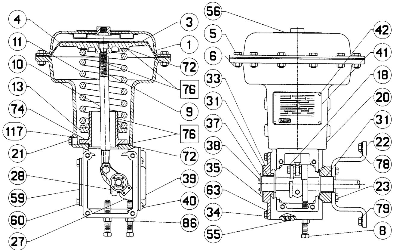
Figura 10. Actuador 1052 Tamanho 33 da Fisher com Adaptação de Montagem F ou G
