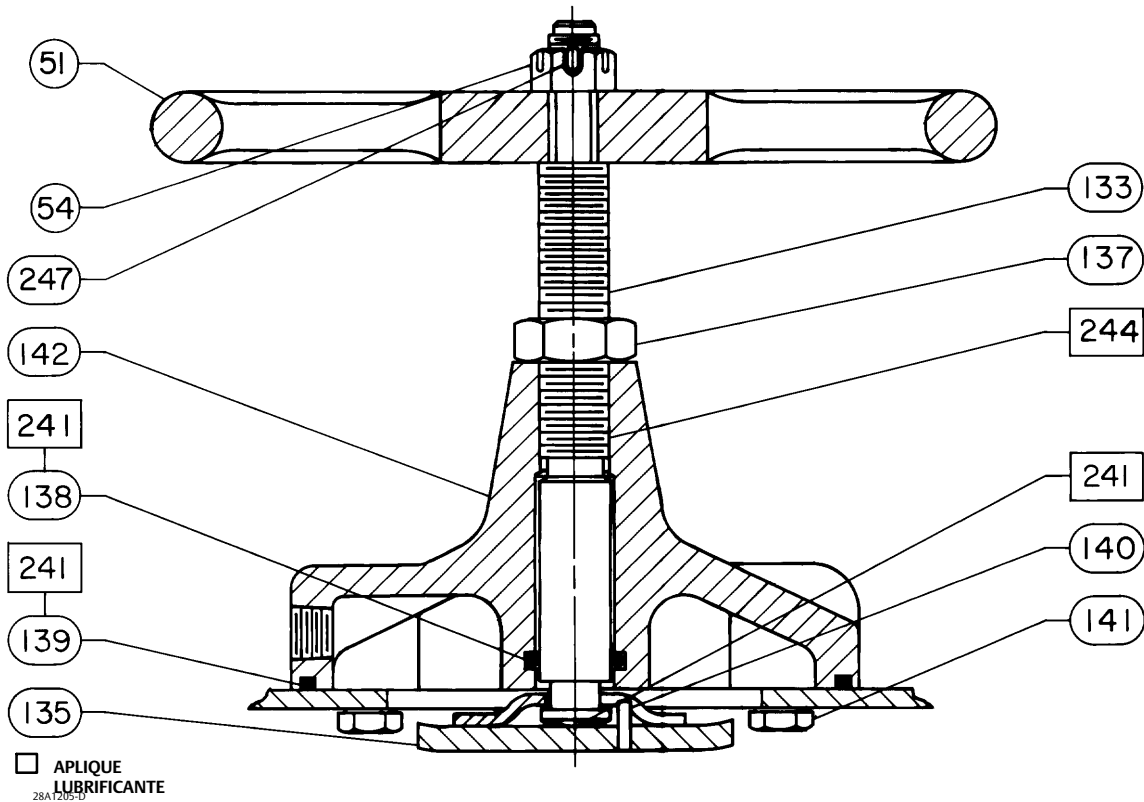
Figura 17. Conjunto do Volante Montado no Topo
