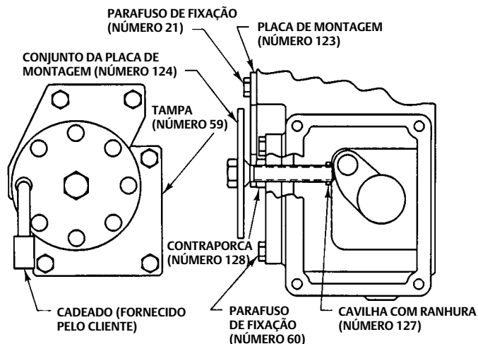
Figura 8. Mecanismo de Bloqueio do Actuador 1051 e 1052 da Fisher
