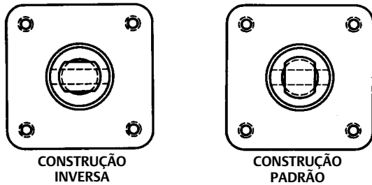
Figura 12. Construções Padrão e Inversa da Manga de Eixo Usadas para as Adaptações de Montagem H
