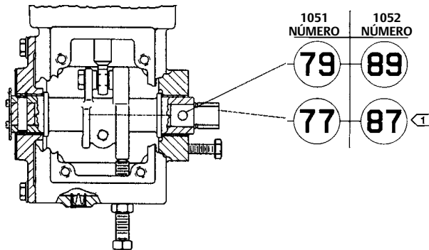
Figura 11. Peças Usadas para a Adaptação de Montagem H
