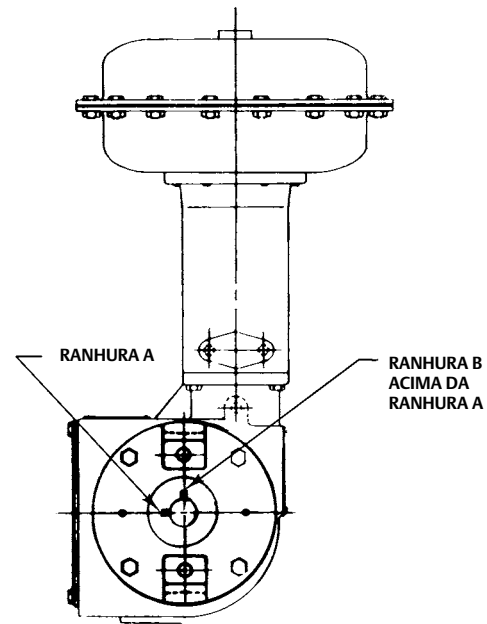
ORIENTAÇÃO DO ACOPLAMENTO DE REFERÊNCIA PARA O QUADRO 5
