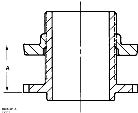
Figura 6. Dimensões Predefinidas da Sede da Mola para o Actuador 1052 Tamanho 33 da Fisher
