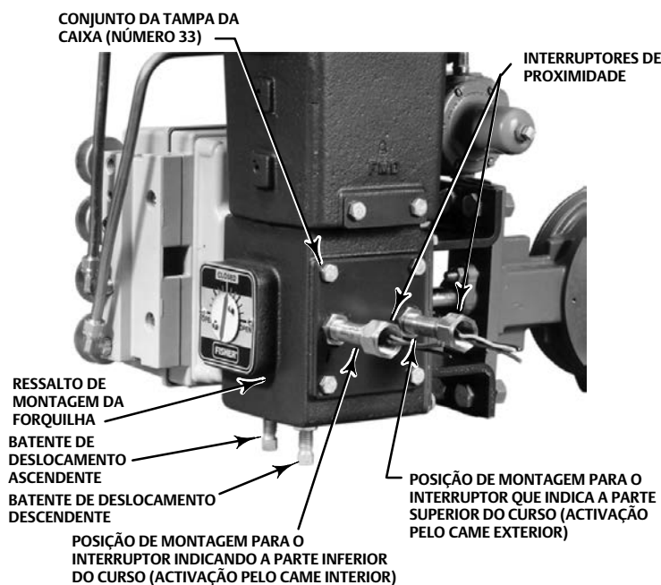
Figura 3. Batentes de Deslocamento e Posições dos Interruptores no Actuador 1051 e 1052 Tamanho 33 da Fisher
