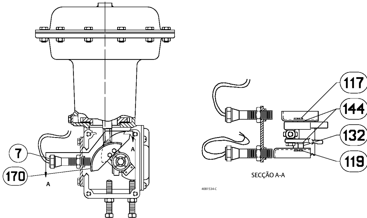
Figura 15. Montagem do Interruptor de Proximidade no Actuador 1051 e 1052 Tamanho 33 da Fisher
