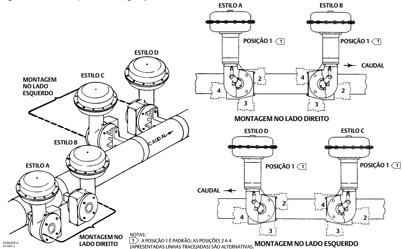
Figura 2. Estilos e Posições de Montagem para Actuadores 1051 e 1052 da Fisher
