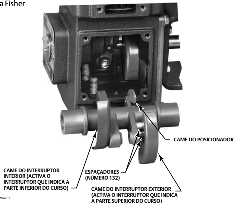
Figura 7. Orientação dos Cames do Interruptor e do Posicionador na Alavanca do Actuador 1051 e 1052 Tamanho 33 da Fisher
