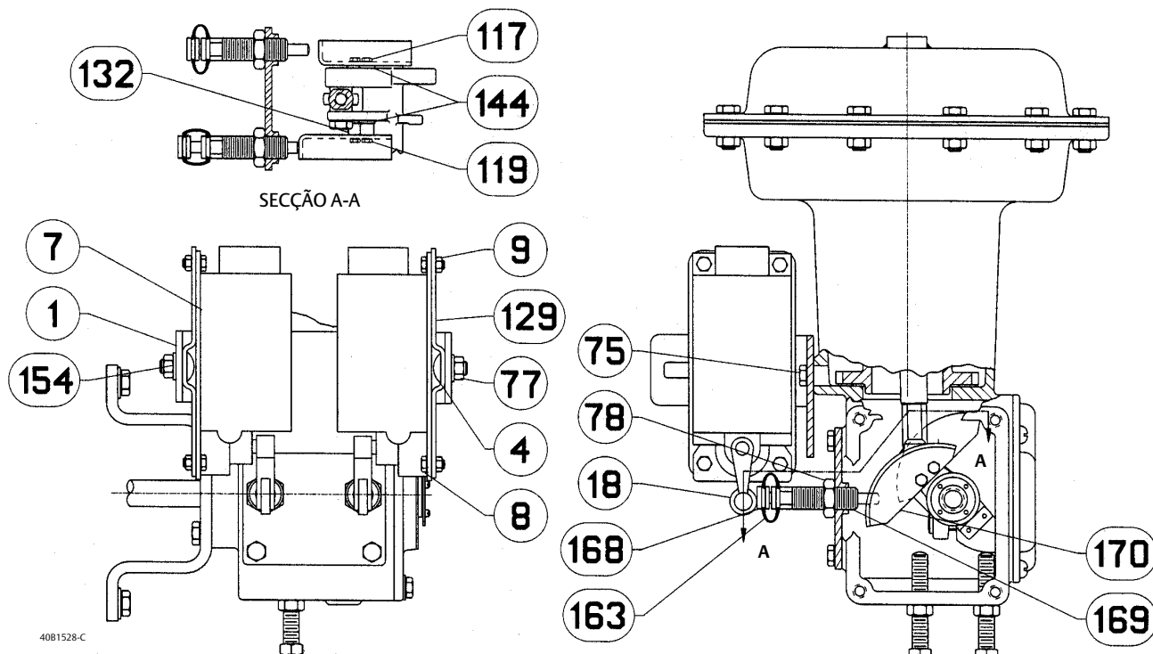
Figura 16. Conjunto de Interruptor Operado por Alavanca Típico
