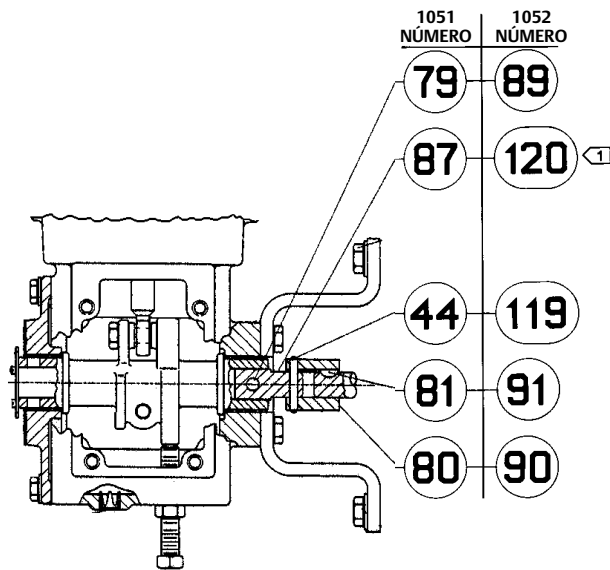
Figura 13. Peças Usadas para a Adaptação de Montagem J
