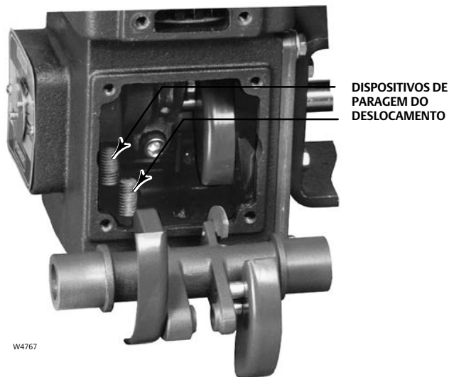
Figura 5. Ajuste da mola
