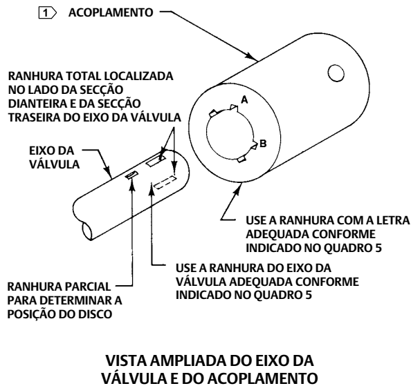
Figura 4. Acoplamento do Eixo da Válvula para a Adaptação de Montagem J
