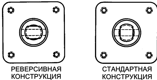
Рис. 12. Стандартная и реверсивная конструкции короткого вала, используемые для крепления типа Н
