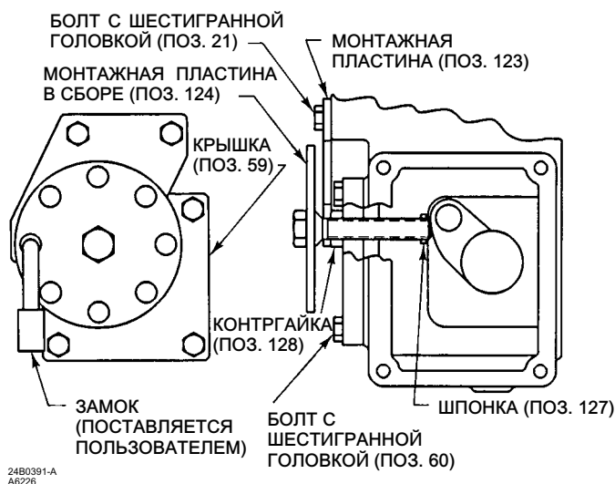
Рис. 8. Блокировочное устройство для приводов Fisher моделей 1051 и 1052
