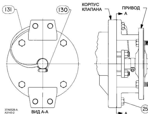
Рис. 3. Шина заземления вала к корпусу клапана (доп.)
