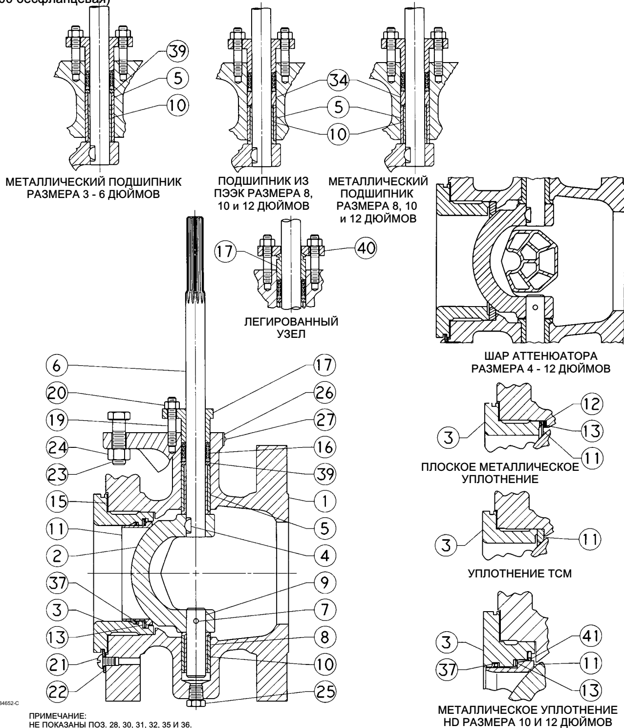
Рис. 32. Узел клапана Fisher конструкции V150 и V300 серии, отличной от В (размер от 3 до 12 дюймов) (детали типичны для конструкции V200, за исключением того, что конструкция V200 бесфланцевая)
