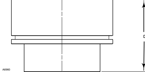
КЛАПАН ТИПА ТОРЕЦ К ТОРЦУ CL150 ANSI B16.10 (УКОРОЧЕННЫЙ)
