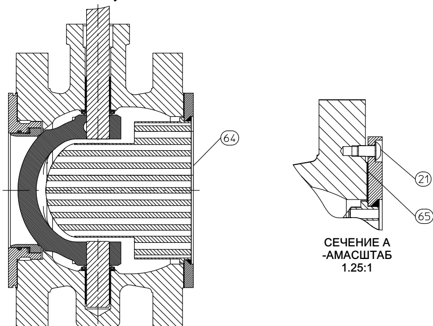
Рис. 29. Вид клапана Fisher V300 с узлом Cavitrol Hex
