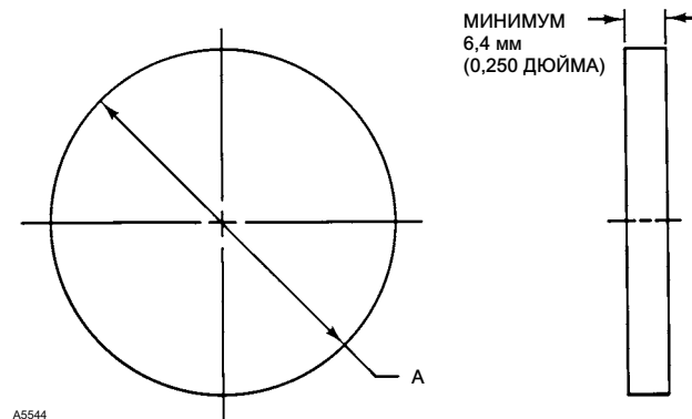
Рис. 12. Размеры пластины для съёма уплотнения HD
