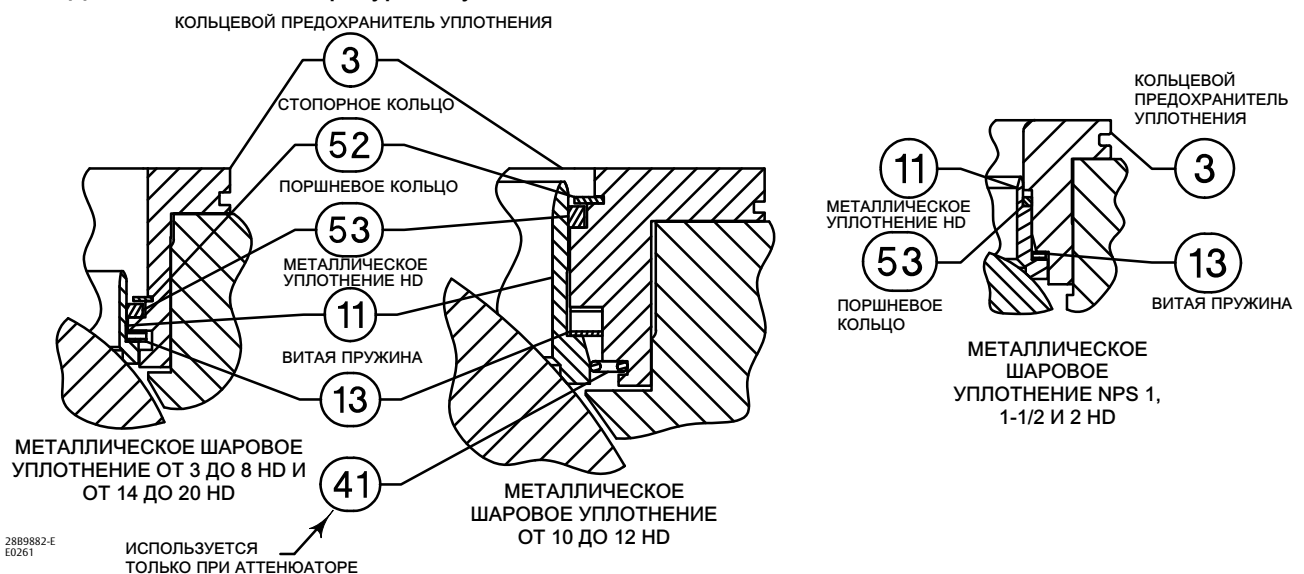
Рис. 10. Детали высокотемпературного уплотнения HD
