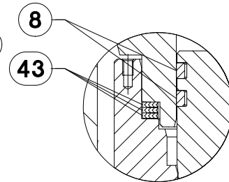
DETTAGLIO A SOLO ANELLO DEL PISTONE
