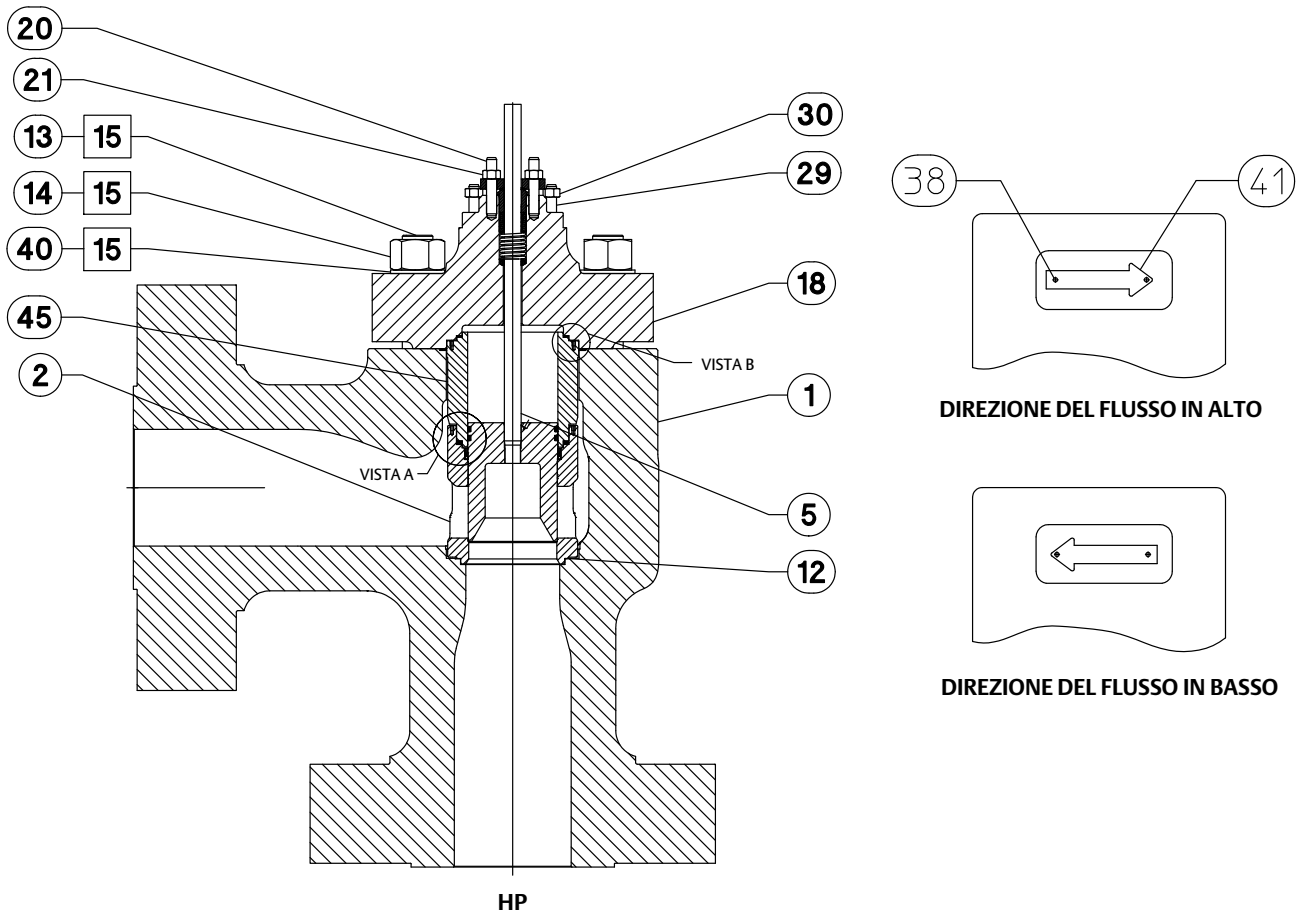
Figura 38. Valvola HPAD e HPAT da 12 pollici
