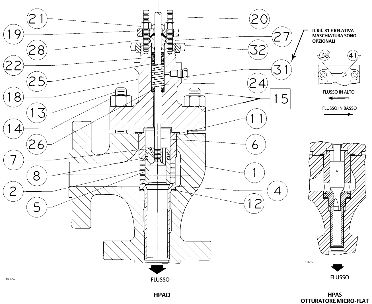
Figura 23. Valvola HPAD da 2 pollici
