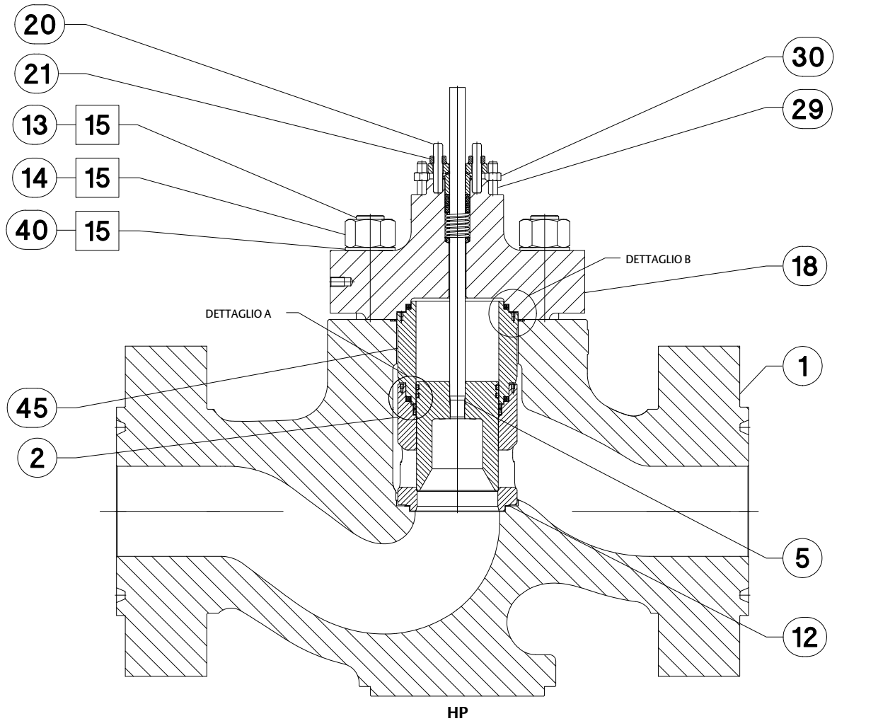
Figura 32. Valvola HPD e HPT da 16 a 24 pollici
