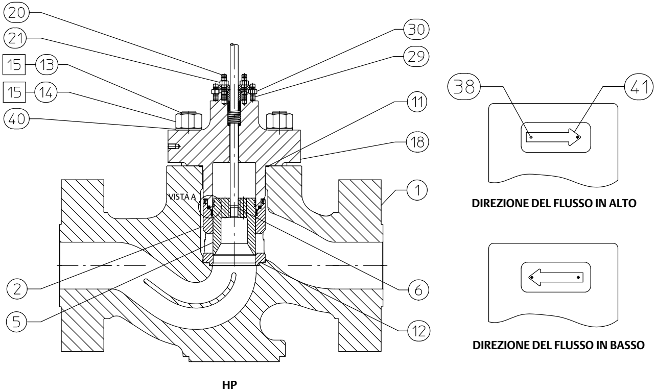
Figura 26. Valvola HPD e HPT da 8 a 12 pollici con cappello bordato
