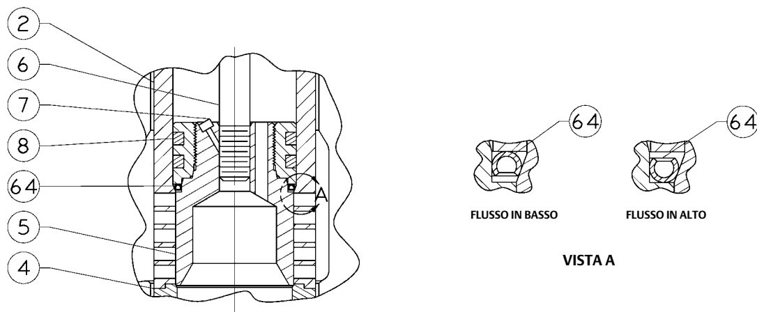
Figura 13. HPD con trim C-seal
