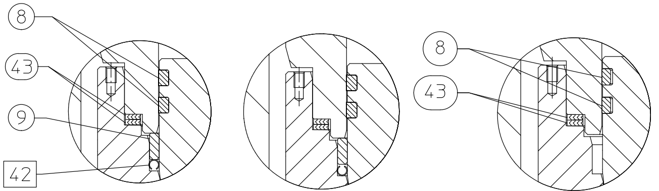
VISTA A TENUTA BORE SEAL, FLUSSO IN BASSO
