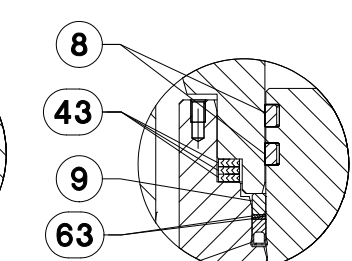
DETTAGLIO A TENUTA HTS1, FLUSSO IN BASSO
