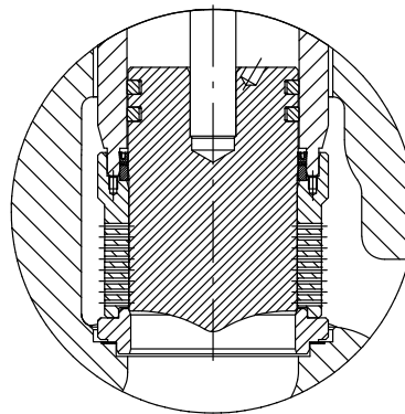
WHISPER III CON OTTURATORE TRAFILATO, UTILIZZARE SOLO PER CL900/CL1500
