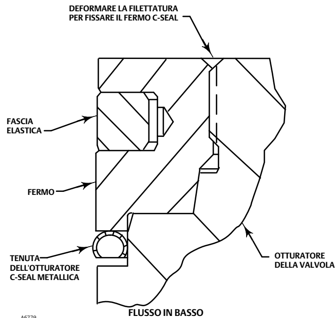
Figura 16. Piegatura delle filettature del fermo C-seal
