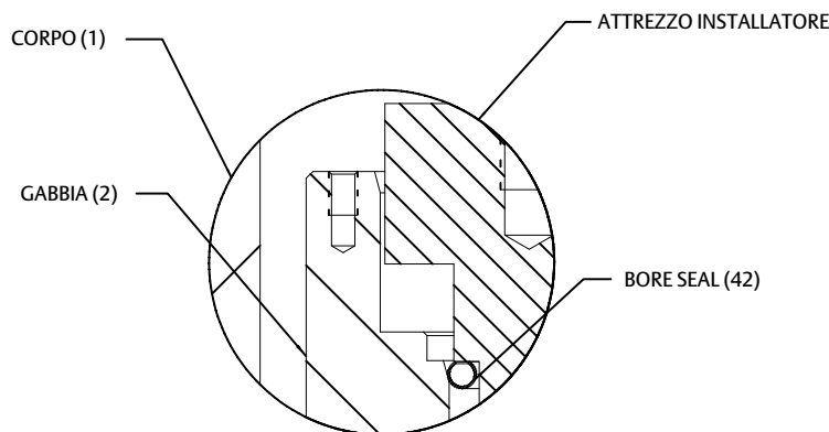
Figura 20. Installazione della tenuta Bore Seal con attrezzo
