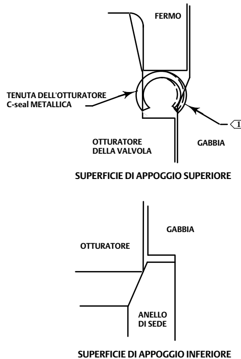
Figura 17. Superfici di appoggio inferiore (otturatore della valvola-anello di sede) e superiore (tenuta dell'otturatore C-seal-gabbia)
