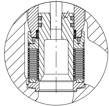
CAVITROL III A 2 STADI
