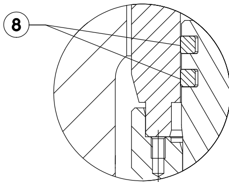
VISTA A HPD, SOLO FASCIA ELASTICA
