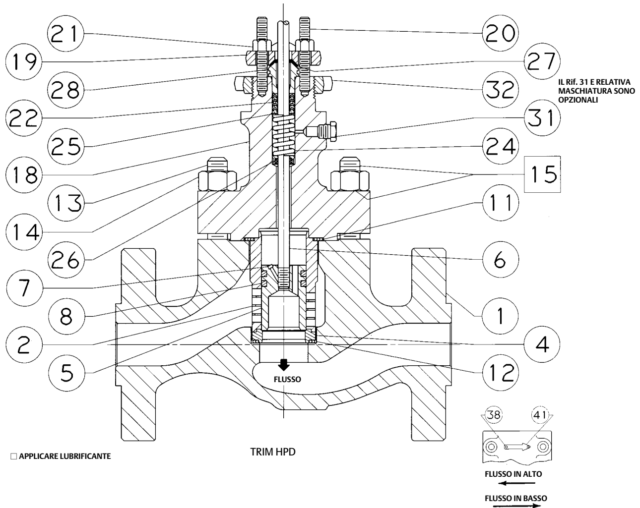
Figura 24. HPD da 2 a 6 pollici (lungo) Valvola
