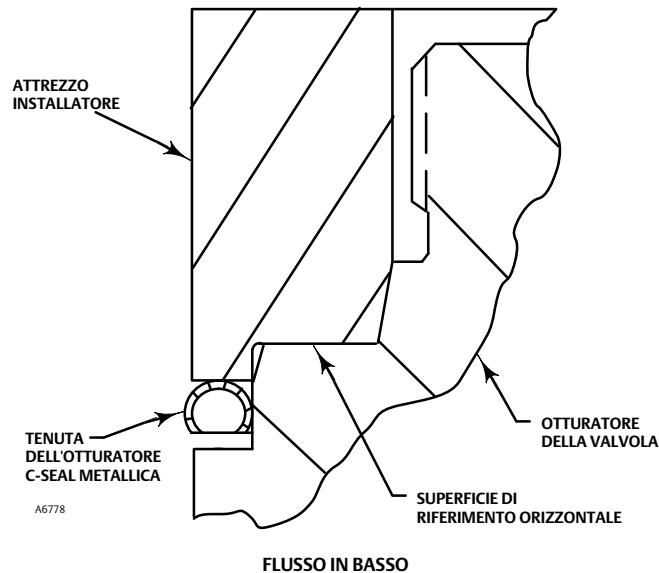
Figura 15. Installazione della tenuta dell'otturatore C-seal con l'attrezzo installatore
