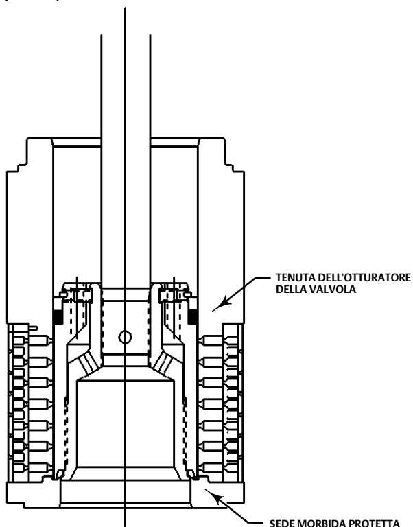
Figura 10. Tipico gruppo trim TSO bilanciato, design con passaggio di grandi dimensioni (diametri di passaggio di 2,6875 pollici e superiori)
