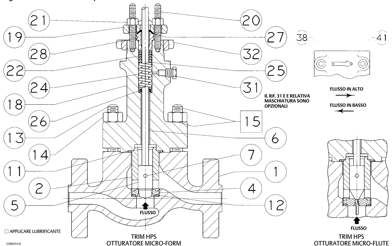
Figura 22. Valvola HPS da 1 pollice
