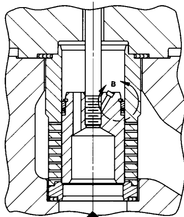
Figura 25. HP da 2 a 6 pollici (lungo) valvola - Configurazioni alternative (continua)
