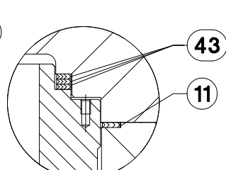
DETTAGLIO B
