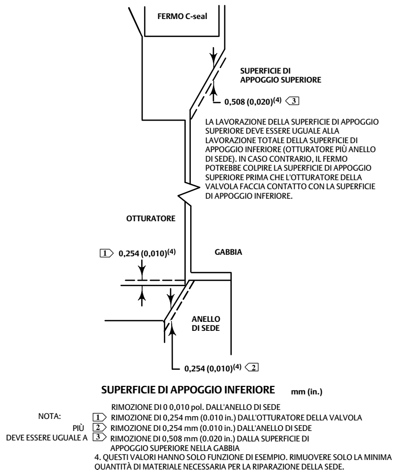
Figura 18. Esempio di lavorazione delle superfici di appoggio inferiore (otturatore della valvola-anello di sede) e superiore (tenuta dell'otturatore C-seal-gabbia)
