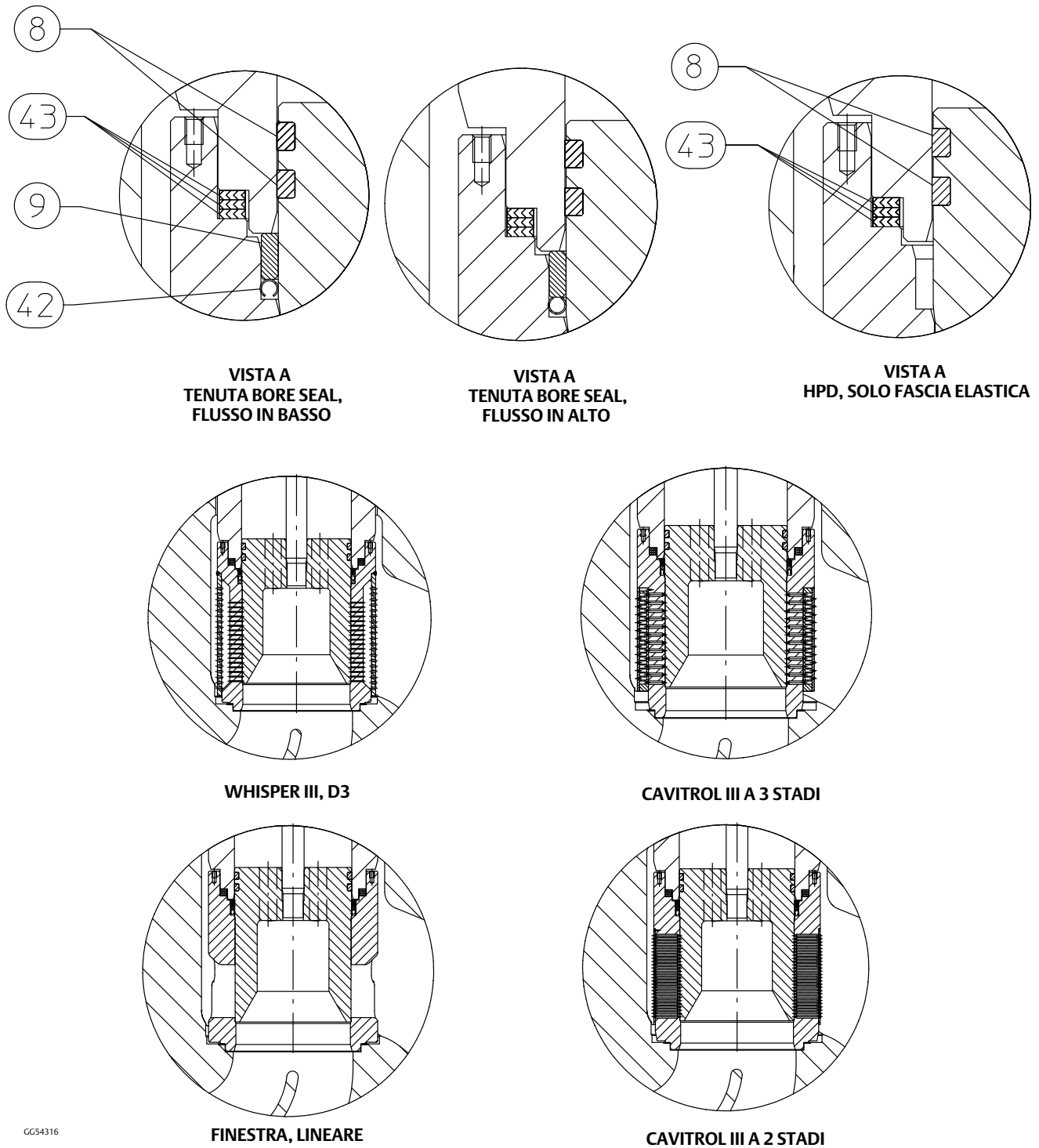
Figura 27. Valvola HPD e HPT da 8 a 12 pollici con cappello bordato - Configurazioni alternative
