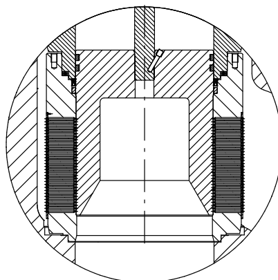
CAVITROL III A 2 STADI
