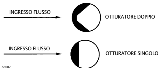
Figura 11. Orientamento otturatore valvola Micro-Flat
