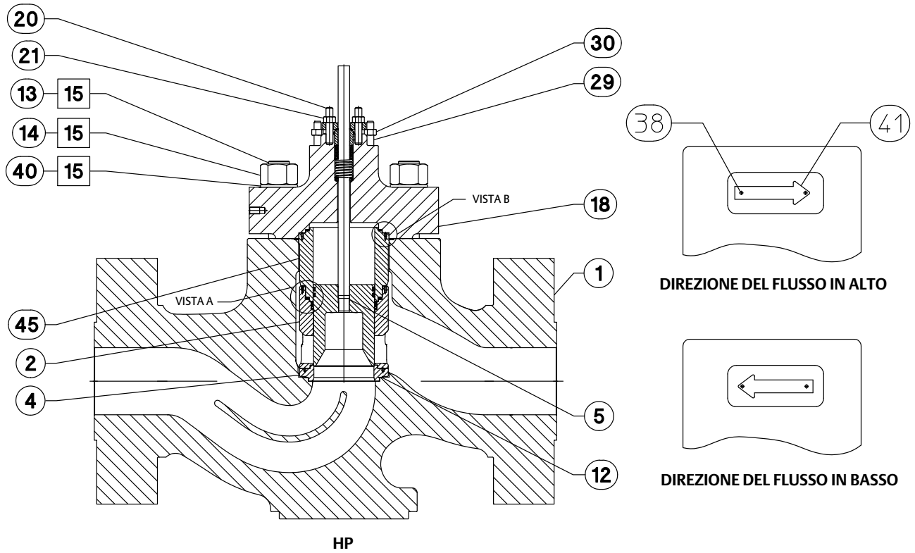
Figura 28. Valvola HPD e HPT da 8 a 12 pollici con fermo della gabbia
