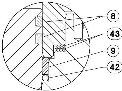
VISTA A TENUTA BORE SEAL, FLUSSO IN BASSO
