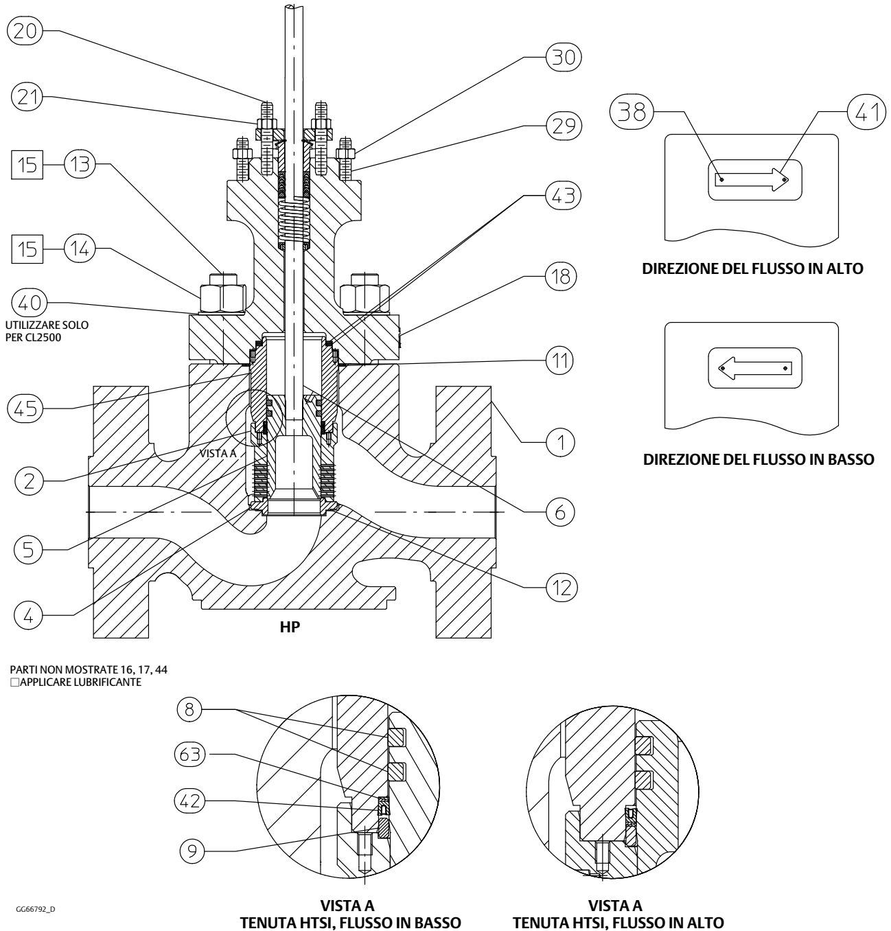
Figura 34. Valvola HPD (corto), HPT (corto) e HPS (corto) da 3 a 6 pollici
