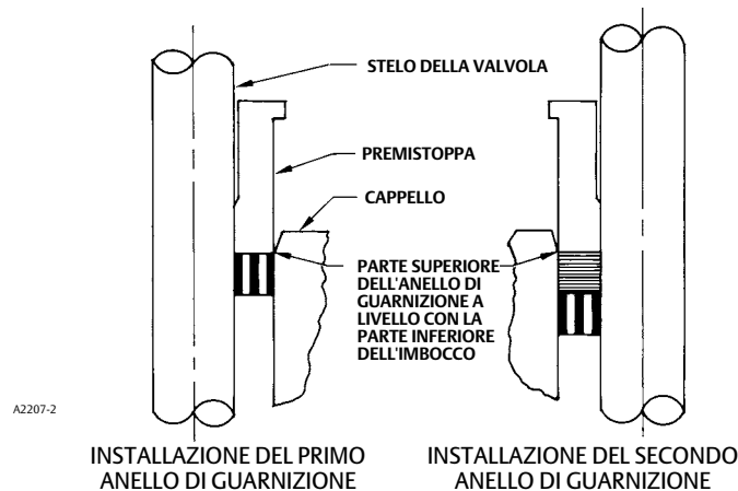
Figura 5. Installazione delle baderne a nastro e a filo di grafite una alla volta
