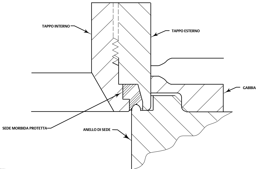
Figura 7. Dettaglio della sede morbida protetta
