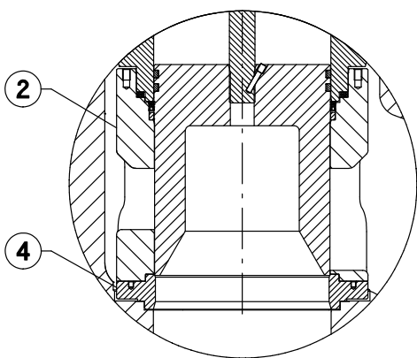
FINESTRA, LINEARE
