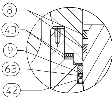
VISTA A TENUTA HTSI, FLUSSO IN BASSO
