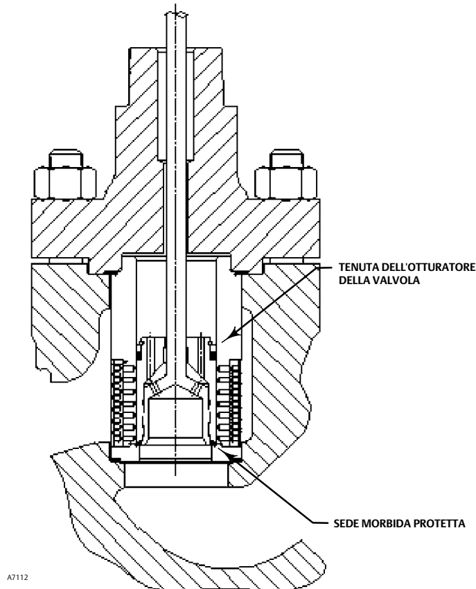
Figura 9. Tipico Trim TSO bilanciato (diametro di passaggio di 1,6875 pollici)
