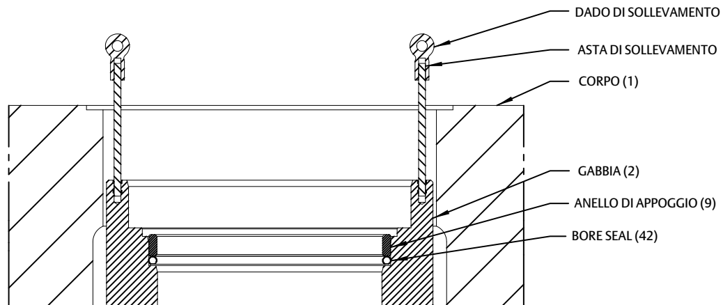
Figura 6. Rimozione della gabbia con asta di sollevamento e dado
