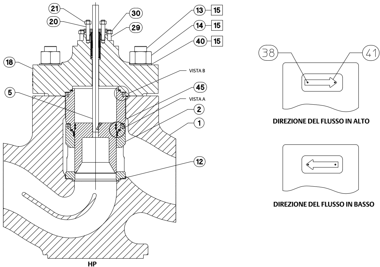
Figura 30. Valvola HPD e HPT da 14 pollici
