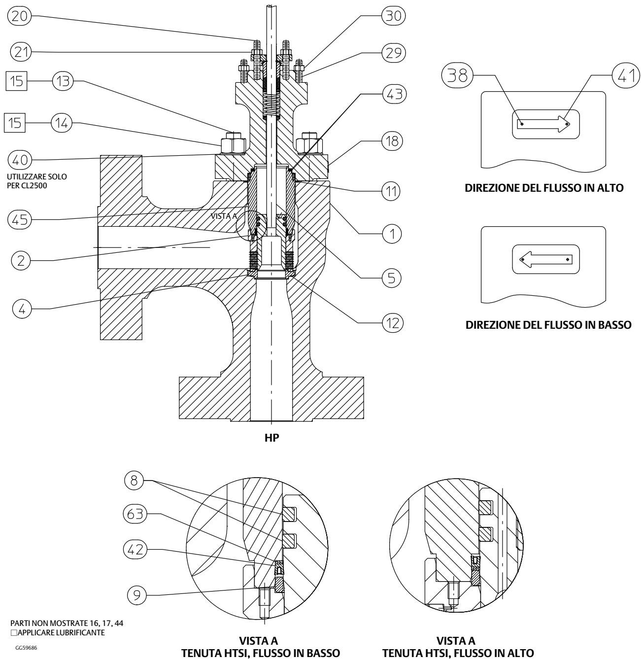
Figura 36. Valvola HPAD e HPAT da 6 e 8 pollici
