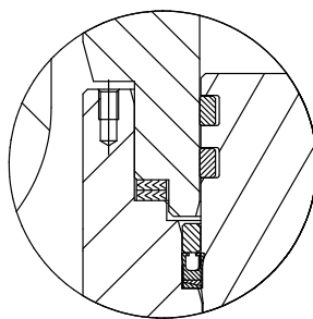
VISTA A TENUTA HTSI, FLUSSO IN ALTO
