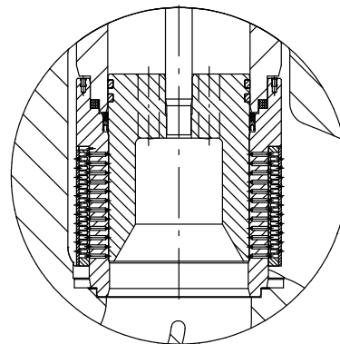
CAVITROL III A 3 STADI
