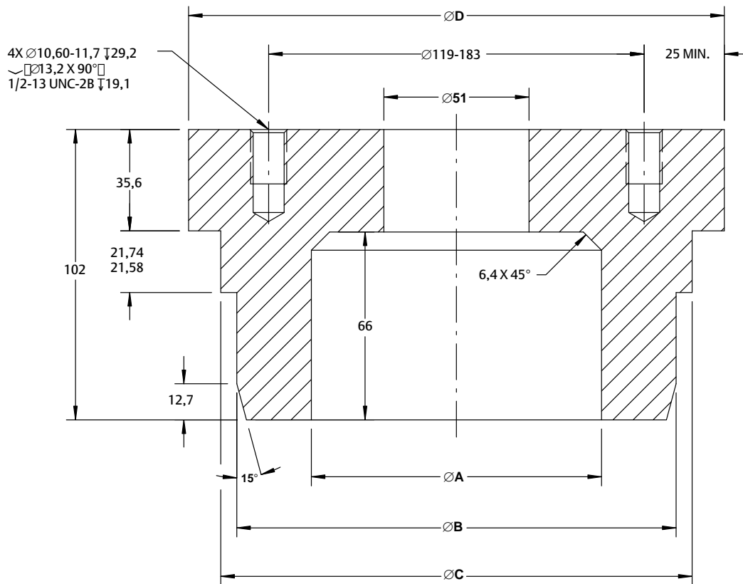
Figura 21. Attrezzo installatore della tenuta Bore Seal
