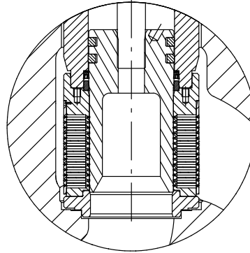
CAVITROL III A 2 STADI
