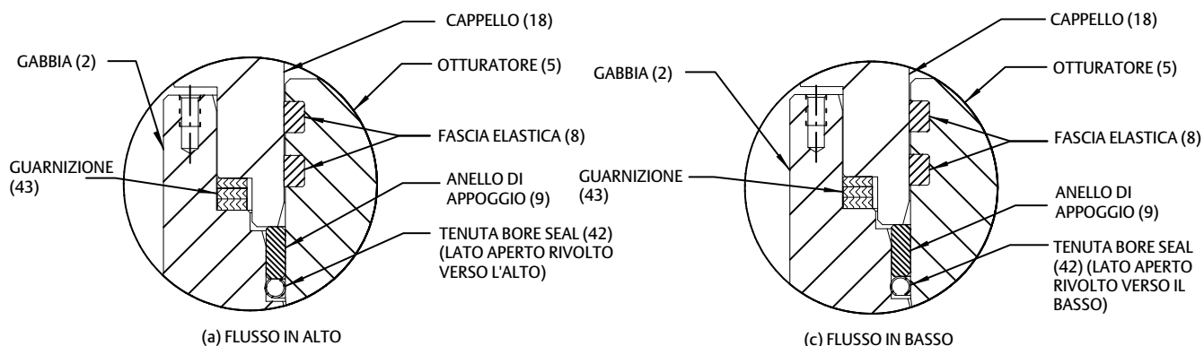
Figura 19. Orientamento di installazione della tenuta Bore Seal
