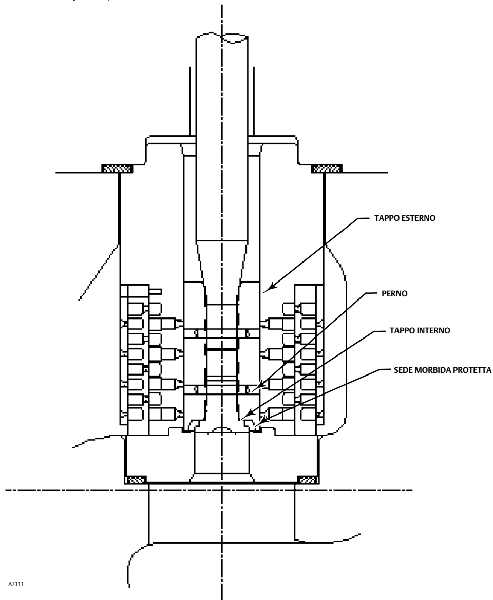
Figura 8. Tipico gruppo trim TSO non bilanciato, design con passaggio ridotto (diametro di passaggio di 0,8125 pollici)
