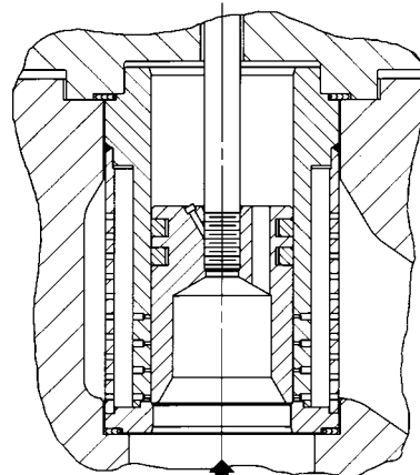
Figura 25. HP da 2 a 6 pollici (lungo) valvola - Configurazioni alternative (continua)
