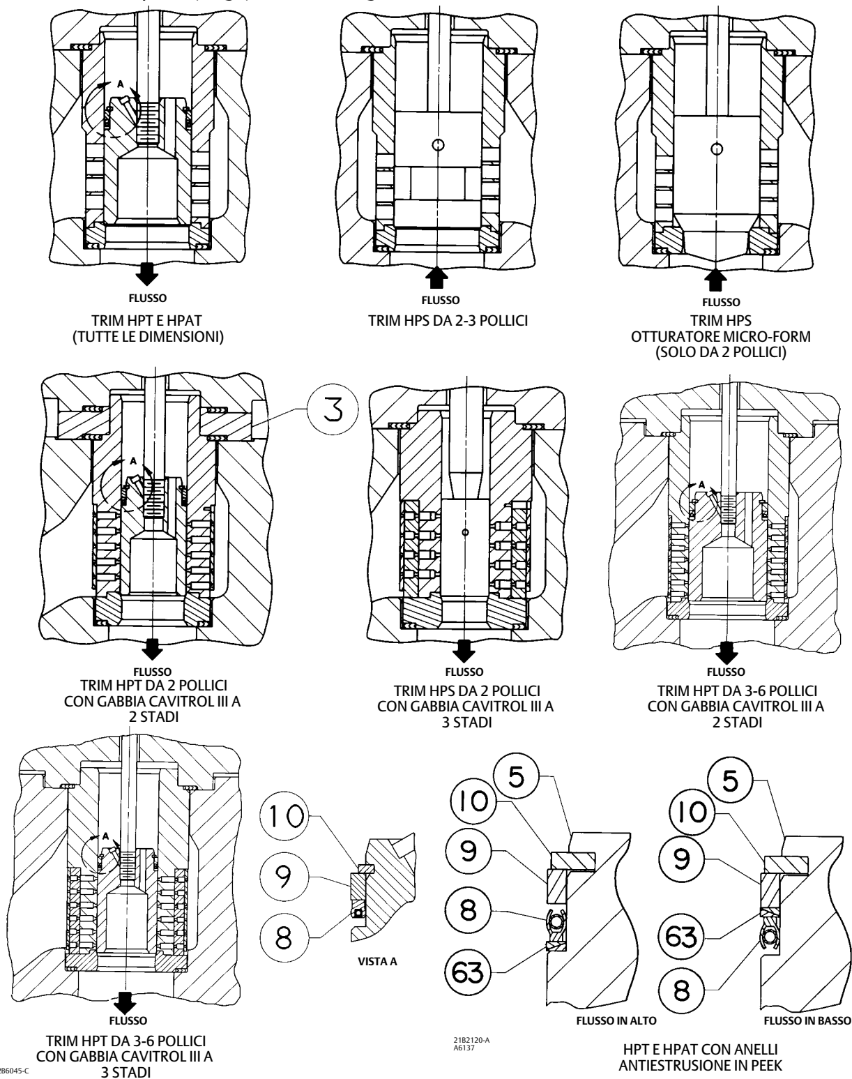
Figura 25. HP da 2 a 6 pollici (lunga) valvola - Configurazioni alternative
