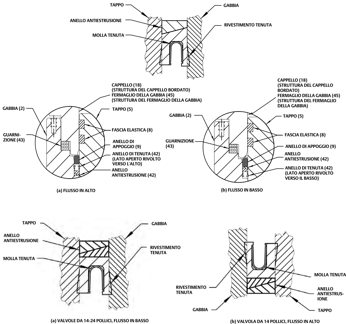
Figura 12. Dettaglio della sede morbida e orientamento di installazione
