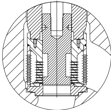
WHISPER III, D3 HPS OPZIONE OTTURATORE NON BILANCIATO
