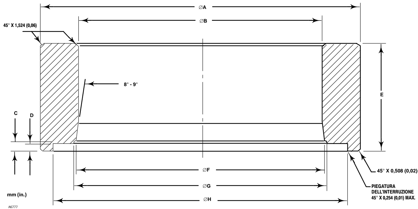
Figura 14. Attrezzo installatore per la tenuta dell'otturatore C-seal
