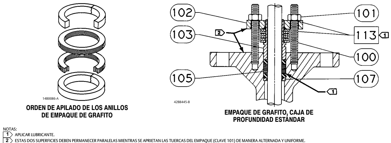
Figura 14. Arreglos de empaque rotativo ENVIRO-SEAL típicos con empaque de grafito
