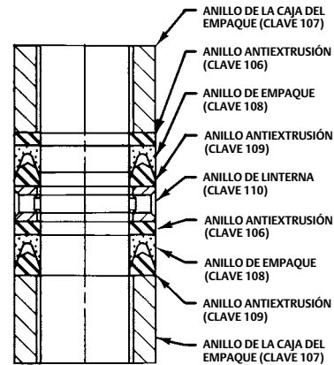
EMPAQUE DE PTFE DOBLE CON TUBERÍA PARA FUGAS Y UNA CAJA DE EMPAQUE PROFUNDO
