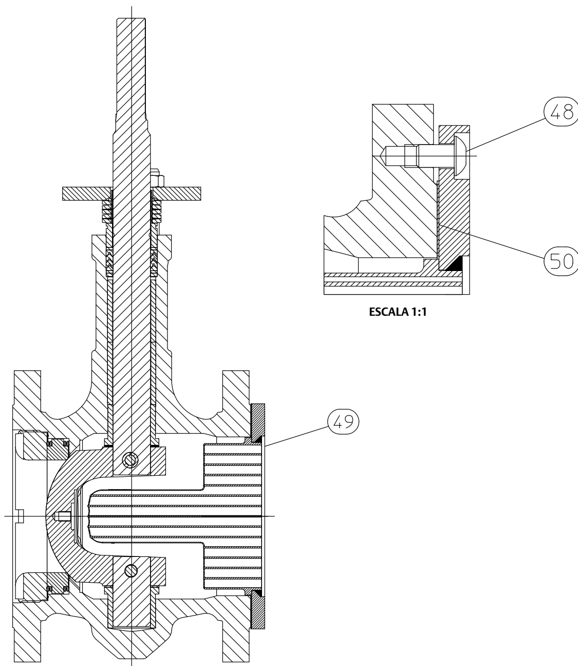
Figura 16. Conjunto de la válvula Fisher CV500 con Cavitrol hexagonal
