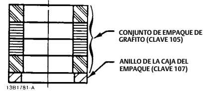
EMPAQUE DE GRAFITO EN UNA CAJA DE PROFUNDIDAD ESTÁNDAR
