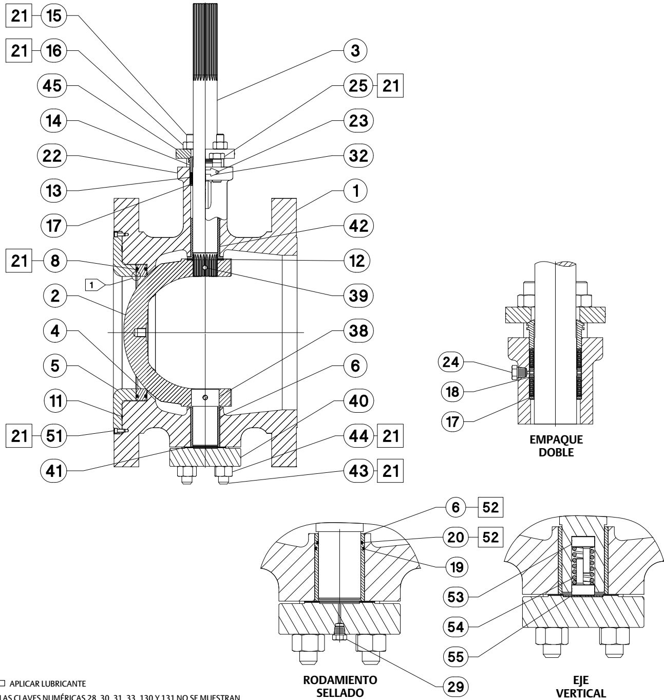
Figura 12. Válvula Fisher CV500, NPS 14 al 20
