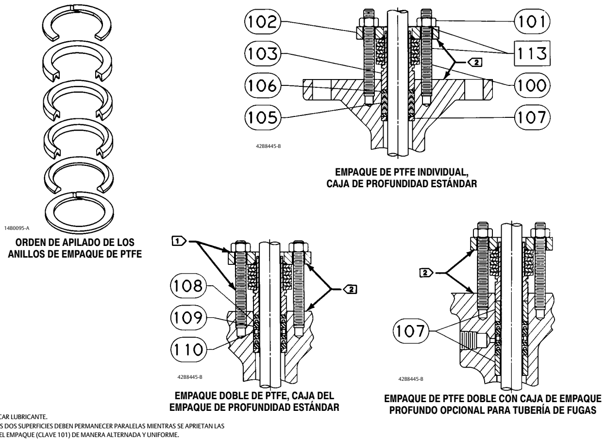
Figura 13. Arreglos de empaque rotativo ENVIRO-SEAL típicos con empaque de PTFE
