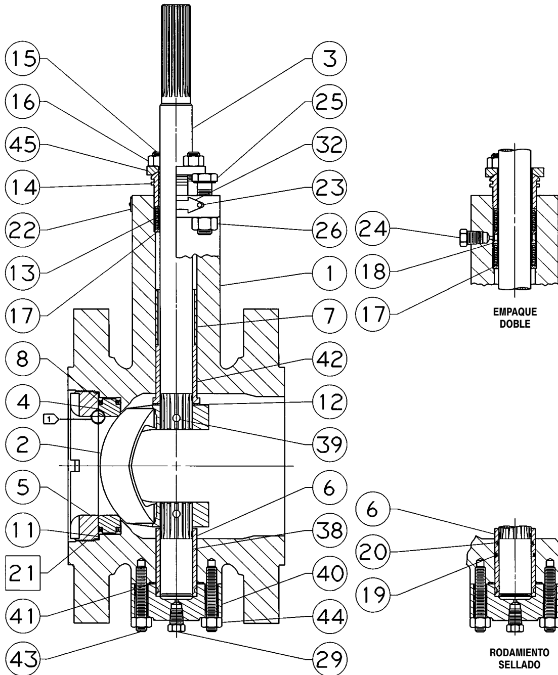
Figura 11. Válvula Fisher CV500, NPS 10 y 12
