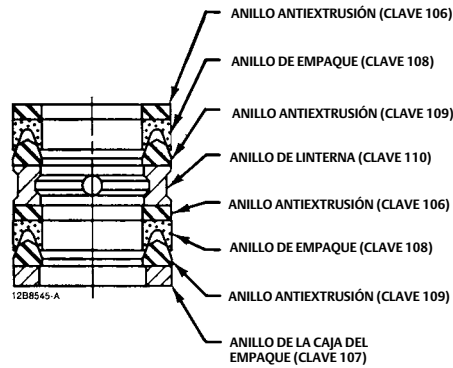
EMPAQUE DOBLE DE PTFE EN UNA CAJA DE PROFUNDIDAD ESTÁNDAR
