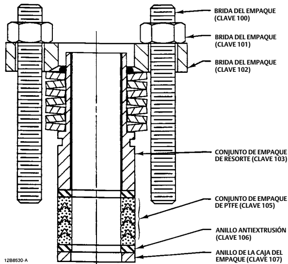
EMPAQUE INDIVIDUAL DE TEFLÓN EN UNA CAJA DE PROFUNDIDAD ESTÁNDAR
