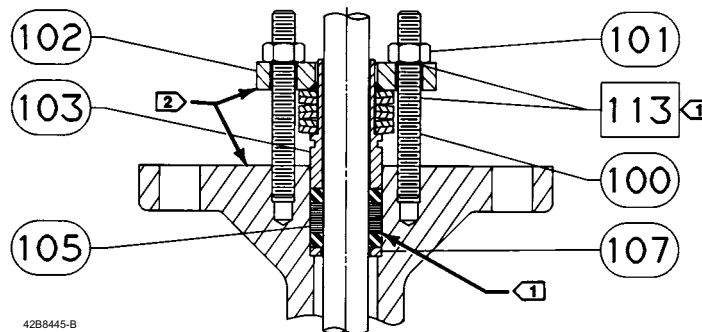
Ilustracja 14. Typowa dławnica ENVIRO-SEAL z pierścieniami grafitowymi do zaworów obrotowych
