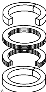
Ilustracja 14. Typowa dławnica ENVIRO-SEAL z pierścieniami grafitowymi do zaworów obrotowych
