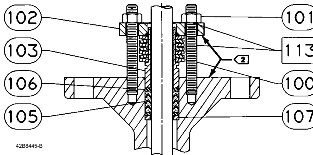
Ilustracja 13. Typowa dławnica ENVIRO-SEAL z pierścieniami z PTFE do zaworów obrotowych
