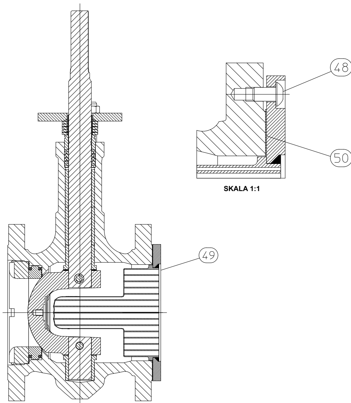
Ilustracja 16. Zespół zaworu Fisher CV500 z zespołem gniazdo-zawieradło Cavitrol Hex
