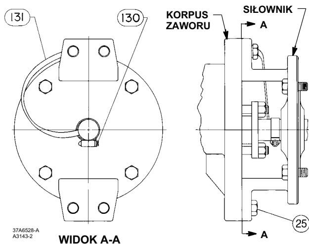
Ilustracja 3. Opcjonalny pasek uziemiający łączący wałek z korpusem
