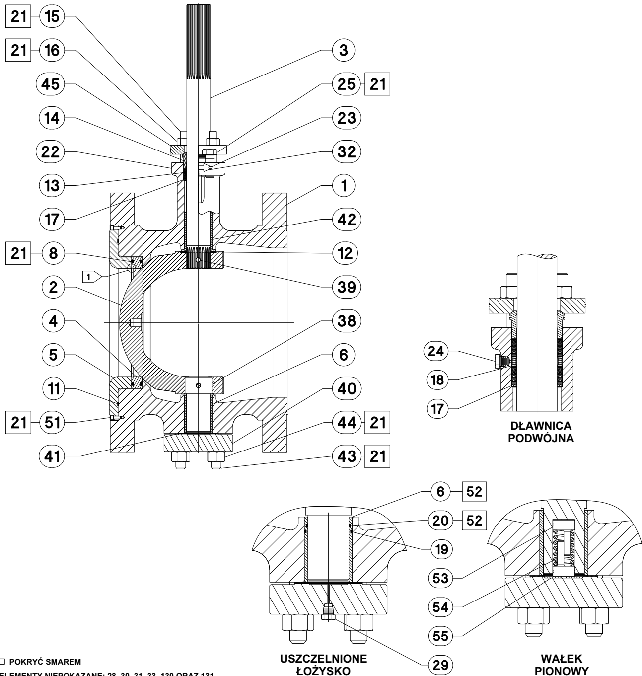
Rysunek 12. Zawór Fisher CV500, wielkość NPS 14 do 20
