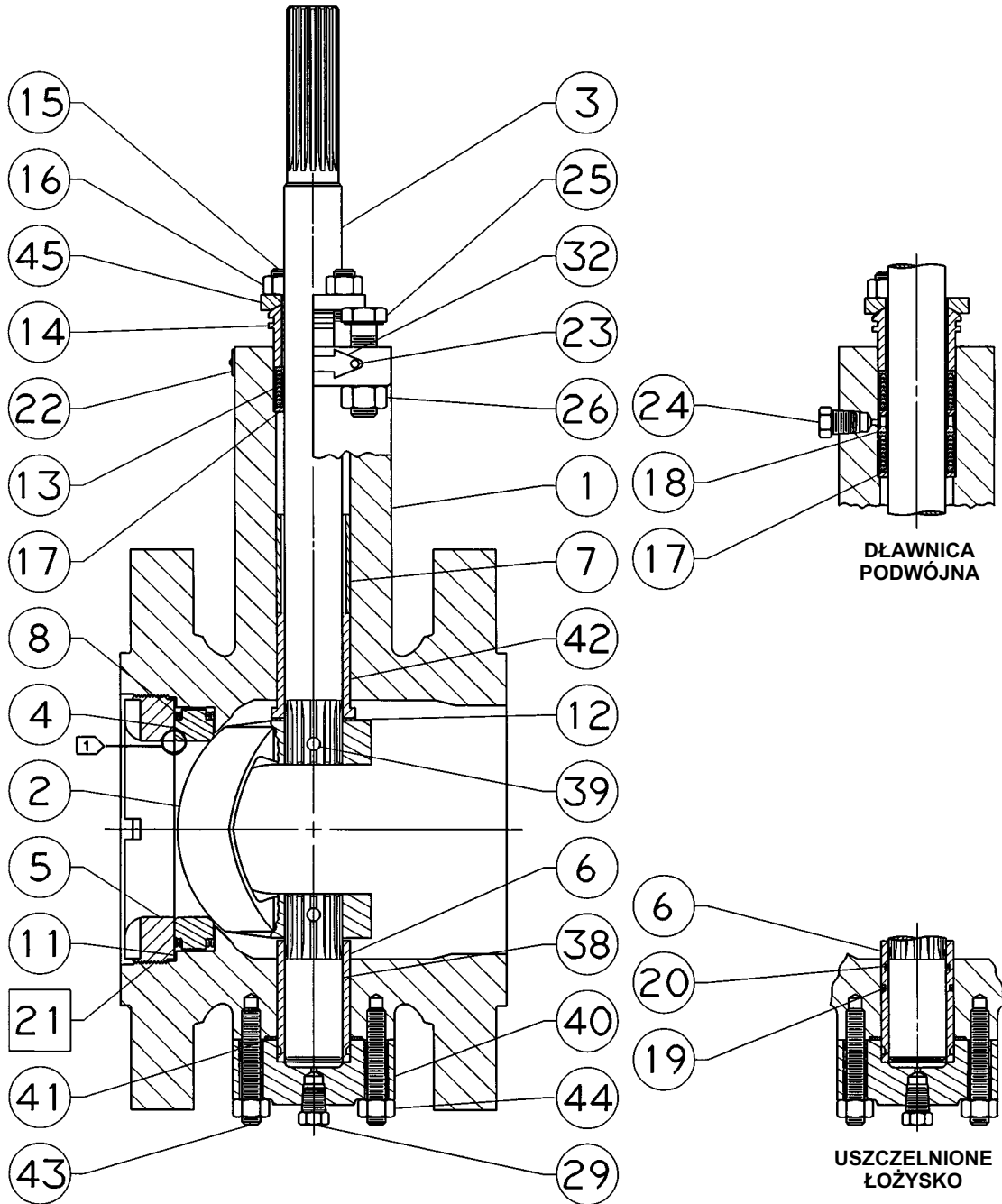
Ilustracja 11. Zawory Fisher CV500, wielkość NPS 10 i 12
