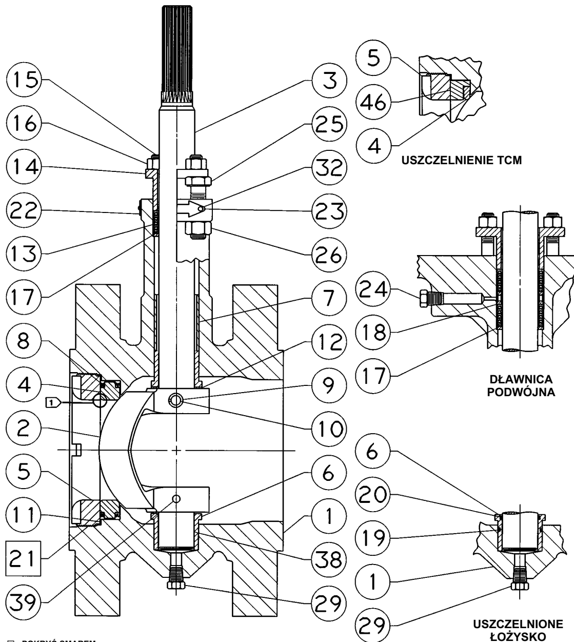
Ilustracja 10. Zawór Fisher CV500, wielkość NPS 3 do 8
