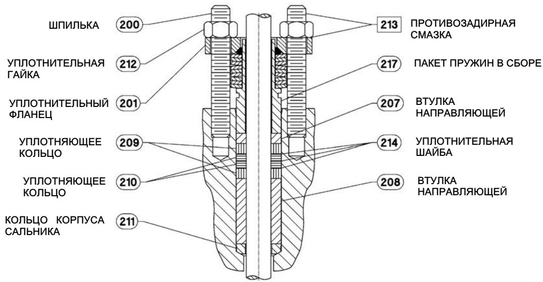
Рис. 7. Графитовое уплотнение ENVIRO SEAL ULF для клапанов easy-e компании Fisher
