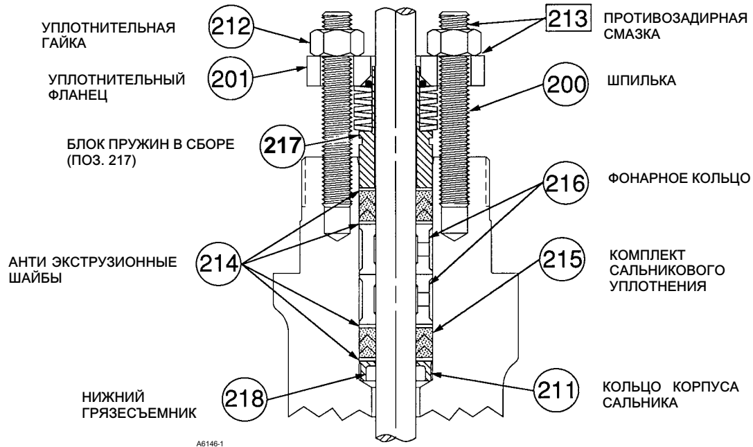
Рис. 5. Уплотнение ENVIRO-SEAL из ПТФЭ для клапанов с поступательным движением штока серии easy-e компании Fisher
