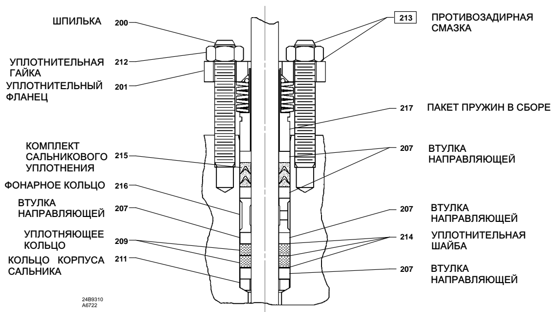
Рис. 6. Двойное сальниковое уплотнение ENVIRO-SEAL для клапанов серии easy-e компании Fisher
