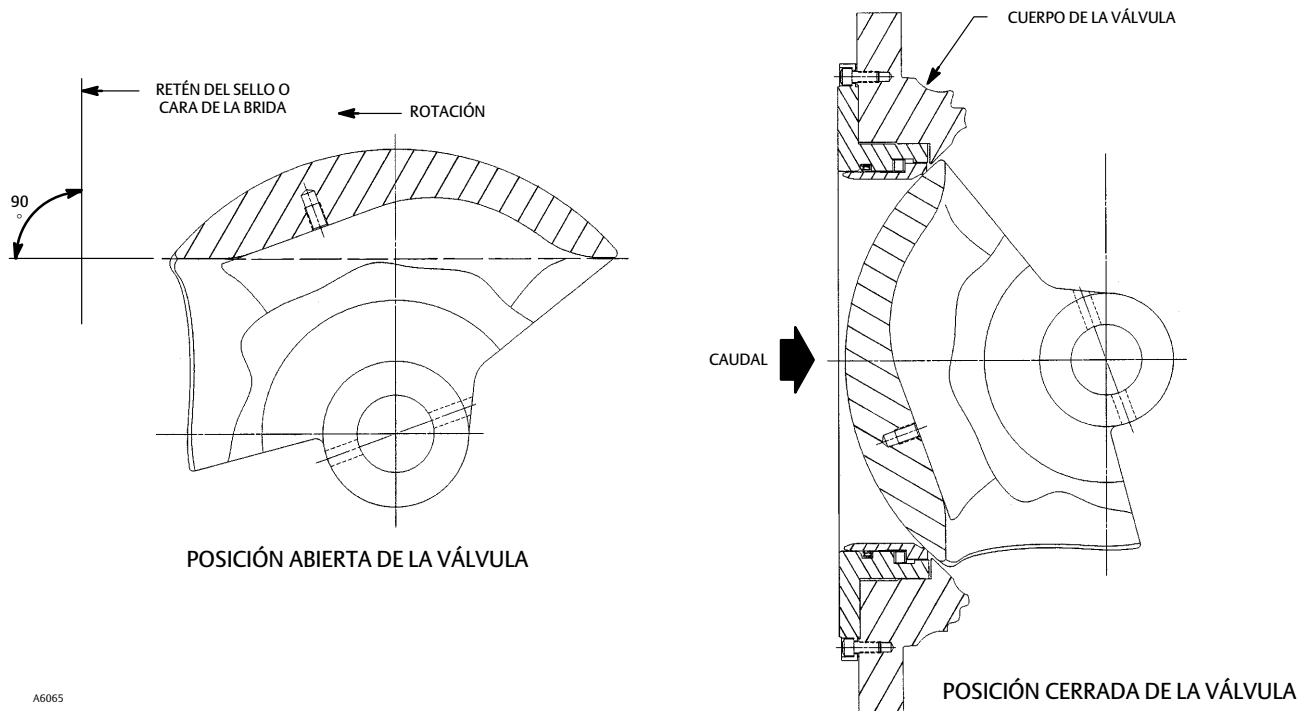
Figura 9. Determinación de la posición de la esfera
