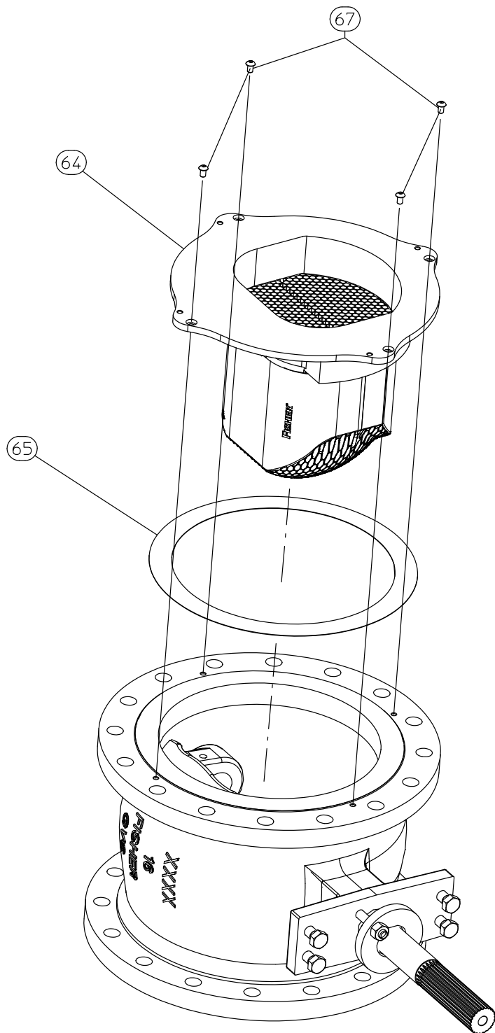
Figura 11. Vista de despiece de Fisher V150 con Cavitrol hexagonal
