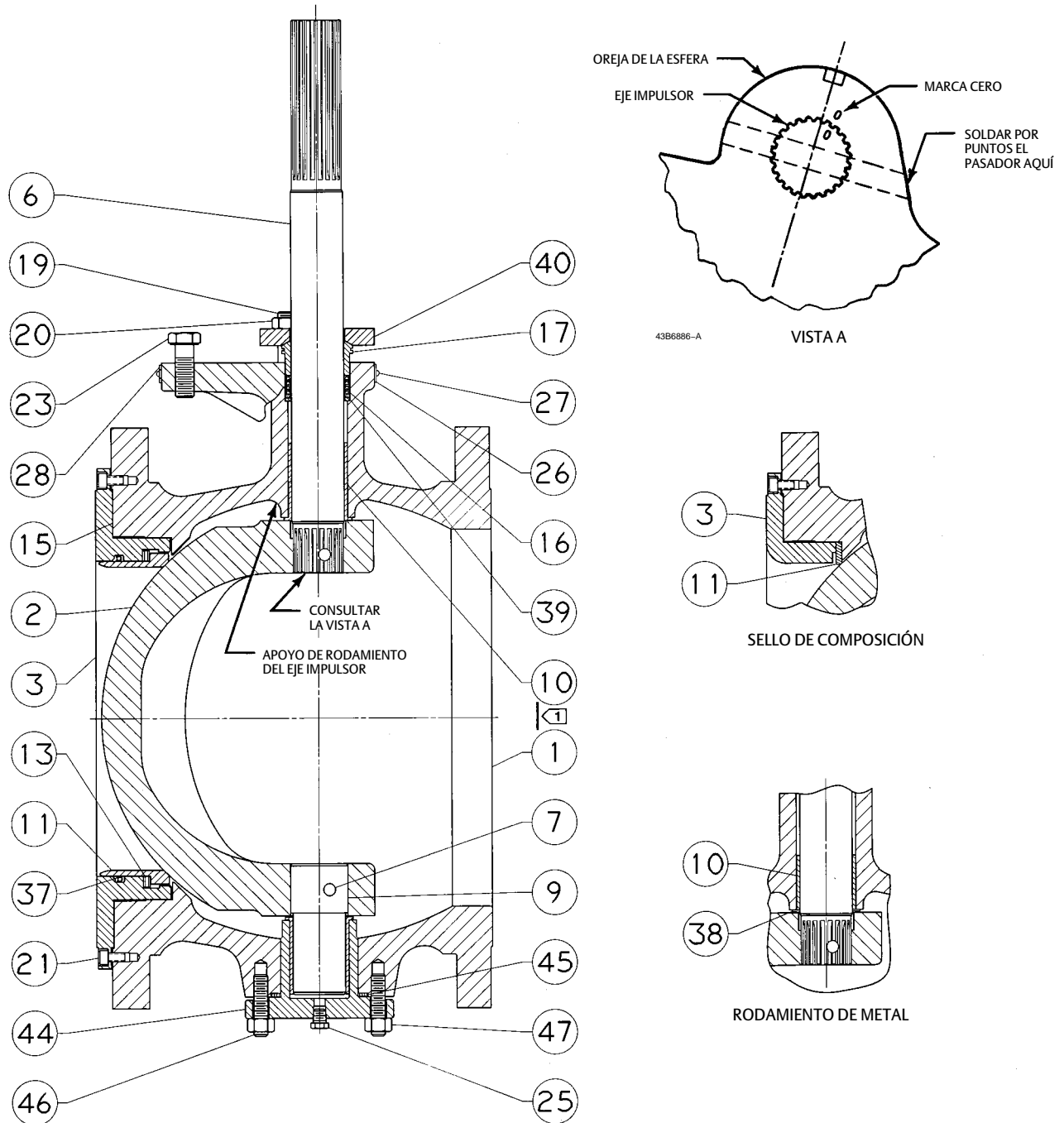
Figura 10. Conjunto de válvula Fisher V150 y V300
