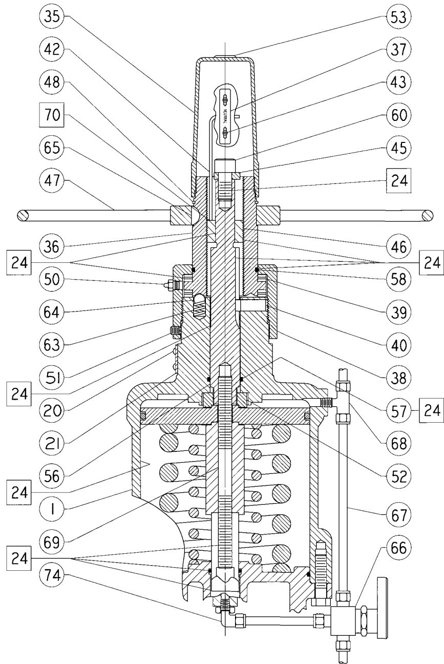
Figura 6. Conjunto de volante dos atuadores Fisher 585C Tamanhos 25 e 50 (mola retrai a haste do atuador)
