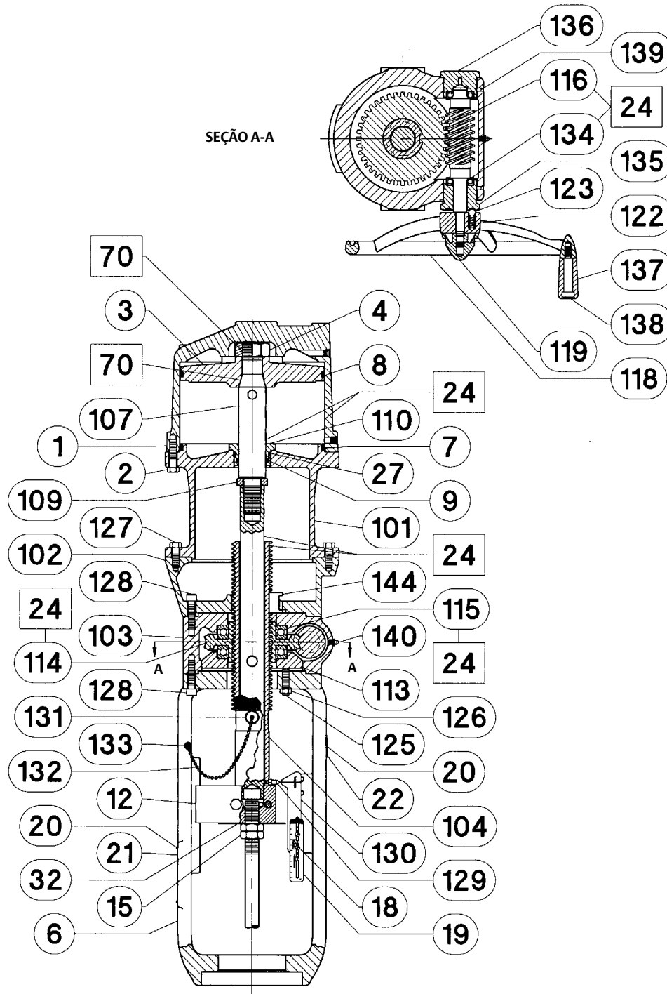
Figura 12. Atuador Fisher 585C com barra de elevação integral Tamanho 80 e 100 com deslocamento de 4 polegadas
