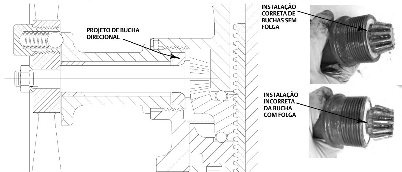
Figura 4. Projeto e instalação de bucha direcional do volante Fisher 585C tamanho 60 e 68
