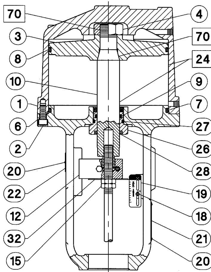
Figura 15. Atuador Fisher 585C Tamanho 60 com deslocamento de 8 polegadas e Tamanho 68 com deslocamento de 2, 4 e 8 polegadas
