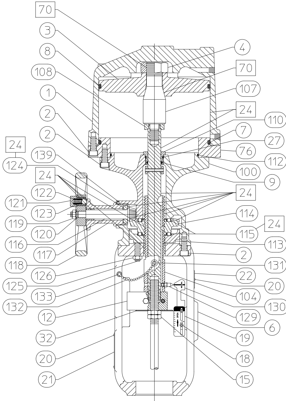
Figura 10. Atuador Fisher 585C com barra de elevação integral Tamanho 68 com deslocamento de 2 e 4 polegadas
