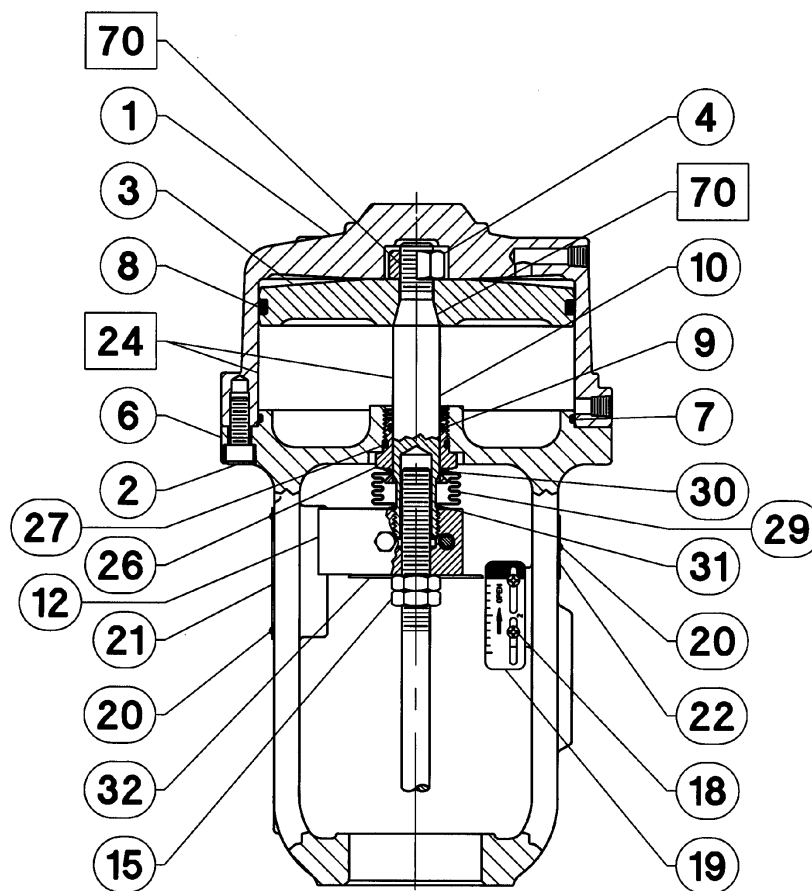
Figura 14. Atuador Fisher 585C Tamanho 60 com deslocamento de 2 e 4 polegadas
