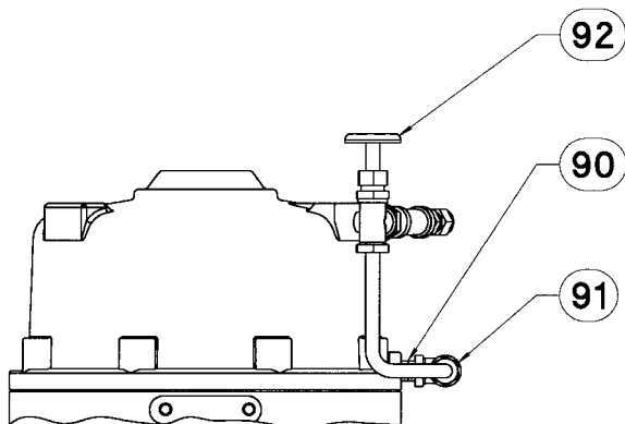
Figura 16. Conjunto de desvio Fisher 585C Tamanhos 60 a 130
