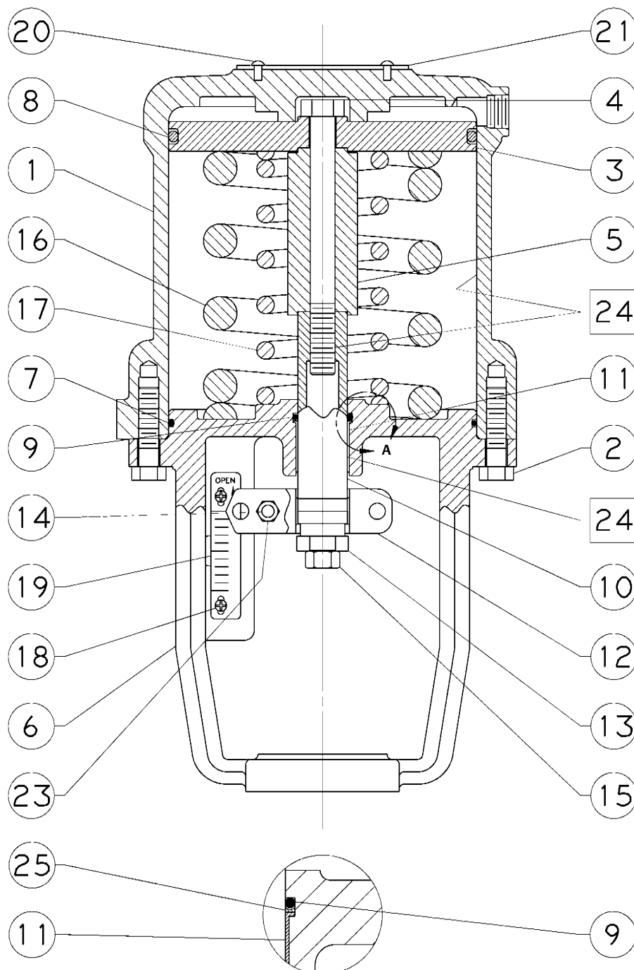
Figura 5. Atuadores Fisher 585C Tamanhos 25 e 50 (mola retrai a haste do atuador)
