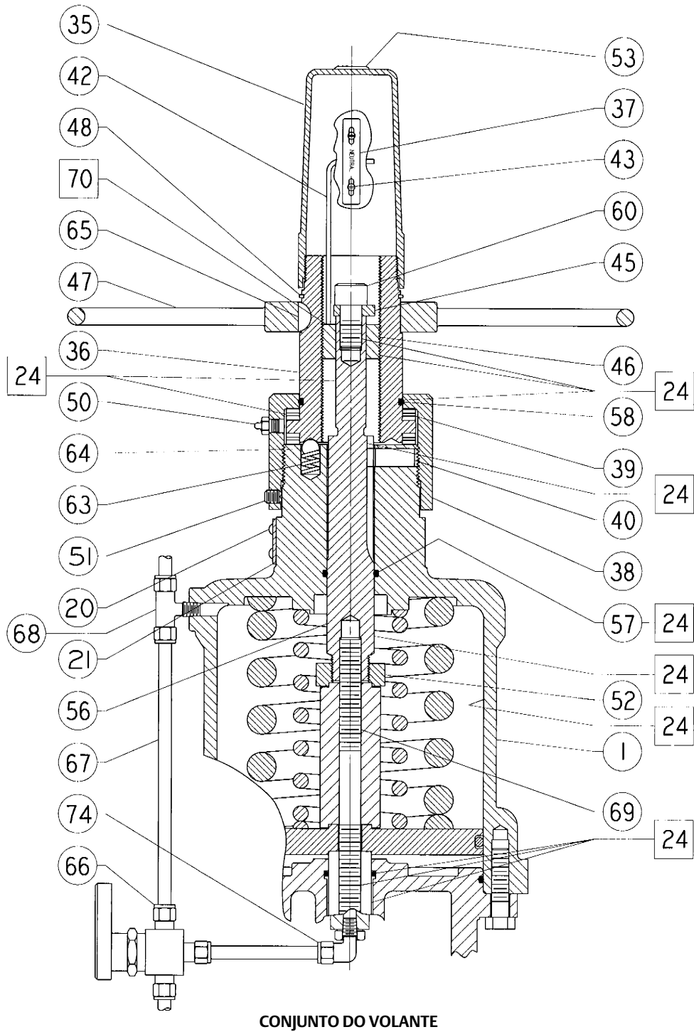
Figura 8. Conjunto de volante dos atuadores Fisher 585CR Tamanhos 25 e 50 (mola estende a haste do atuador)
