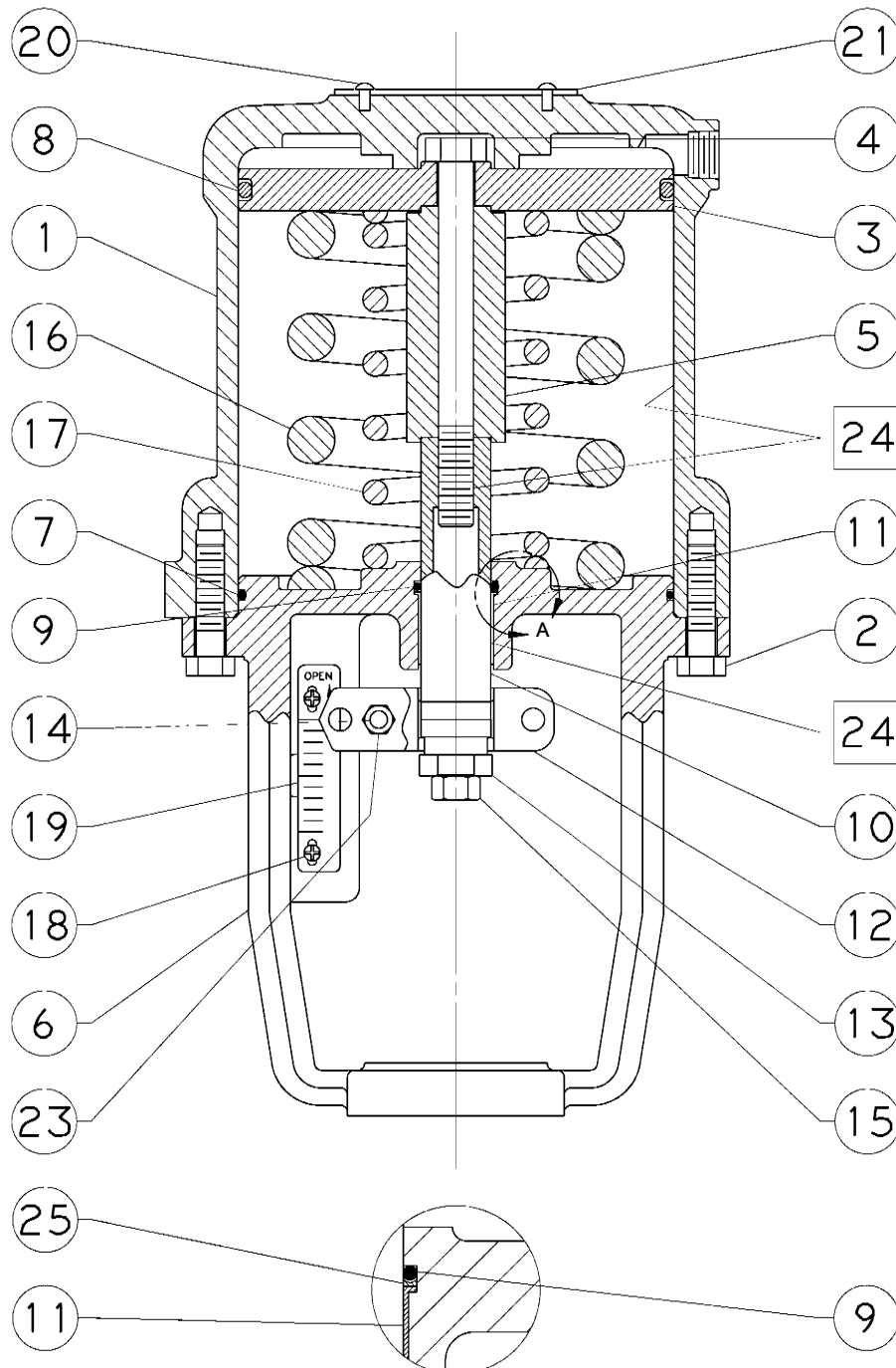
5 pav. 25 ir 50 dydžio pavaros mechanizmai „Fisher 585C“ (spyruoklė įtraukia pavaros mechanizmo kotą)
