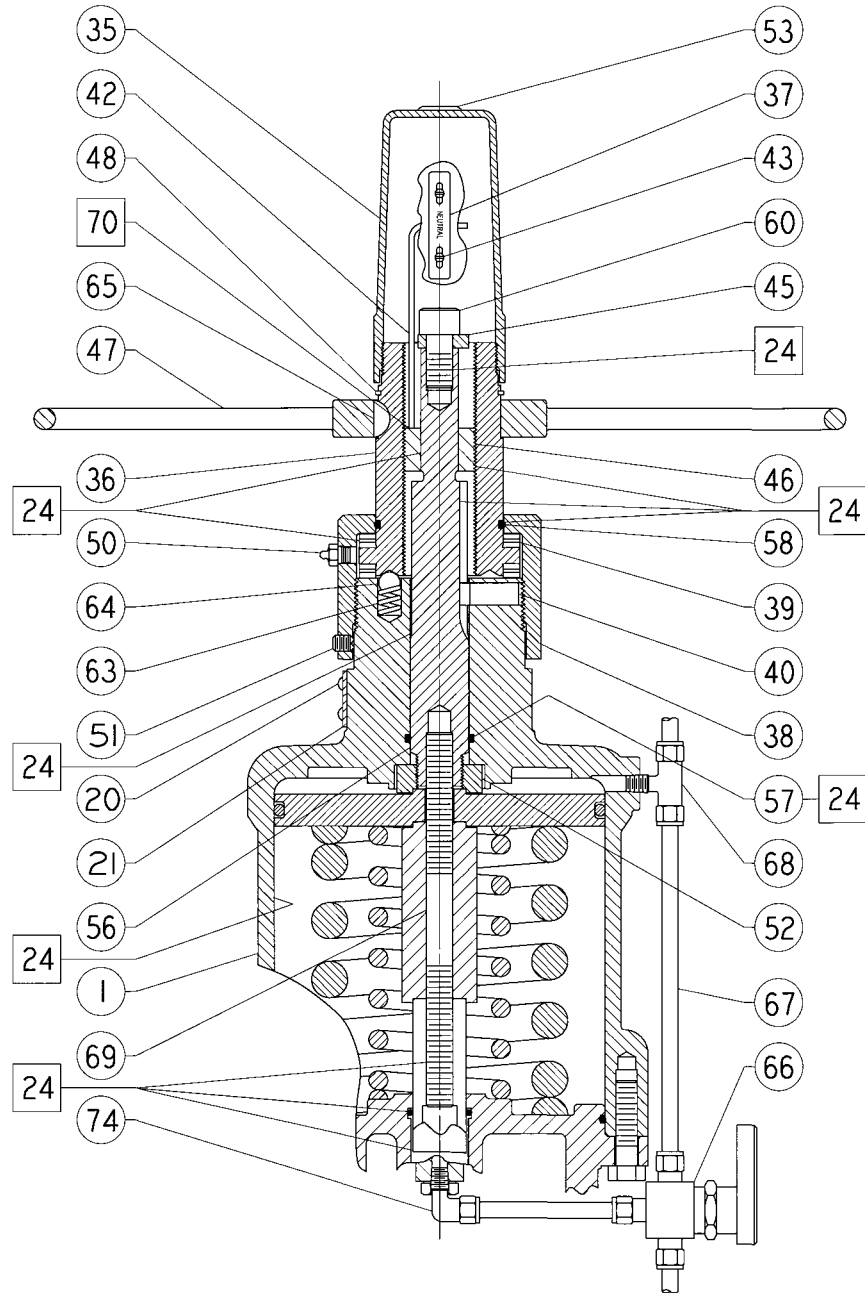
6 pav. 25 ir 50 dydžio pavaros mechanizmų „Fisher 585C“ rankinio valdymo rato blokas (spyruoklė įtraukia pavaros mechanizmo kotą)
