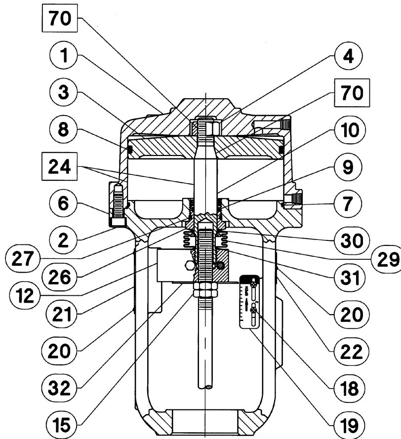
14 pav. 60 dydžio pavaros mechanizmas „Fisher 585C“ (2 ir 4 col. eiga)
