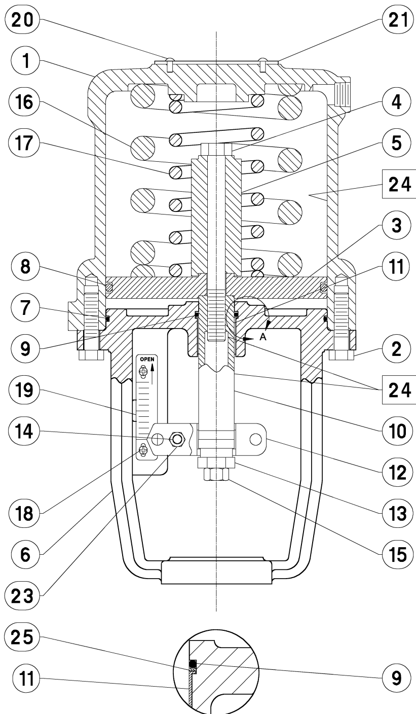
7 pav. 25 ir 50 dydžio pavaros mechanizmai „Fisher 585CR“ (spyruoklė ištraukia pavaros mechanizmo kotą)
