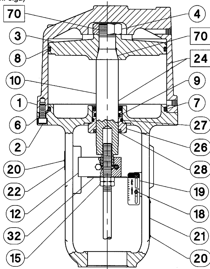
15 pav. 60 dydžio pavaros mechanizmas „Fisher 585C“ (8 col. eiga) ir 68 dydžio pavaros mechanizmas „Fisher 585C“ (2, 4 ir 8 col. eiga)
