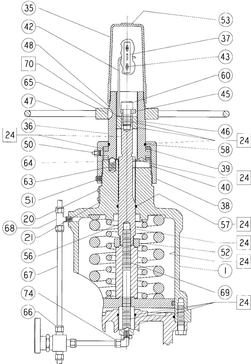
8 pav. 25 ir 50 dydžio pavaros mechanizmo „Fisher 585CR“ rankinio valdymo rato blokas (spyruoklė ištraukia pavaros mechanizmo kotą)
