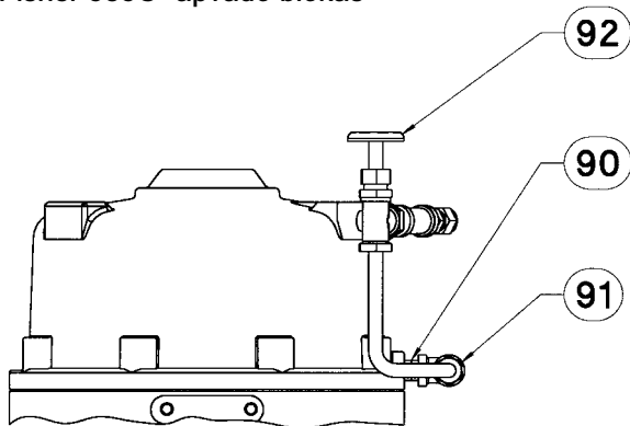
16 pav. 60 - 130 dydžio pavaros mechanizmų „Fisher 585C“ apvado blokas
