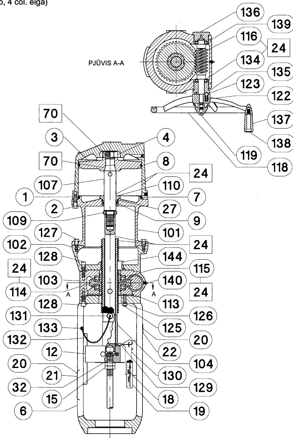
12 pav. Pavaros mechanizmas „Fisher 585C“ su integruotu rankinio valdymo ratu (80 ir 100 dydžio, 4 col. eiga)
