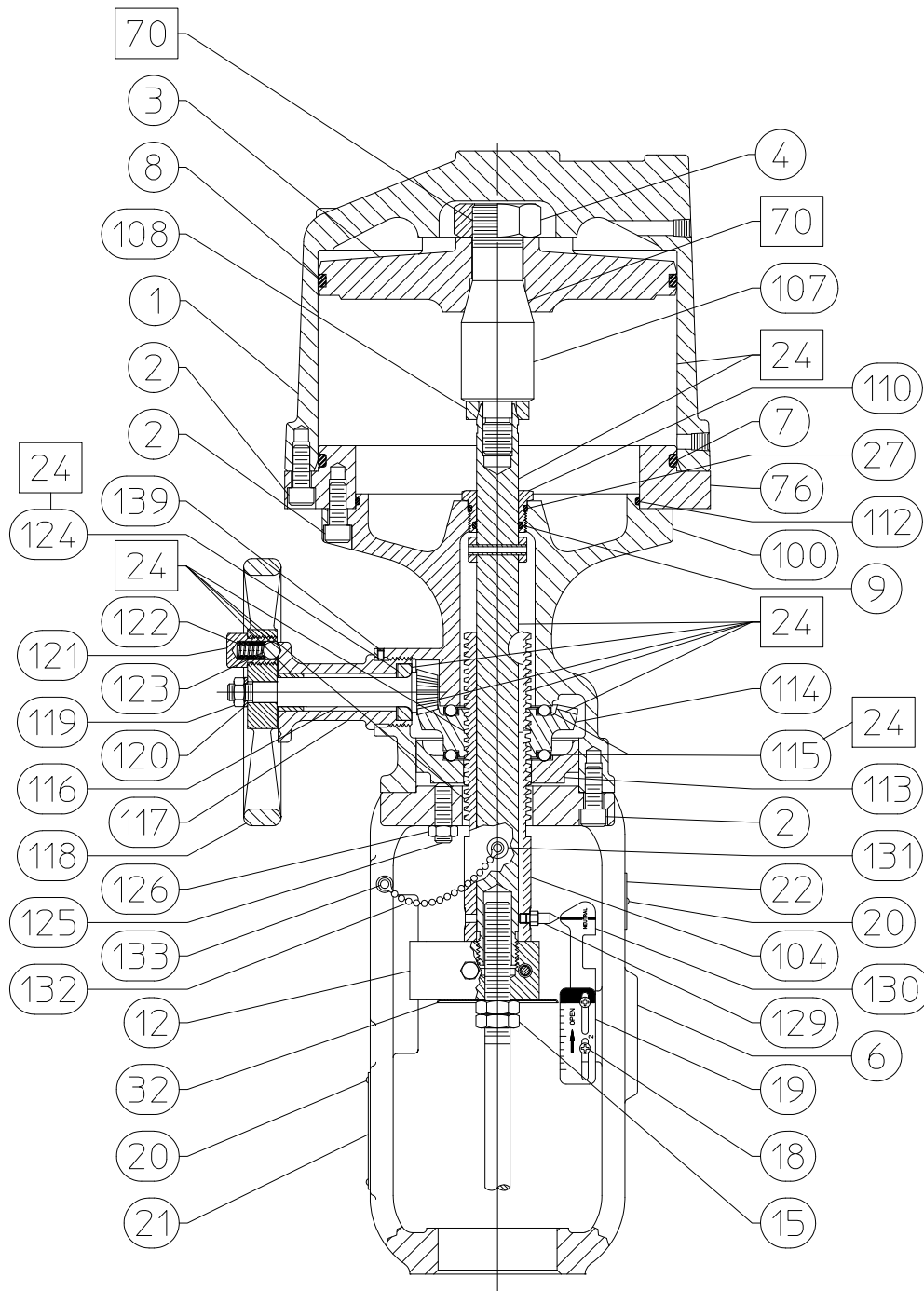
10 pav. Pavaros mechanizmas „Fisher 585C“ su integruotu rankinio valdymo ratu (68 dydžio, 2 ir 4 col. eiga)
