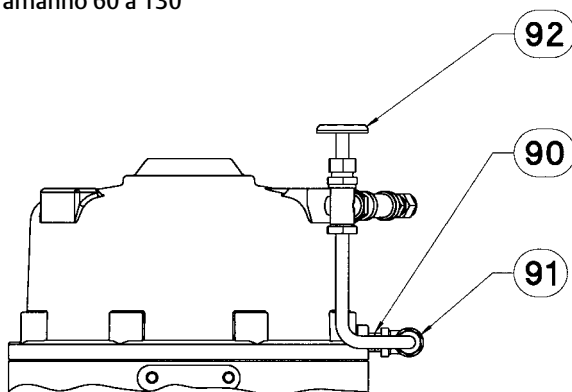
Figura 16. Conjunto de Bypass 585C da Fisher Tamanho 60 a 130
