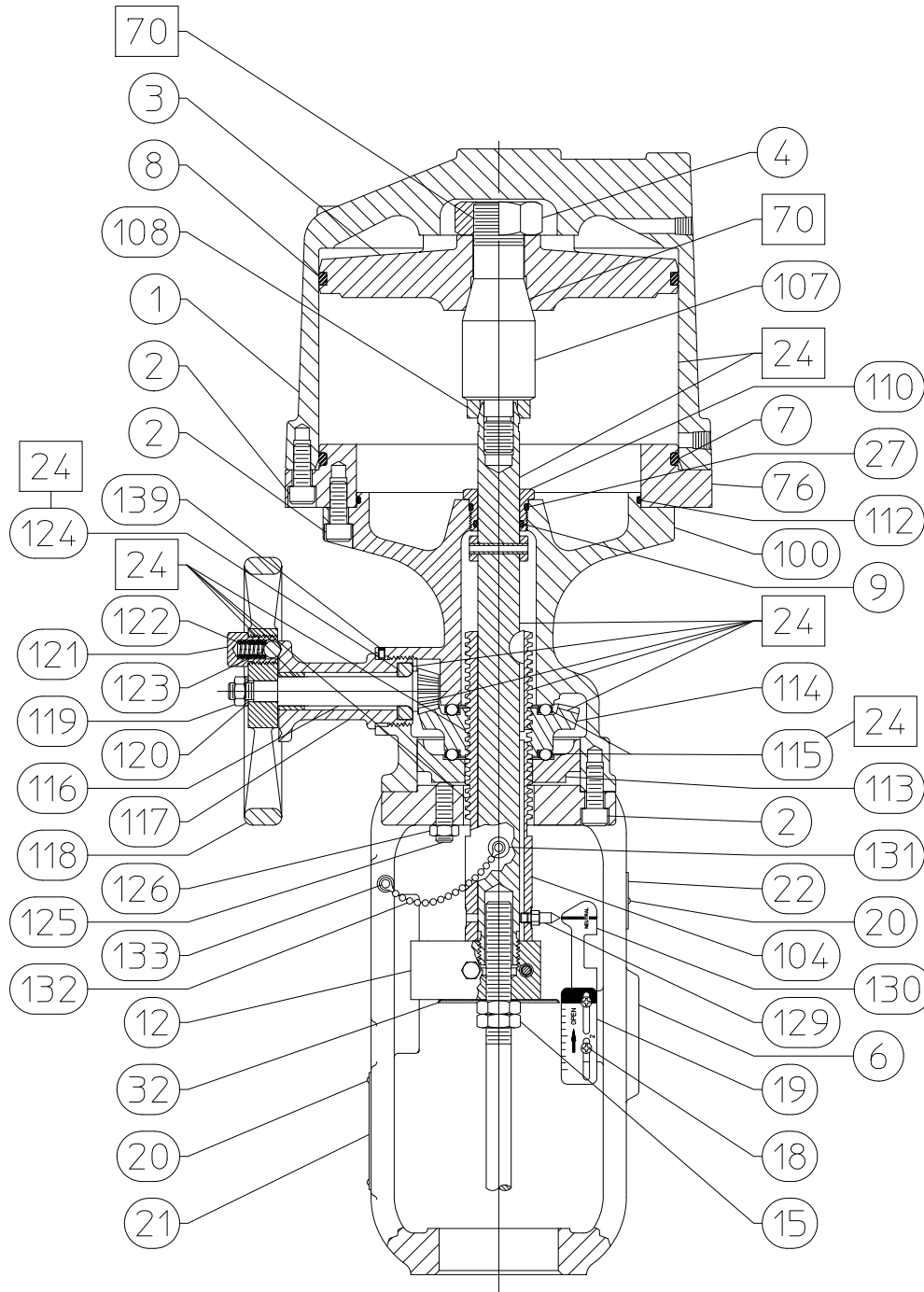
Figura 10. Actuador 585C da Fisher com Suporte Manual Integral Tamanho 68 com Deslocamento de 2 e 4 Pol.
