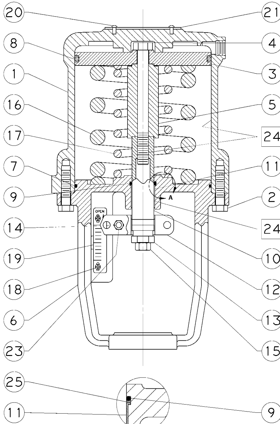
VISTA A TAMANHO 50
