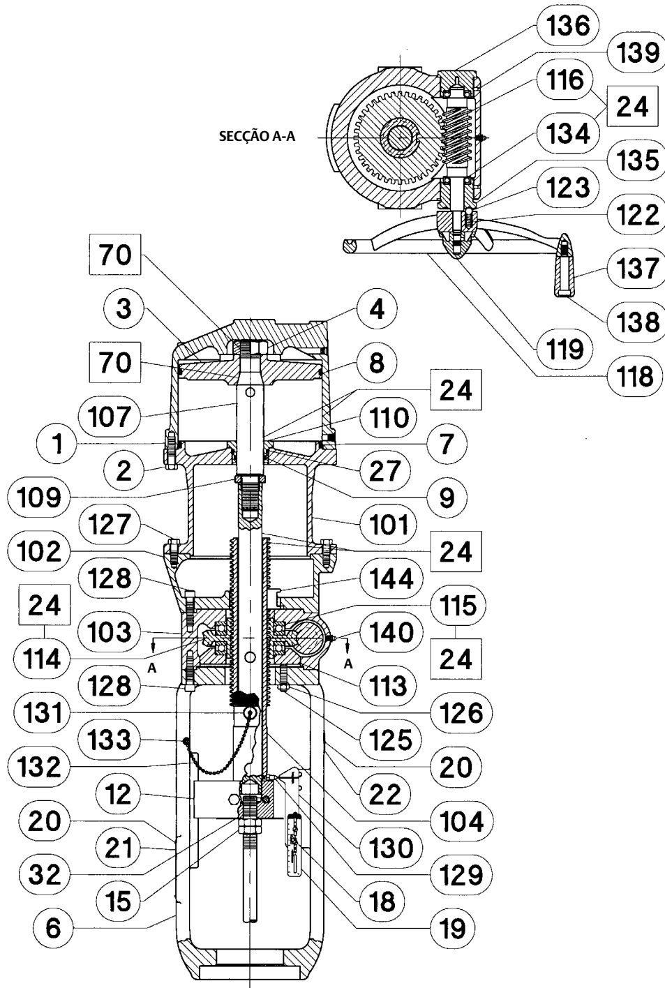
Figura 12. Actuador 585C da Fisher com Suporte Manual Integral Tamanho 80 e 100 com Deslocamento 4 Pol.
