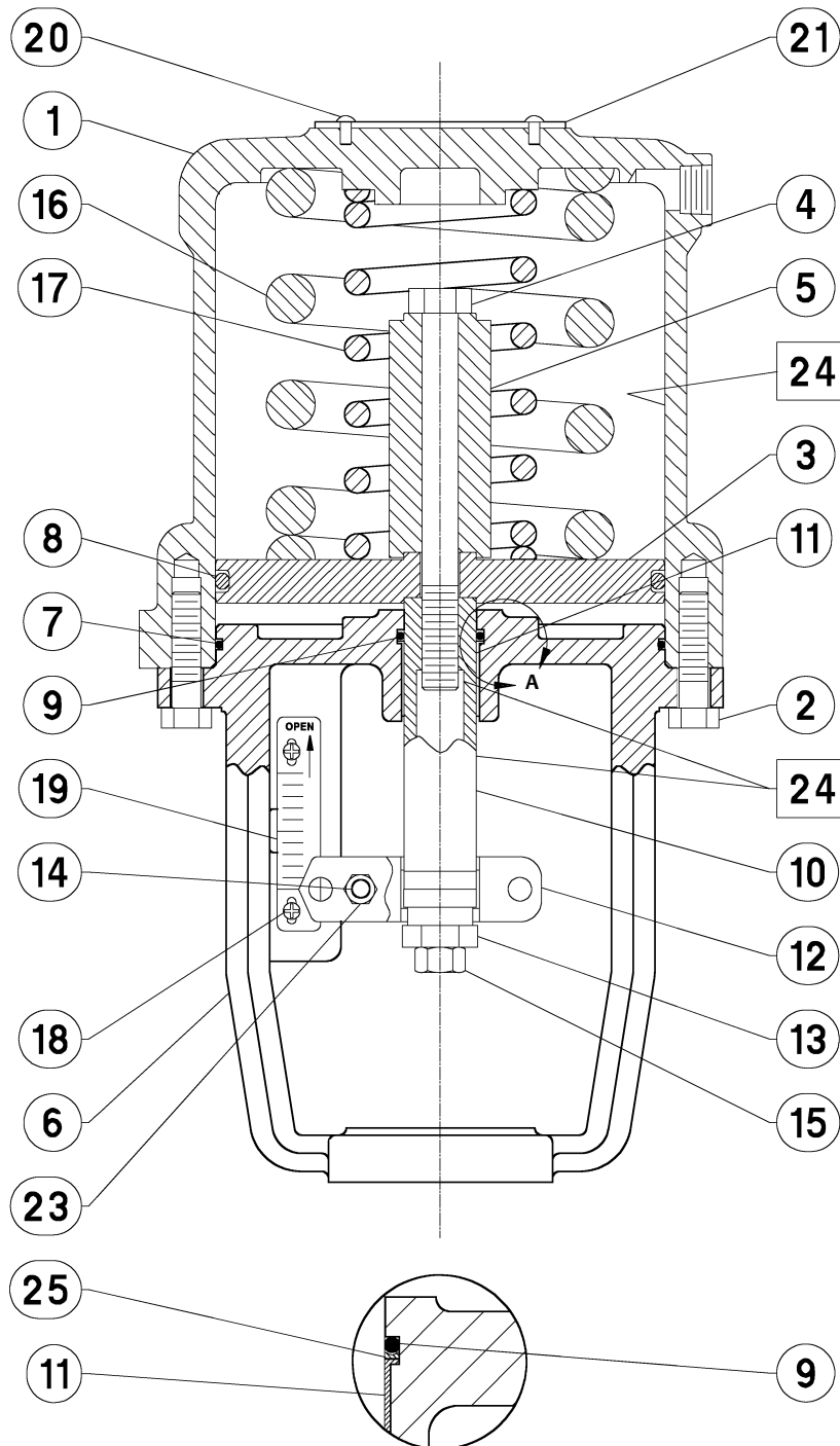
Figura 7. Actuadores 585CR da Fisher, Tamanhos 25 e 50 (a mola estende o tirante do actuador)
