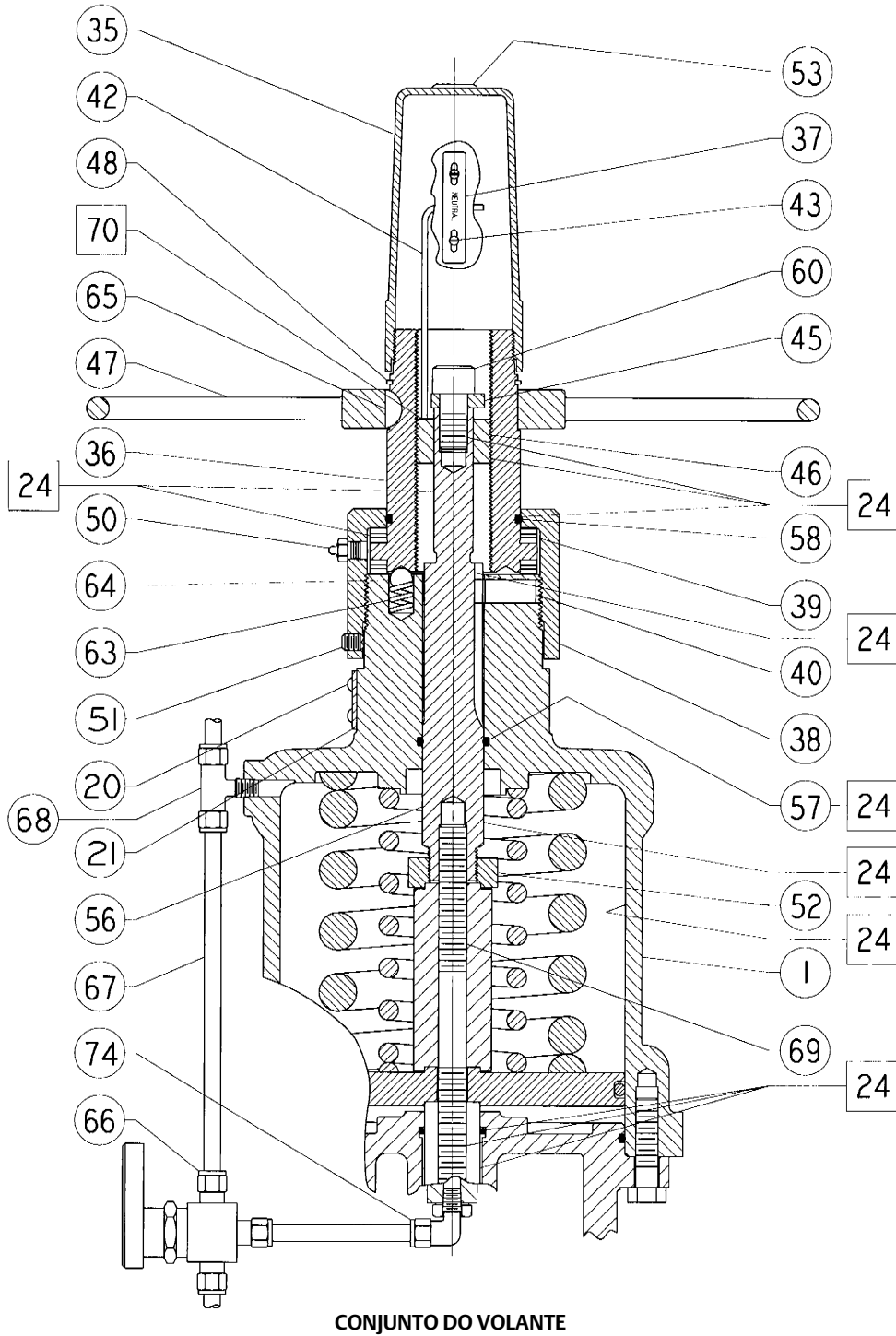
Figura 8. Conjunto do Volante de Actuadores 585CR da Fisher, Tamanhos 25 e 50 (a mola estende o tirante do actuador)
