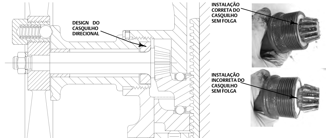
Figura 4. Desenho e instalação do casquilho direcional do volante Fisher 585C tamanho 60 e 68
