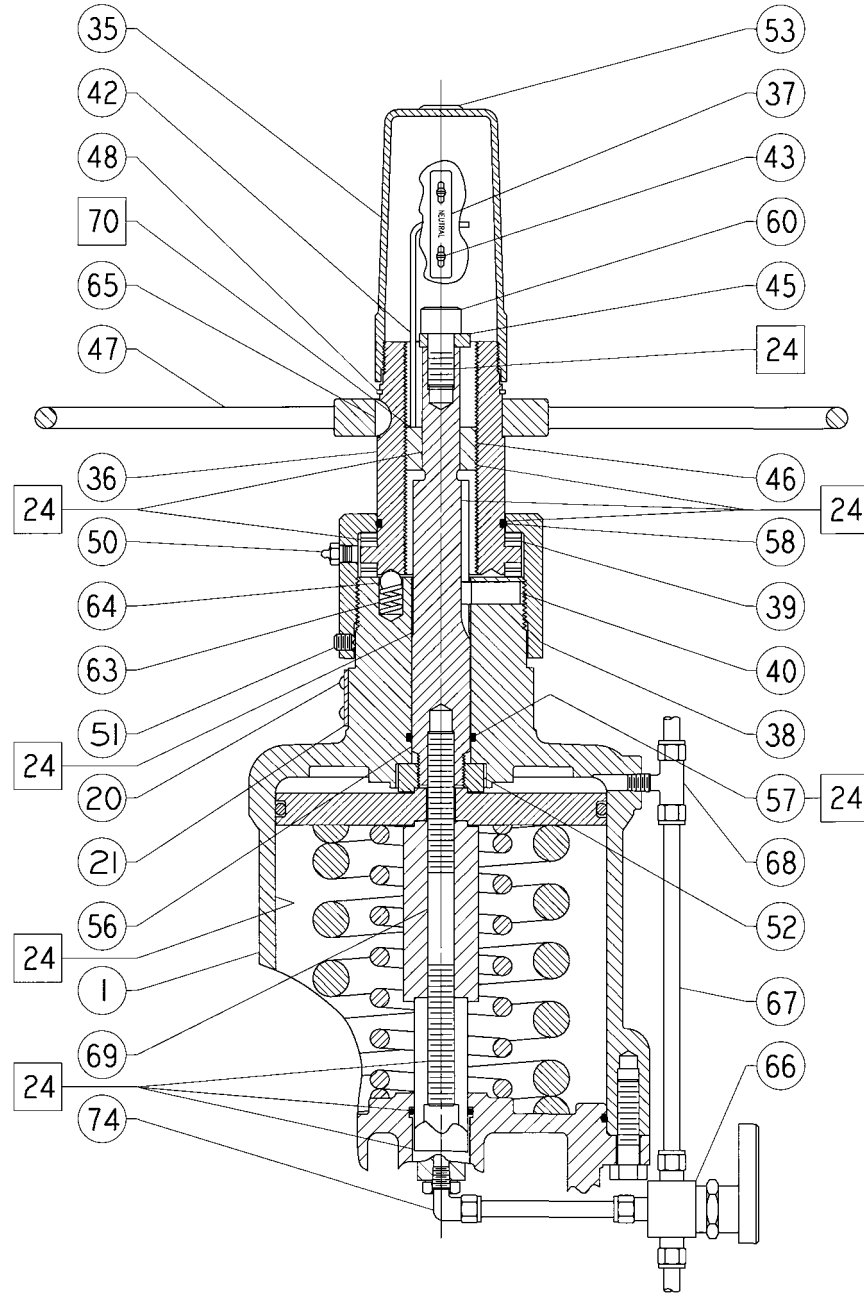
Figura 6. Conjunto do Volante de Actuadores 585C da Fisher Tamanhos 25 e 50 (a mola retrai o tirante do actuador)
