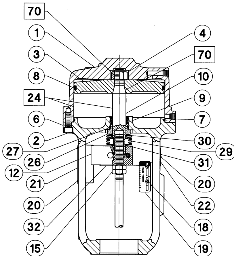
Figura 14. Actuador 585C da Fisher Tamanho 60 com Deslocamento de 2 e 4 Pol.
