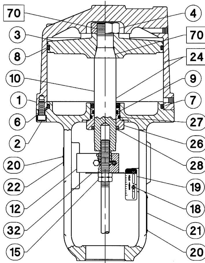
Figura 15. Actuador 585C da Fisher Tamanho 60 com Deslocamento de 8 Pol. e Tamanho 68 com Deslocamento de 2, 4 e 8 Pol.
