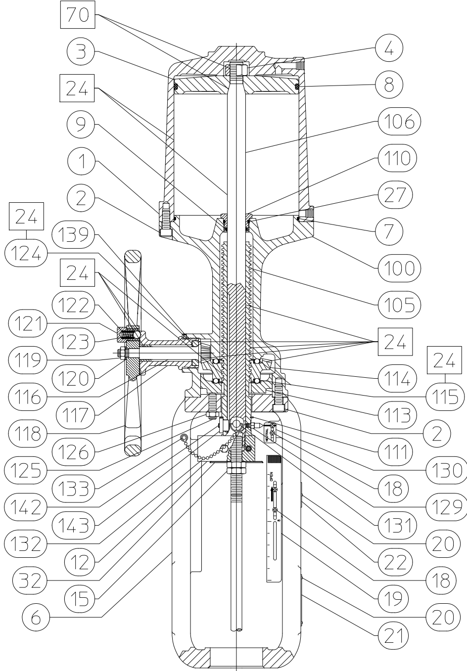
Şekil 11. 8 İnç Hareket Mesafeli Entegre Kriko bulunan 60 Ebat Fisher 585C Aktüatör
