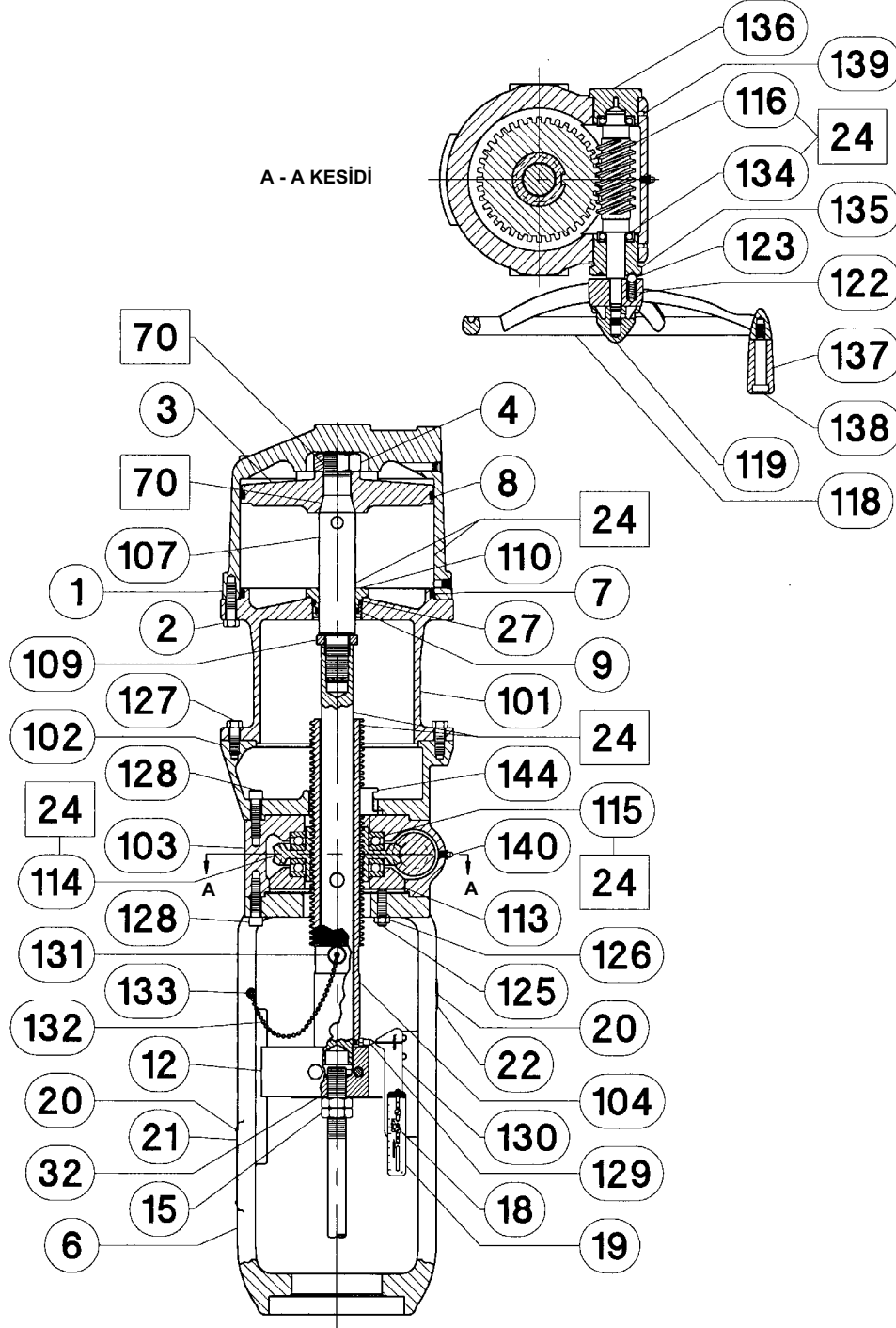
Şekil 12. 4 İnç Hareket Mesafeli Entegre Volanlı 80 ve 100 Ebat Fisher 585C Aktüatörler
