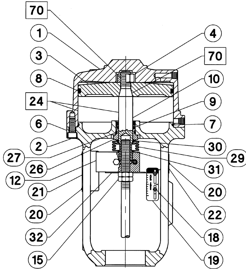
Şekil 14. 2 ve 4 İnç Hareket Mesafeli 60 Ebat Fisher 585C Aktüatörler
