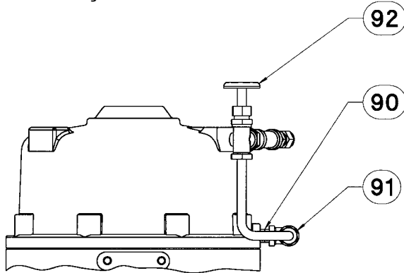
Şekil 16. 60 - 130 Arası Ebatlı Fisher 585C Aktüatör Aşırma Grubu
