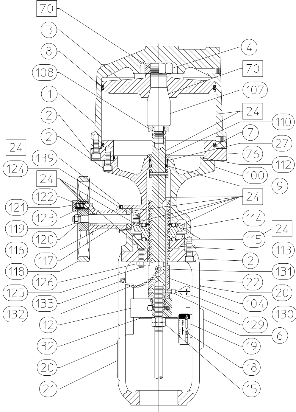
Şekil 10. 2 ve 4 İnç Hareket Mesafeli Entegre Volanlı 68 Ebat Fisher 585C Aktüatörler
