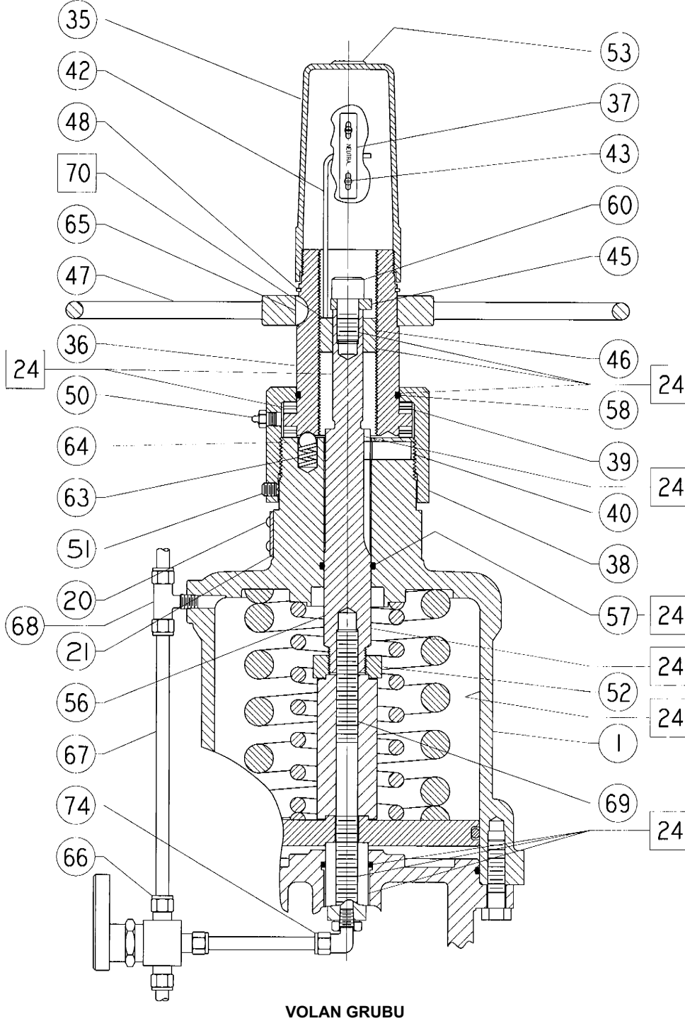
Şekil 8. 25 ve 50 Ebat Fisher 585CR Aktüatörlerin Volan Grubu (yay aktüatör gövdesini uzatır)
