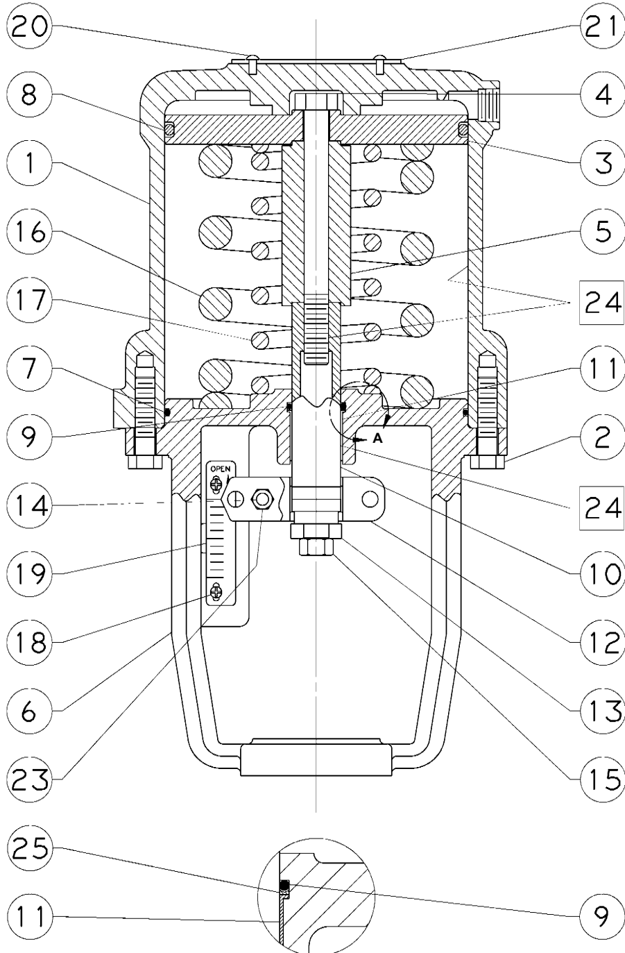
A GÖRÜNÜMÜ 50 EBAT
