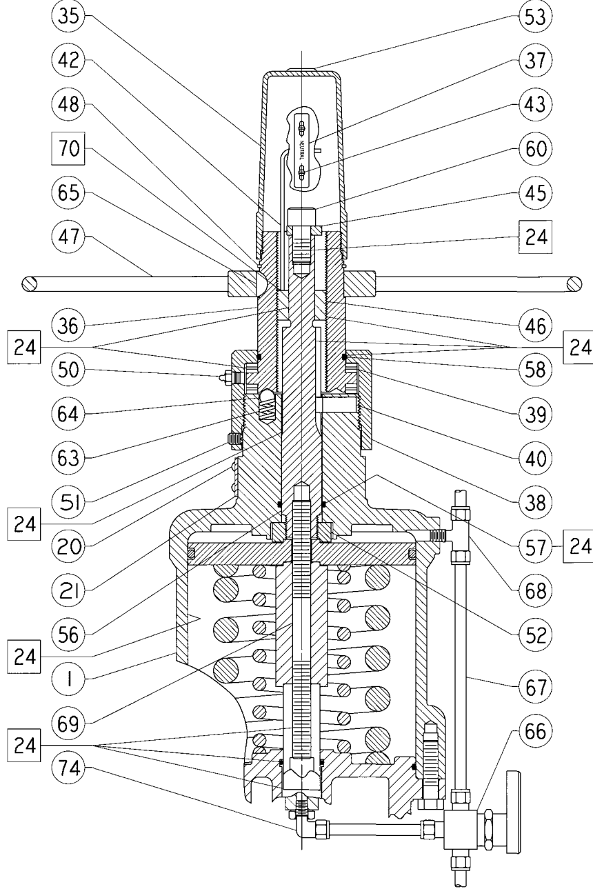
Şekil 6. 25 ve 50 Ebat Fisher 585C Aktüatörlerin Volan Grubu (yay aktüatör gövdesini geri çeker)
