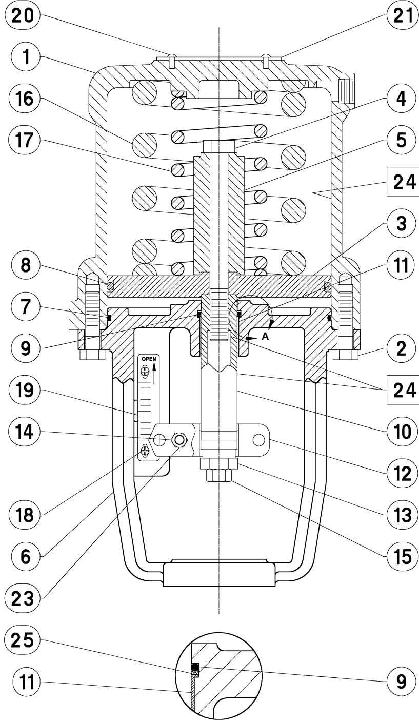
Şekil 7. 25 ve 50 Ebat Fisher 585CR Aktüatörler (yay aktüatör gövdesini uzatır)
