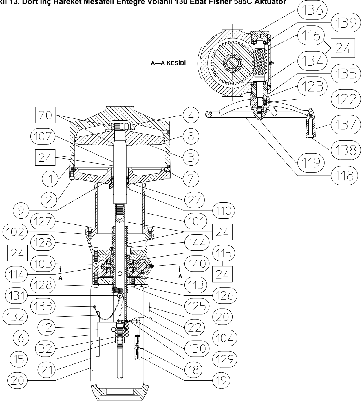
Şekil 13. Dört inç Hareket Mesafeli Entegre Volanlı 130 Ebat Fisher 585C Aktüatör
