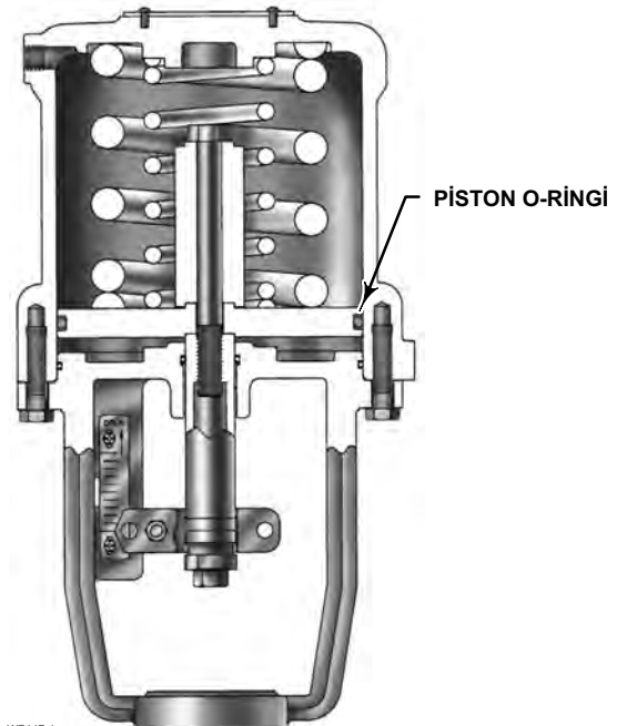
Şekil 3. Yayla Geri Çekilen Fisher 585C Pistonlu Aktüatör
