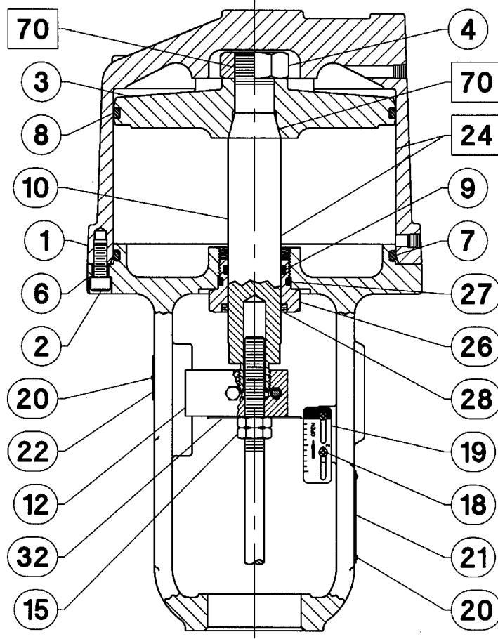
Şekil 15. 8 İnç Hareket Mesafeli 60 Ebat ve 2, 4 ve 8 İnç Hareket Mesafeli 68 Ebat Fisher 585C Aktüatörler
