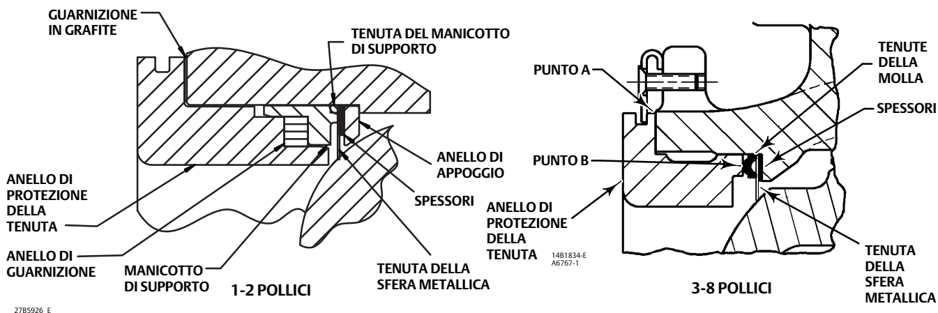
Figura 1. Dettaglio di una tenuta metallica SS-252B Fisher con molle multiple
