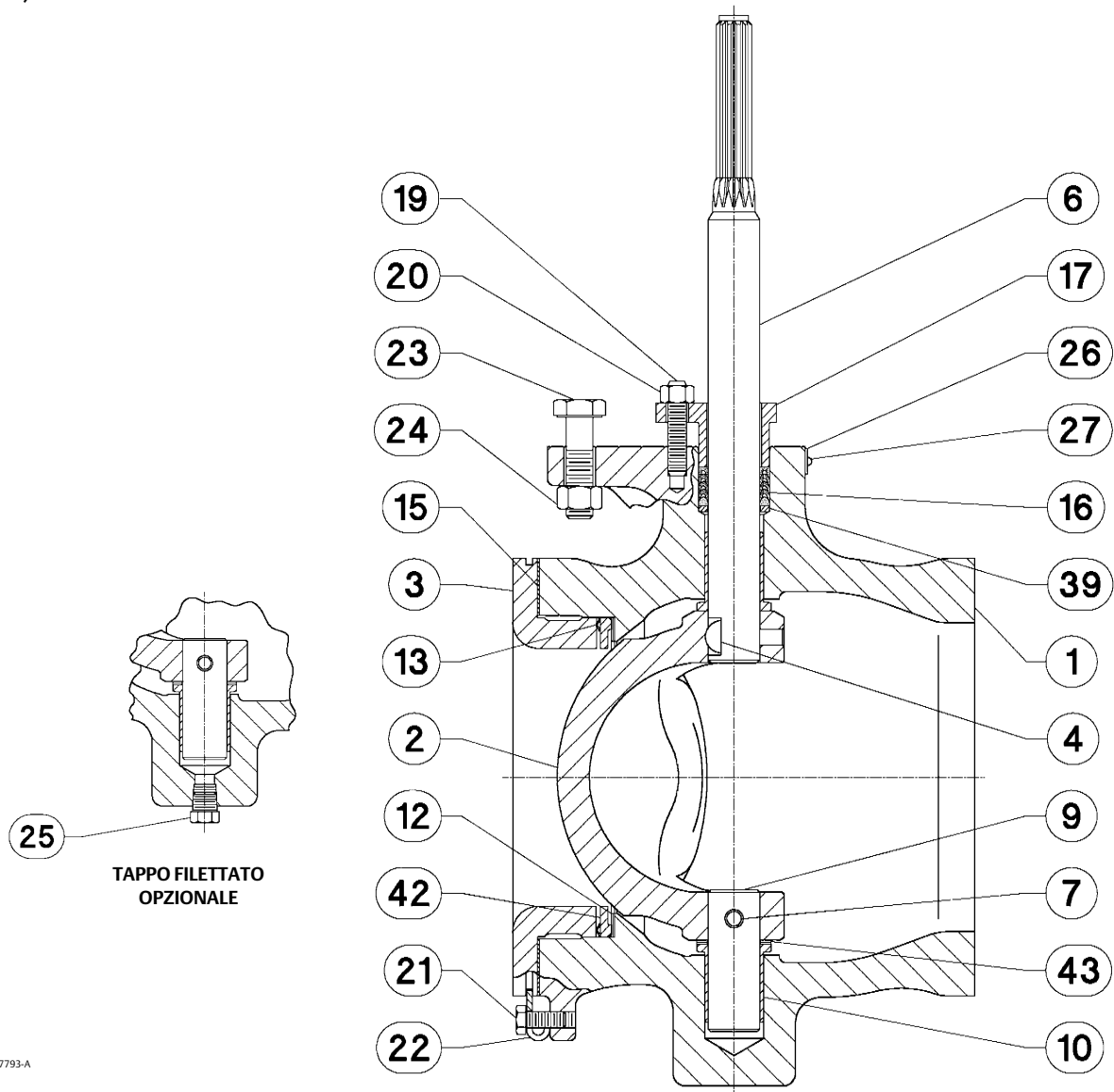
Figura 3. Gruppo valvola SS-138B Fisher (dettagli comuni anche alla valvola SS-252B, tranne che per la parte della tenuta)
