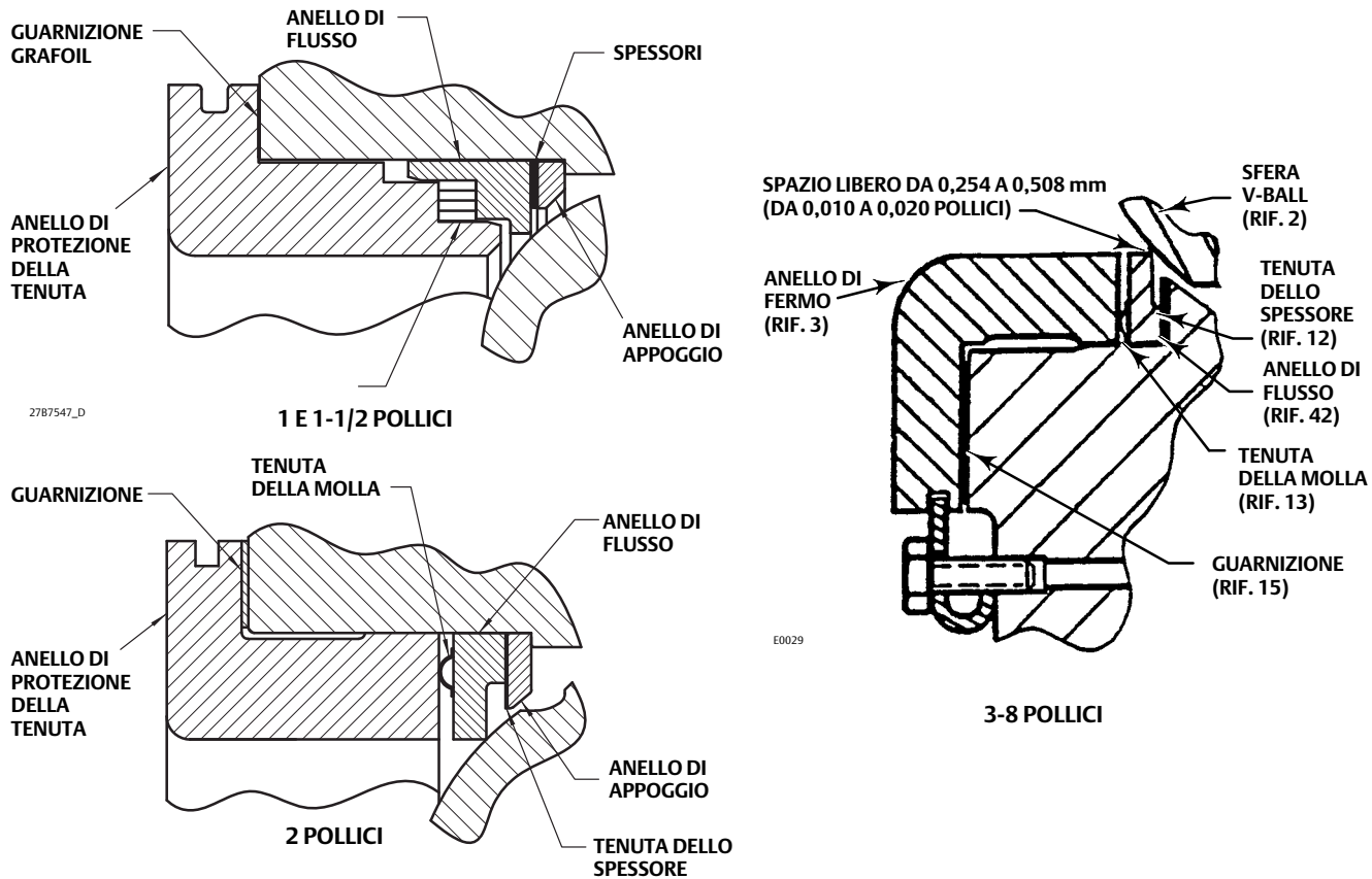
Figura 2. Dettagli della tenuta delle valvole SS-138B Fisher
