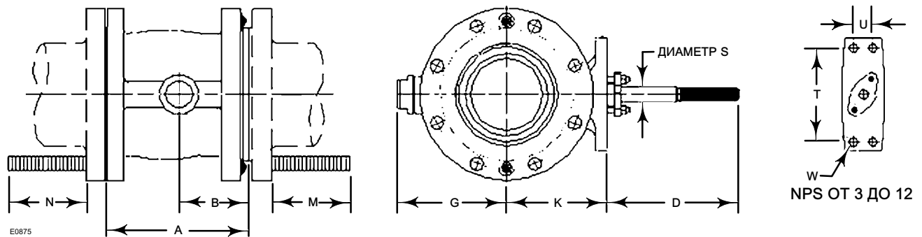
Рис. 4. Габаритные размеры шламового регулирующего клапана Fisher Vee-Ball (см. Табл. 4 и 5)
