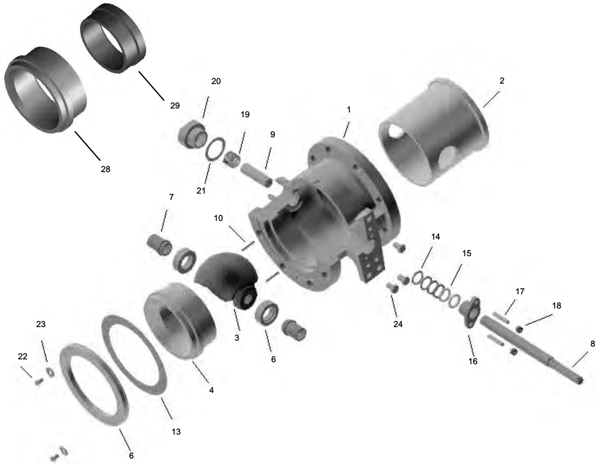
Рис. 9. Покомпонентное изображение: шламный регулирующий клапан Fisher Vee-Ball, размеры NPS 3 -12 (включая альтернативную конструкцию керамической вкладки, поз. 28 и 29)
