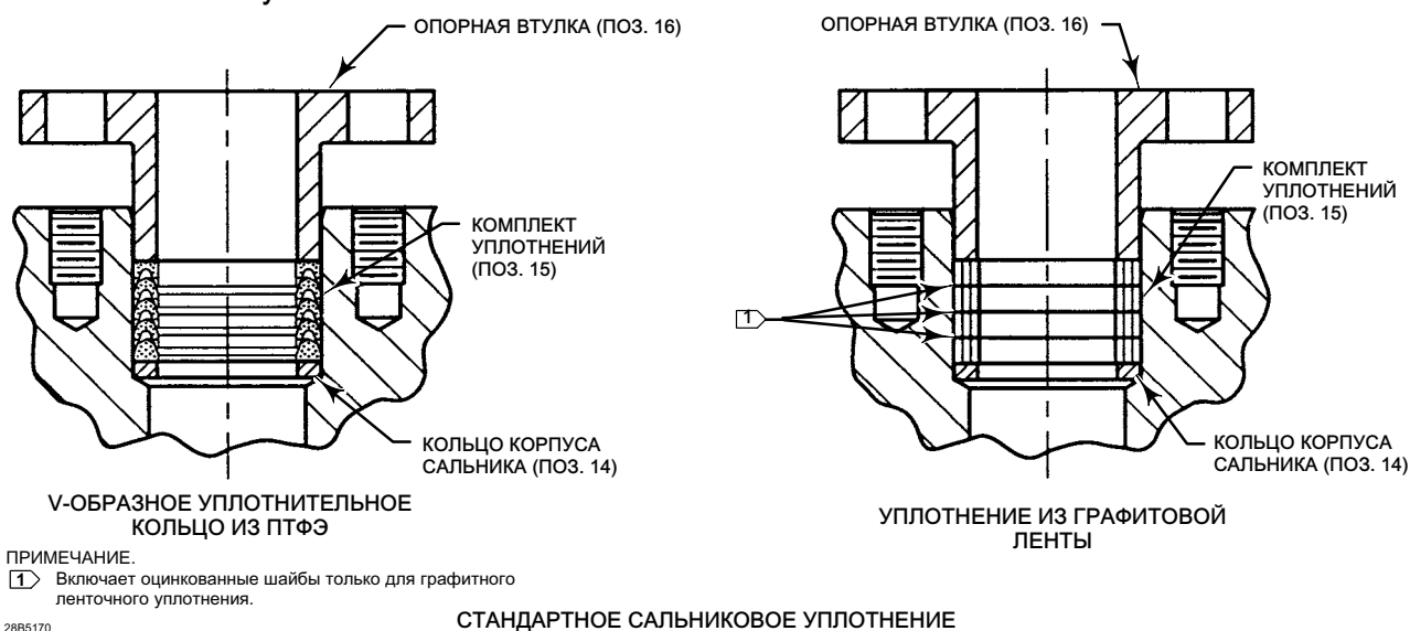
Рис. 6. Компоновки уплотнений
