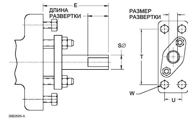
Рис. 5. Размеры шламового клапана Fisher Vee-Ball для приводного вала с лысками (см. табл. 6)
