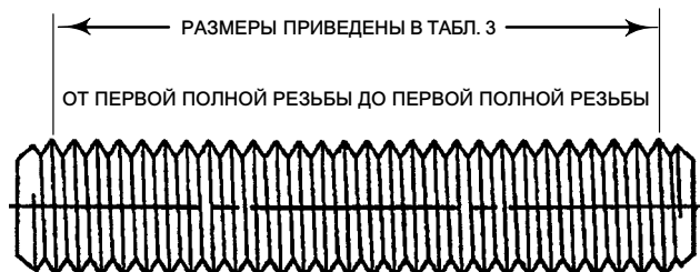
Рис. 2. Длина шпильки фланца для соединения предохранителя уплотнения
