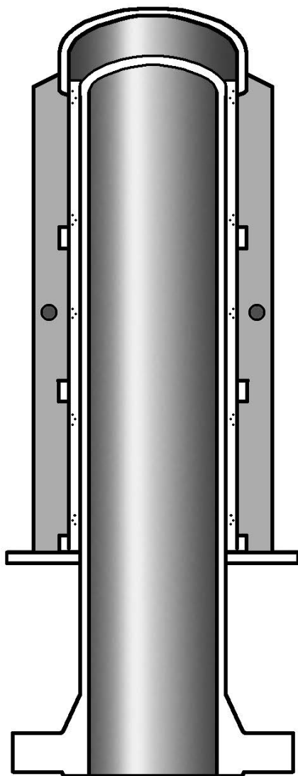
Figura 2. Diffusore di sfiato 6012 Fisher
