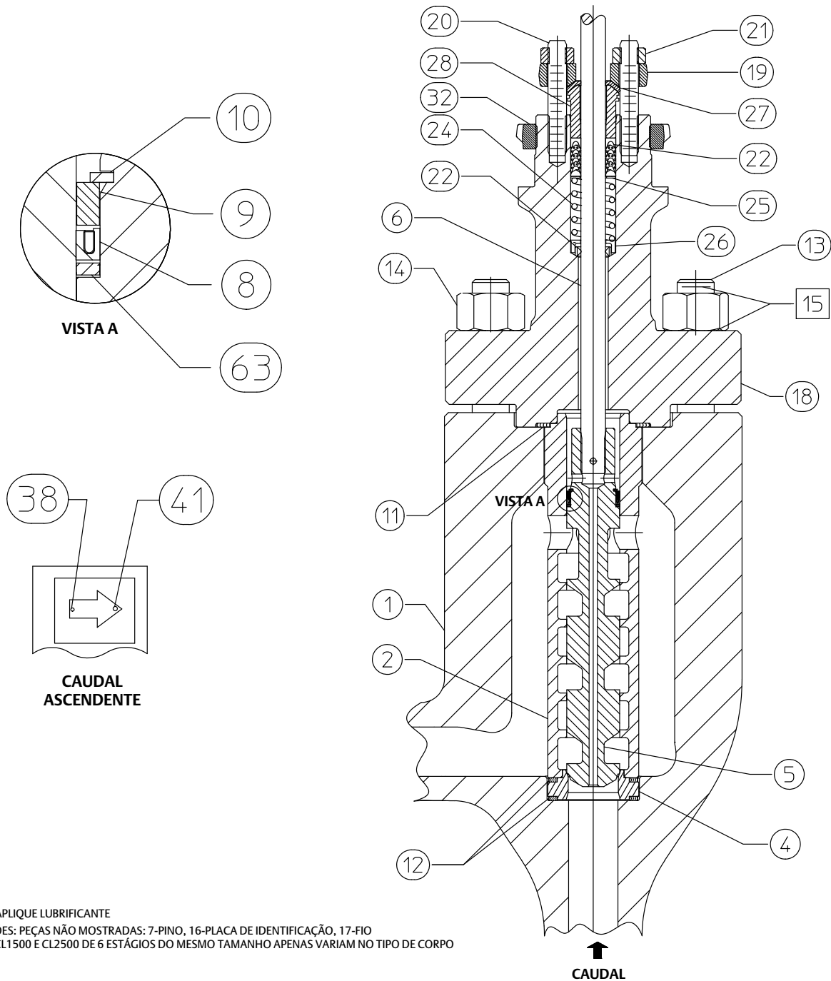
Figura 19. Conjunto de Válvula de Ângulo Fundida NotchFlo DST CL2500 de 6 Estágios (NPS 2 e 3) da Fisher
