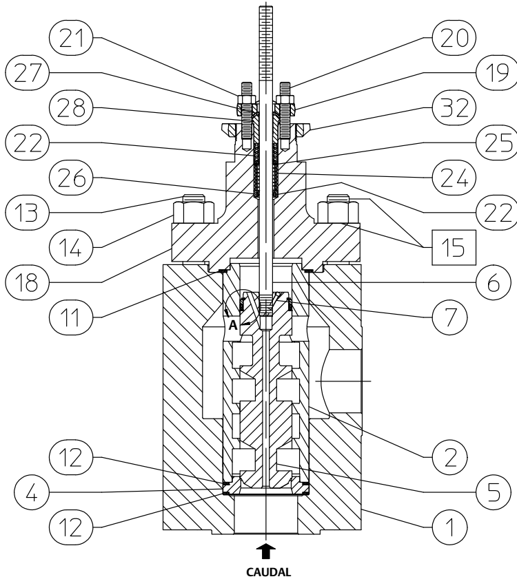
MOSTRADA NotchFlo DST CL1500 NPS 4, DE 4 ESTÁGIOS
