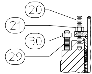
RESSALTO DA FORQUILHA DE 5 POL.
