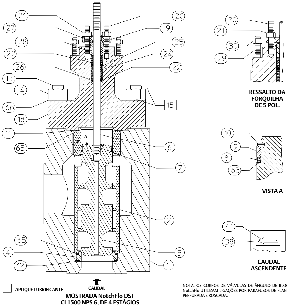
Figura 16. Conjunto de Válvula de Ângulo Equilibrada NotchFlo DST CL1500 ≥ NPS 6 da Fisher
