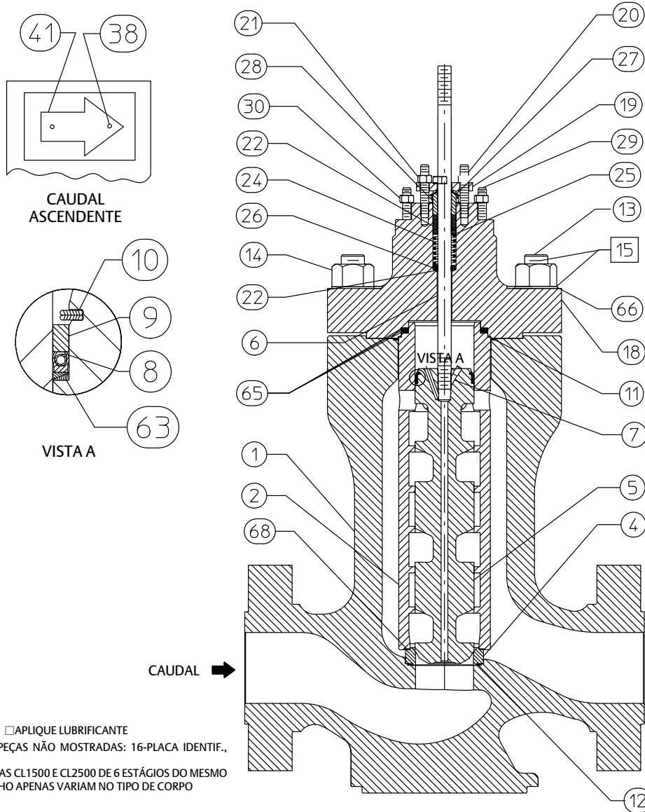
Figura 18. Conjunto de Válvula de Globo NotchFlo DST CL1500 e CL2500 de 6 Estágios (NPS 4 e 6) da Fisher
