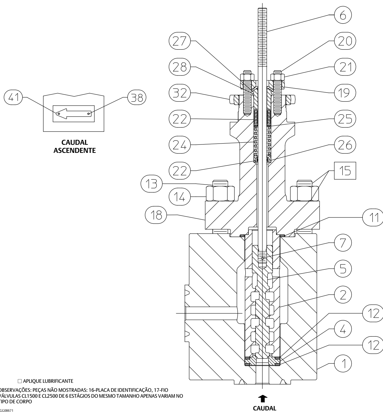
Figura 17. Conjunto de Válvula de Ângulo Não Equilibrada NotchFlo DST CL2500 de 6 Estágios (NPS 1) da Fisher
