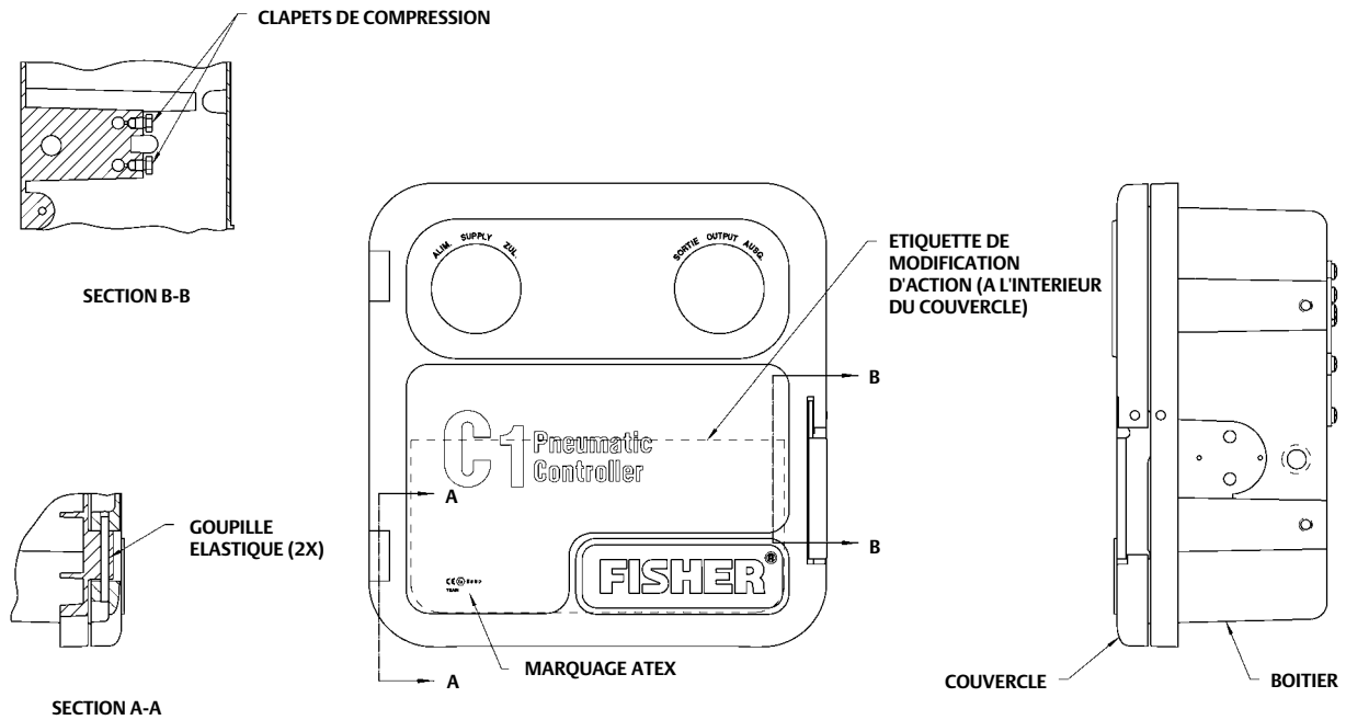
Figure 26. Vue frontale du boîtier et du couvercle
