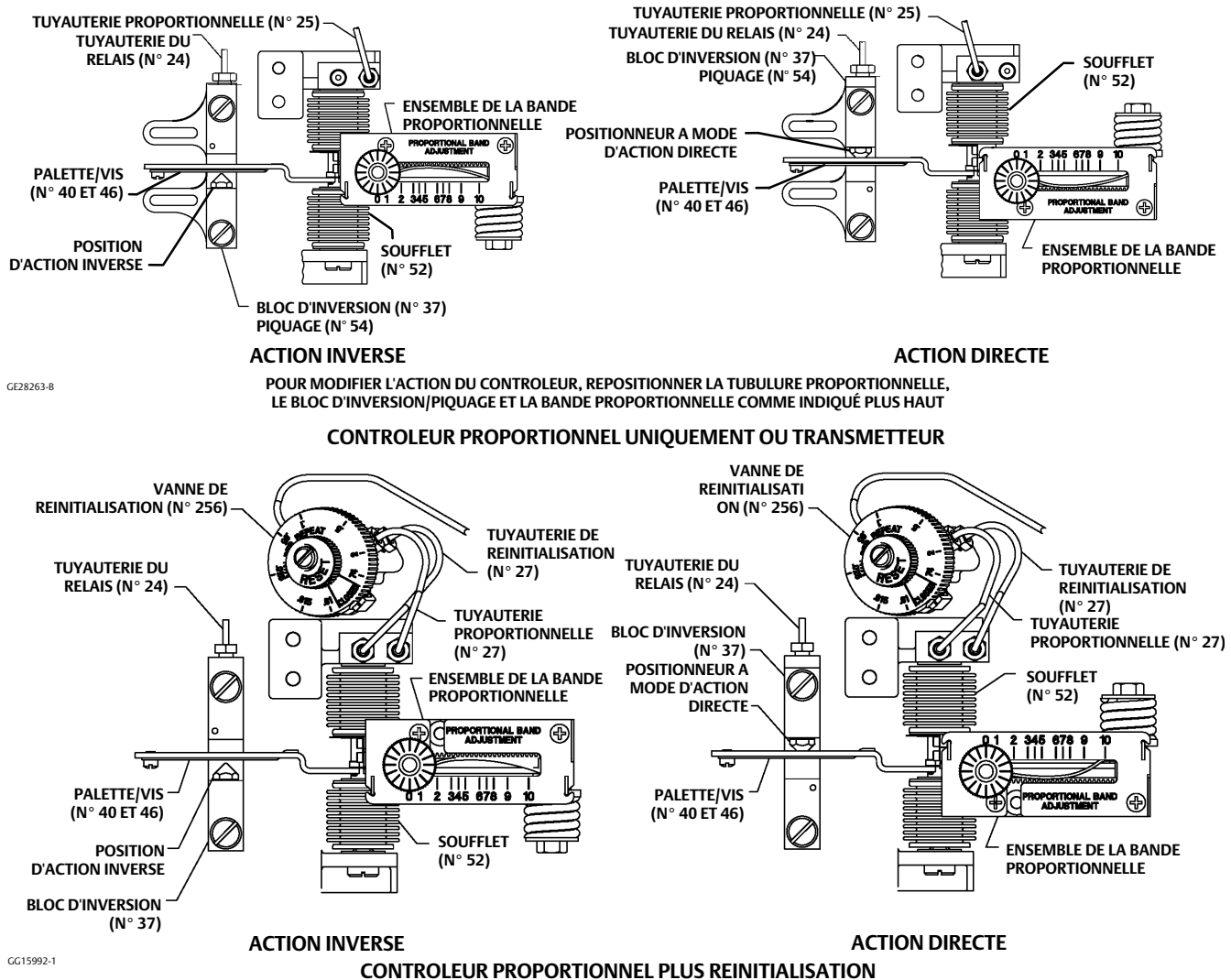
Figure 18. Raccordement de la tuyauterie à action directe/inverse pour les contrôleurs proportionnels ou pour le transmetteur
