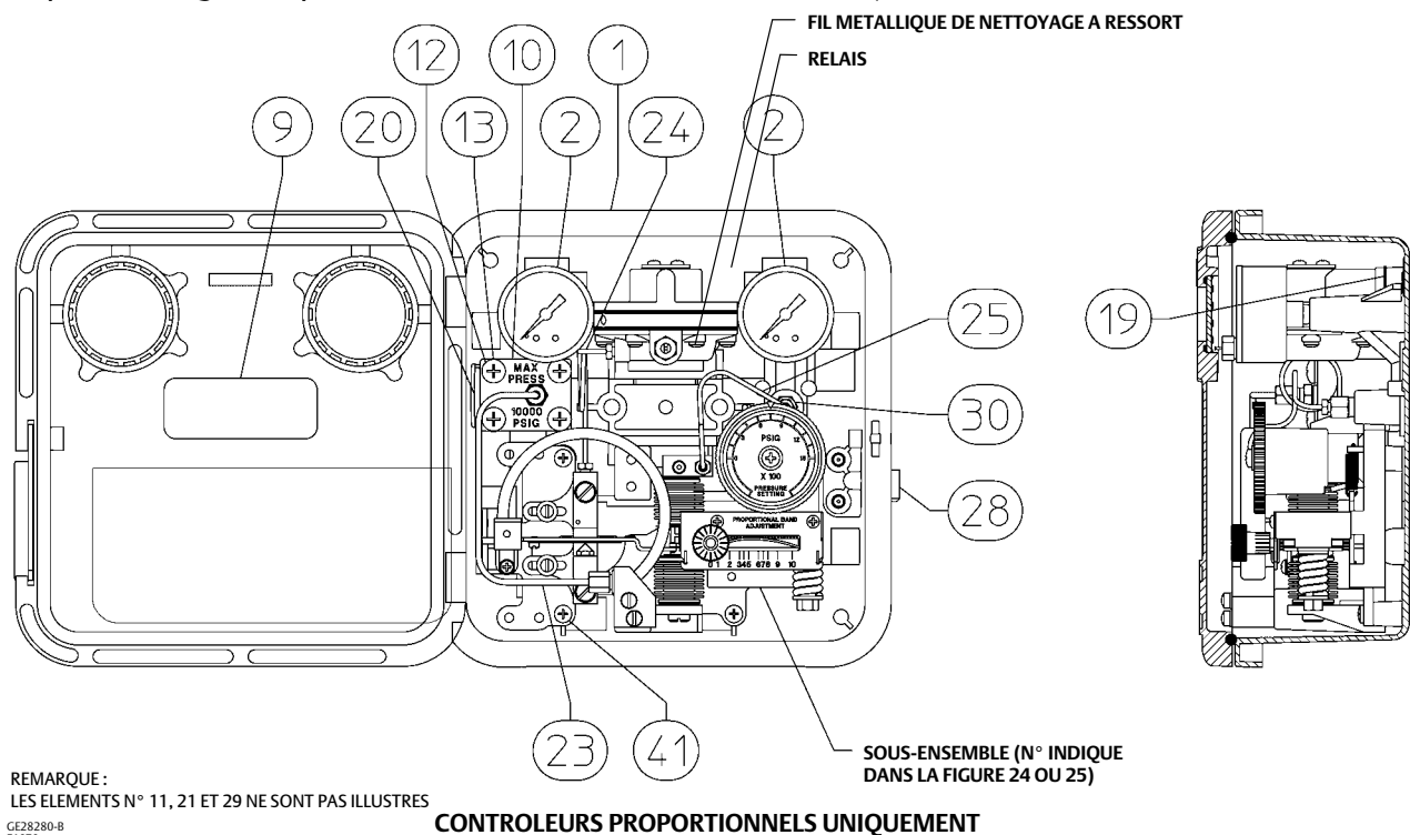
Figure 22. Ensemble C1 de Fisher à action inverse type (suite) (se reporter à la figure 26 pour la vue frontale du boîtier et du couvercle)
