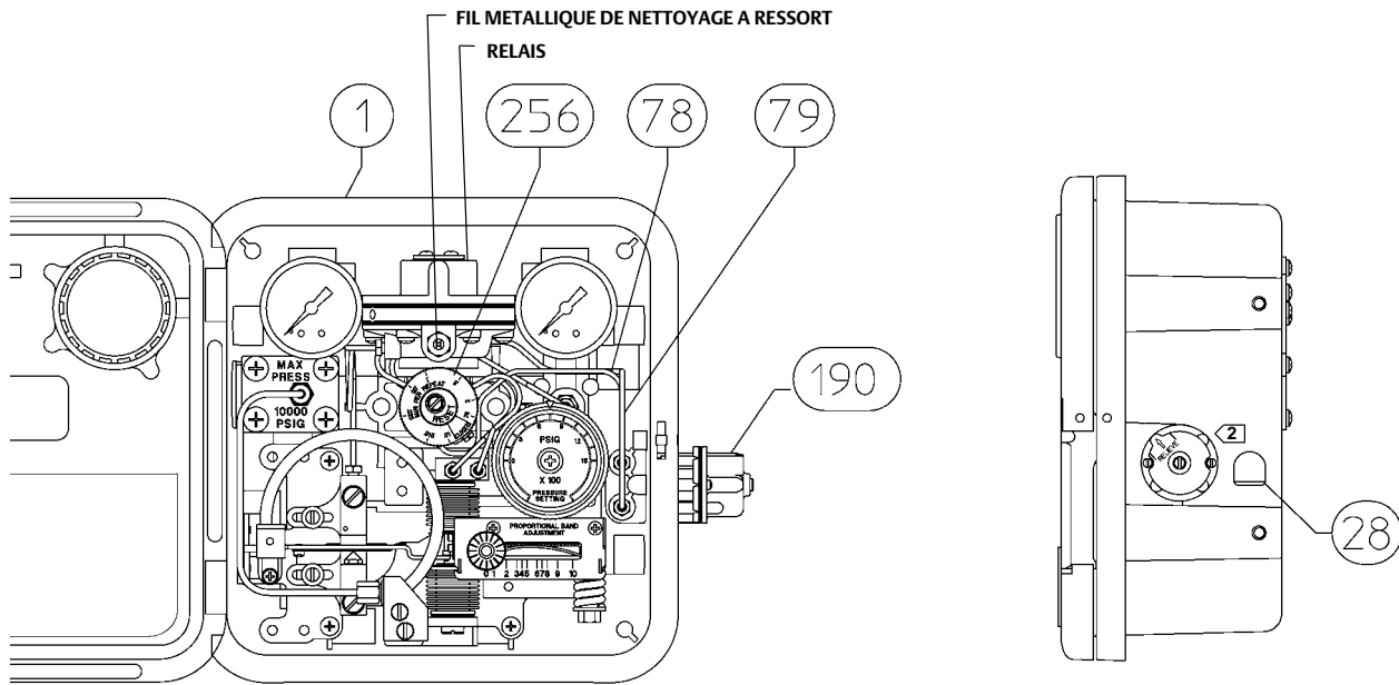
Figure 23. Ensemble C1 de Fisher à action inverse type Ensemble proportionnel plus réinitialisation (suite) (se reporter à la figure 26 pour la vue frontale du boîtier et du couvercle)
