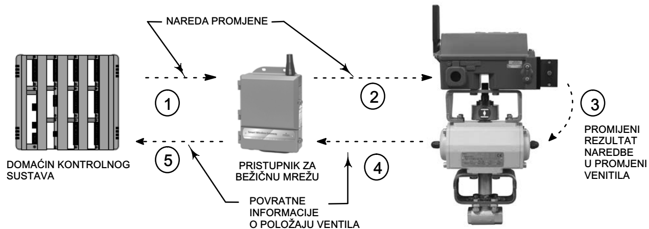
Slika 2. Kontrolni rad - bežični automatizirani ventil
