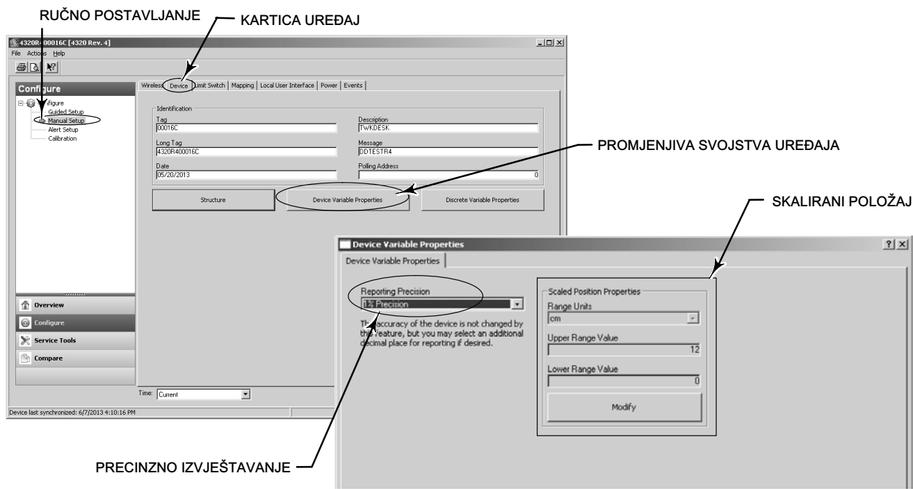
Slika 25. Promjenjiva svojstva uređaja
