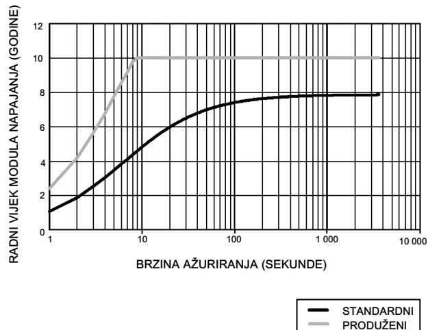
Slika 16. Učinak brzine ažuriranja na radni vijek modula napajanja; kontrola i nadzor uključivanja/isključivanja
