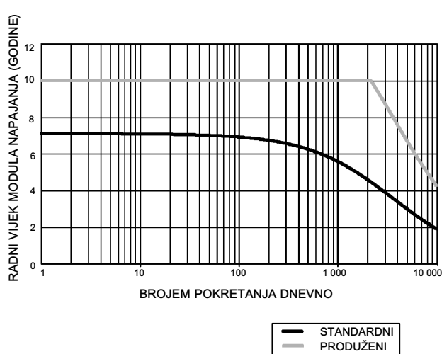
Slika 19. Učinak pokretanja na radni vijek modula napajanja; kontrola uključivanja/isključivanja
