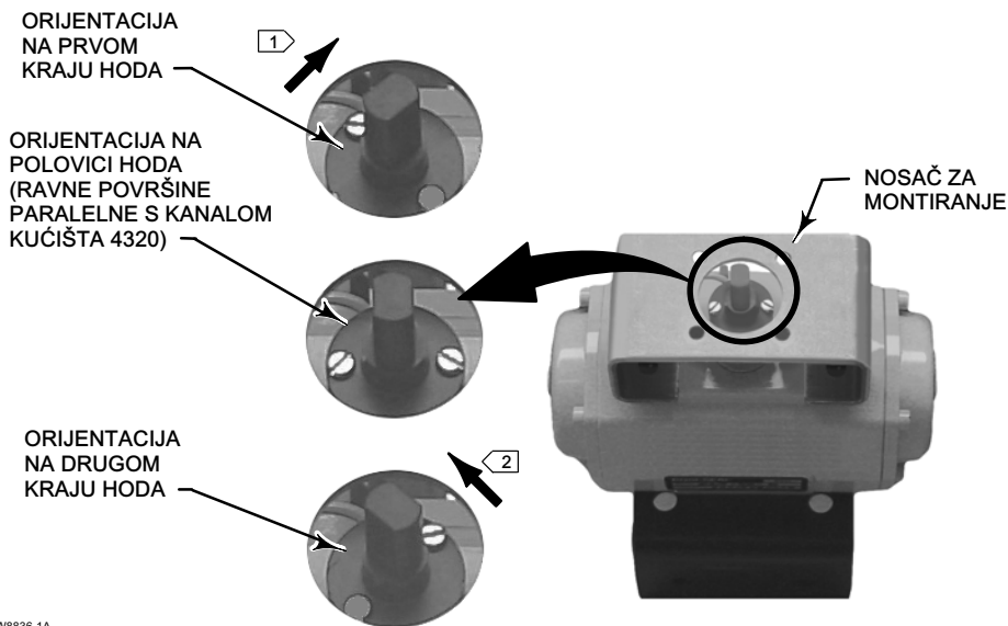
Slika 14. Orijentacija sklopa magneta
