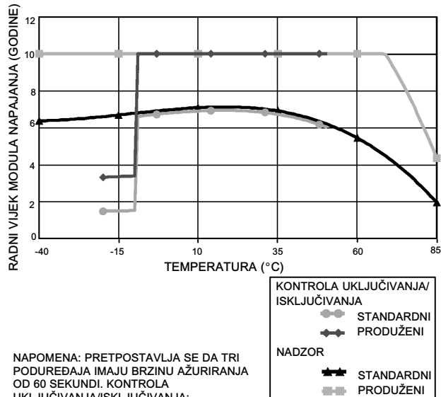
Slika 18. Učinak temperature na radni vijek modula napajanja; kontrola i nadzor uključivanja/isključivanja
