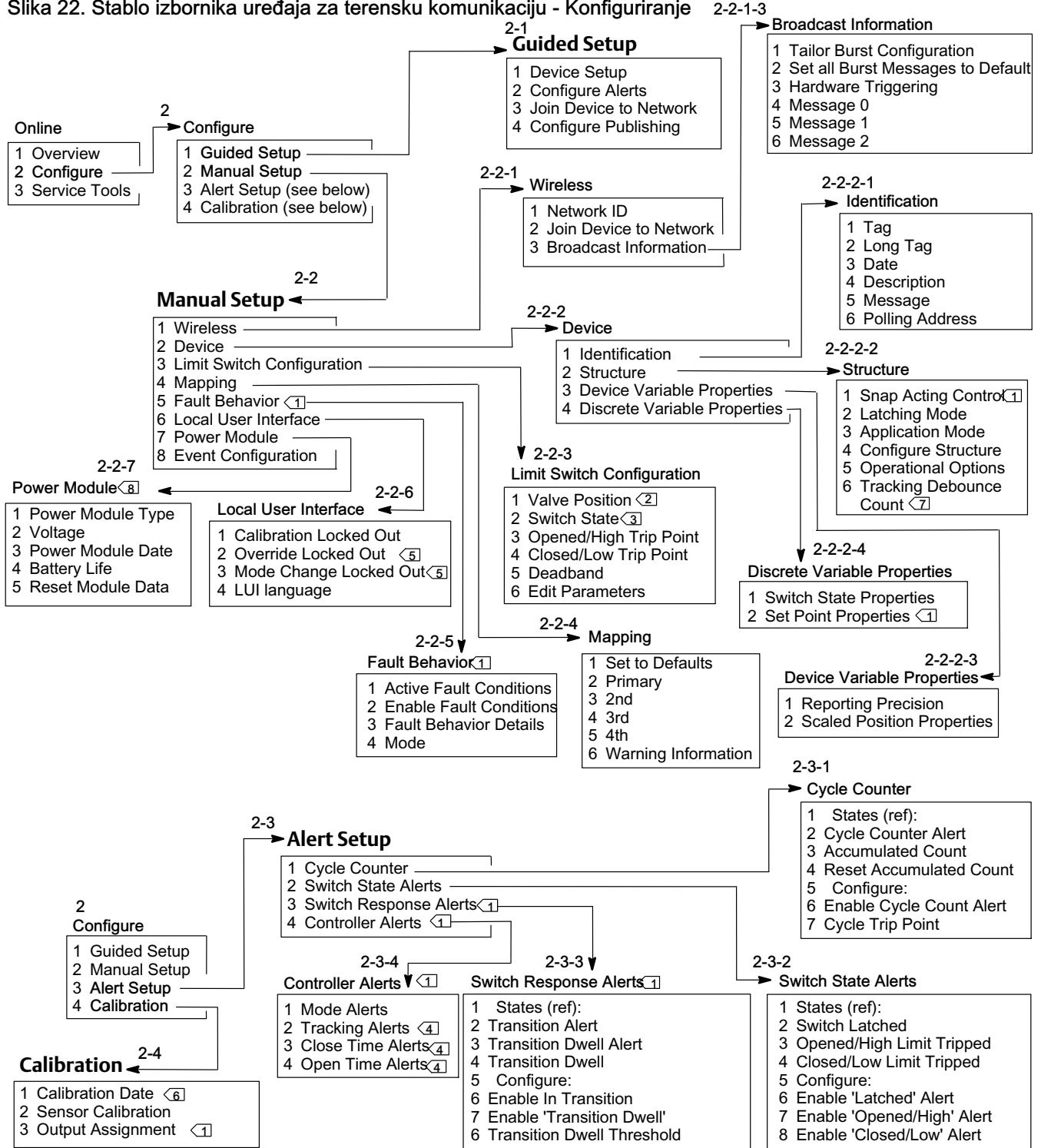
Slika 22. Stablo izbornika uređaja za terensku komunikaciju - Konfiguriranje
