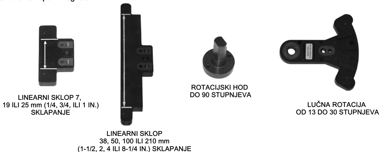
Slika 9. Sklopovi magneta
