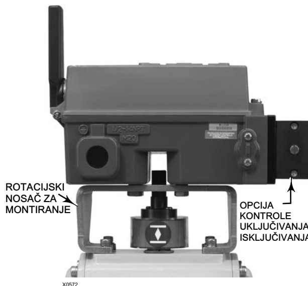
Slika 12. Za pokretače s rotacijskom osovinom (klasičan nosač za montiranje)
