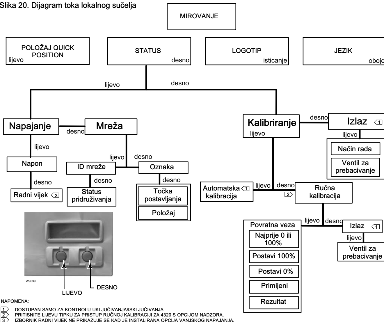
Slika 20. Dijagram toka lokalnog sučelja
