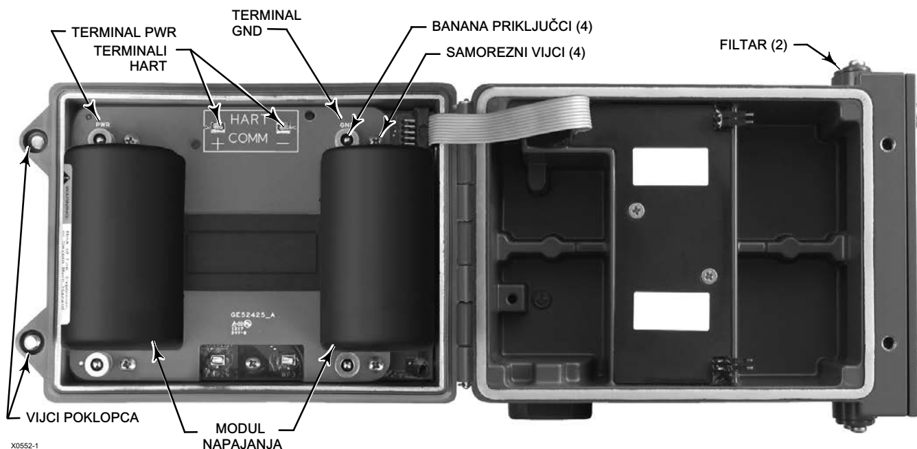
Slika 5. Fisher 4320 s modulima baterijskog izvora napajanja
