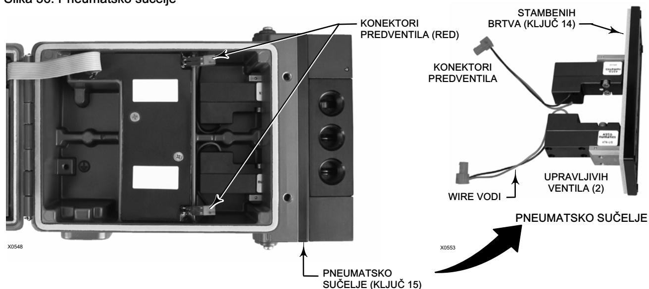
Slika 36. Pneumatsko sučelje
