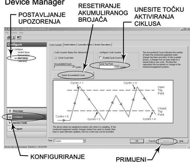
Slika 26. Resetiranje akumuliranog brojača ciklusa u programima AMS Wireless Configurator i AMS Device Manager
