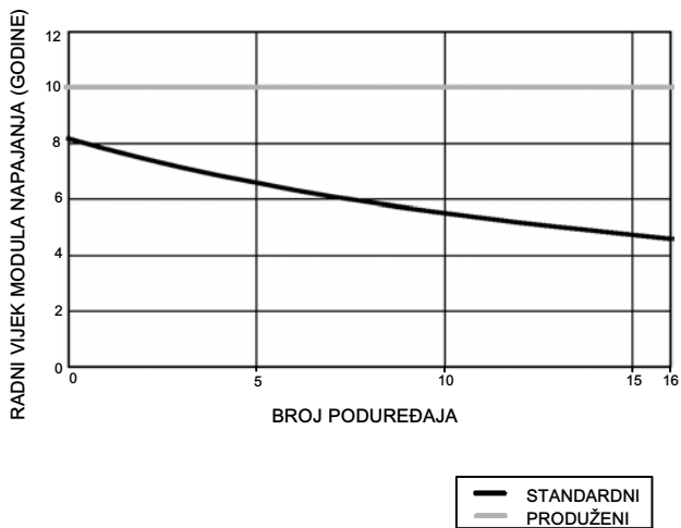
Slika 17. Broj poduređaja utječe na radni vijek modula napajanja, nadzor
