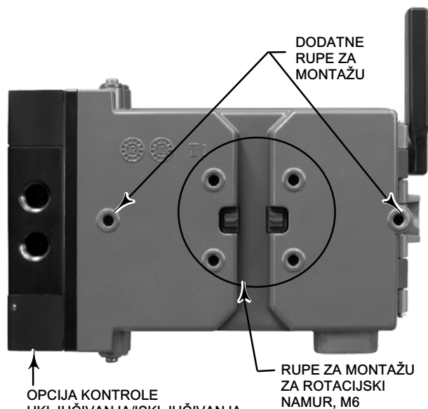
Slika 11. Kućište i montiranje linearnog i pokretača s četvrtinom okreta
