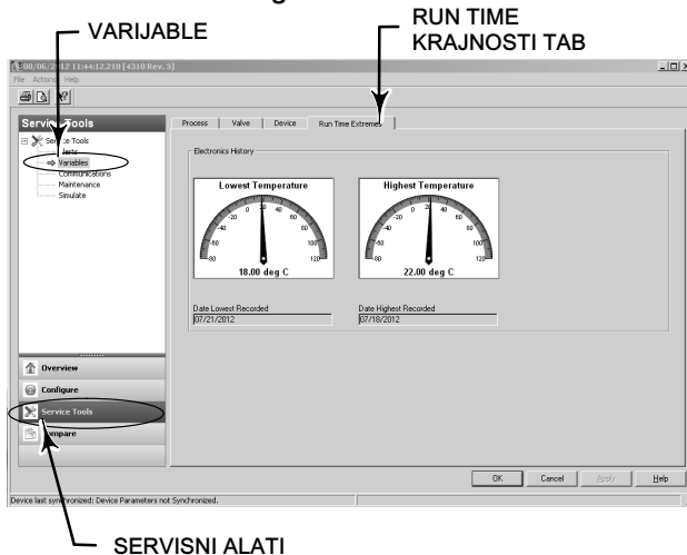
Slika 31. Prikazivanje radnih ekstrema u programima AMS Wireless Configurator i AMS Device Manager
