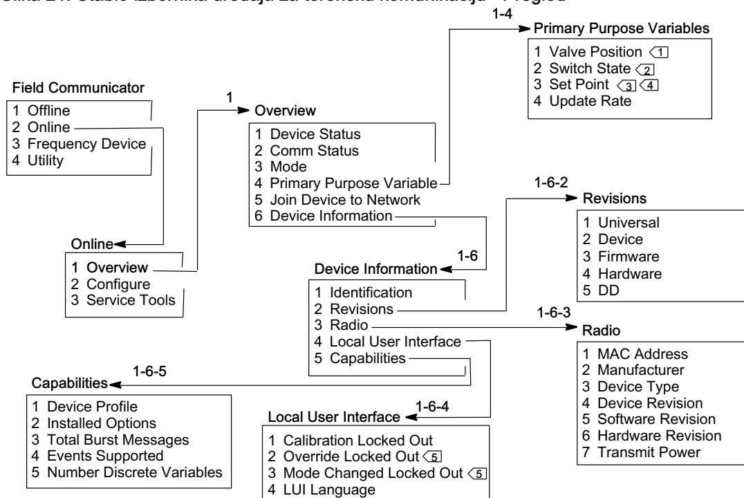
Slika 21. Stablo izbornika uređaja za terensku komunikaciju - Pregled
