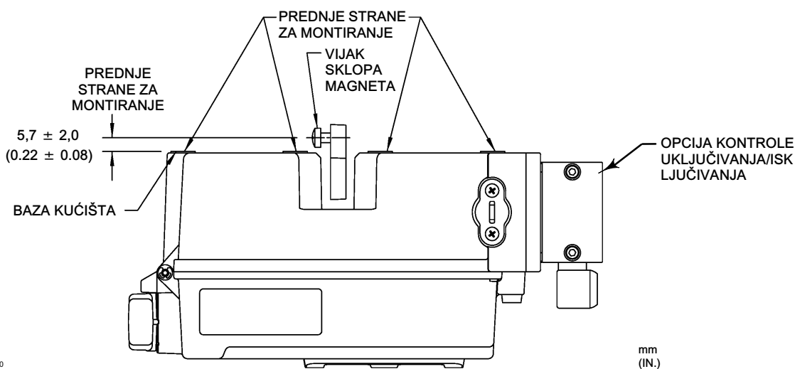
Slika 10. Montiranje - sklop magneta s kliznim vretenom
