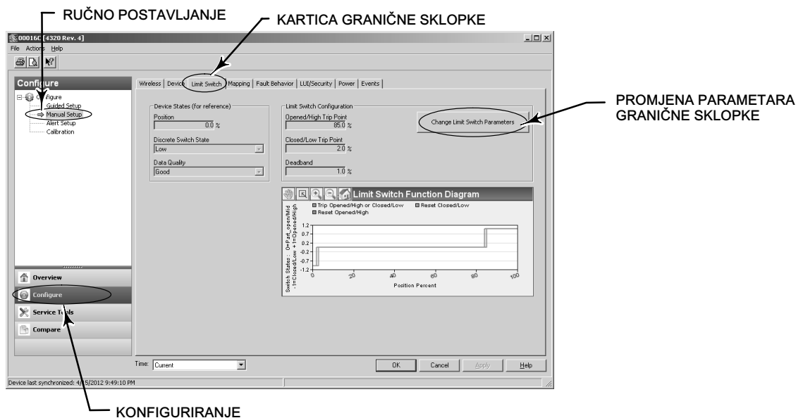
Slika 24. Postavljanje točaka aktiviranja u programima AMS Wireless Configurator i AMS Device Manager
