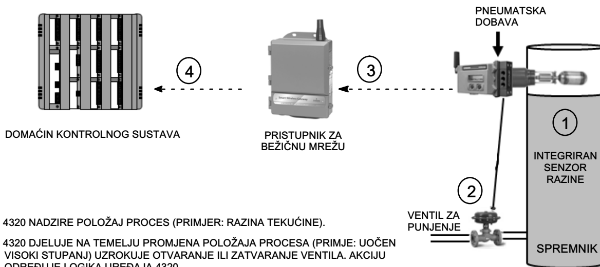
Slika 3. Kontrolni rad - kontrola zatvaranja
