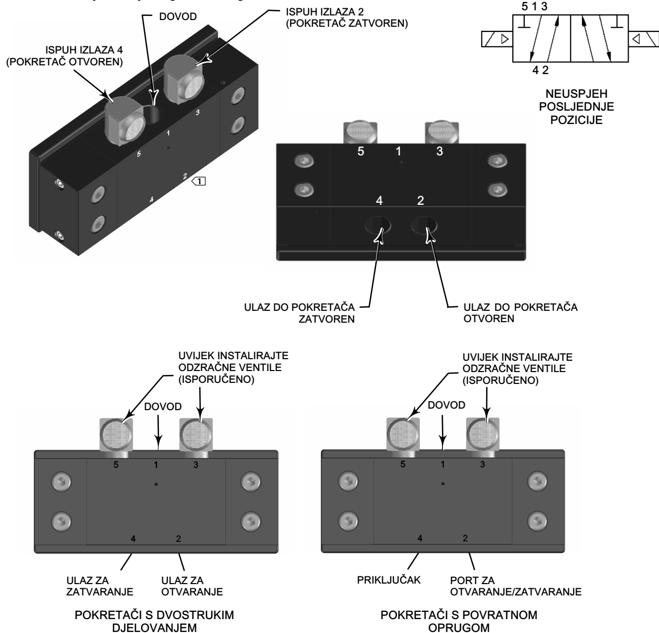
Slika 15. Instalacija 4-smjernog razvodnog ventila
