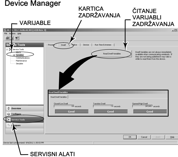
Slika 29. Prikazivanje zadržavanja i prijelaza u uređajima AMS Wireless Configurator i AMS Device Manager
