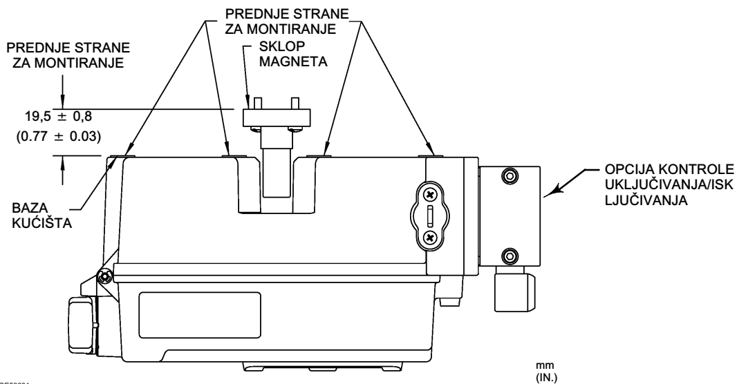
Slika 13. Montiranje - Sklop rotacijskog magneta
