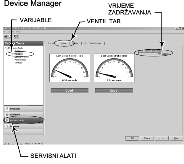
Slika 28. Pregledava zadnja otvoriti i zatvoriti vrijeme u AMS Wireless Configurator i AMS Device Manager
