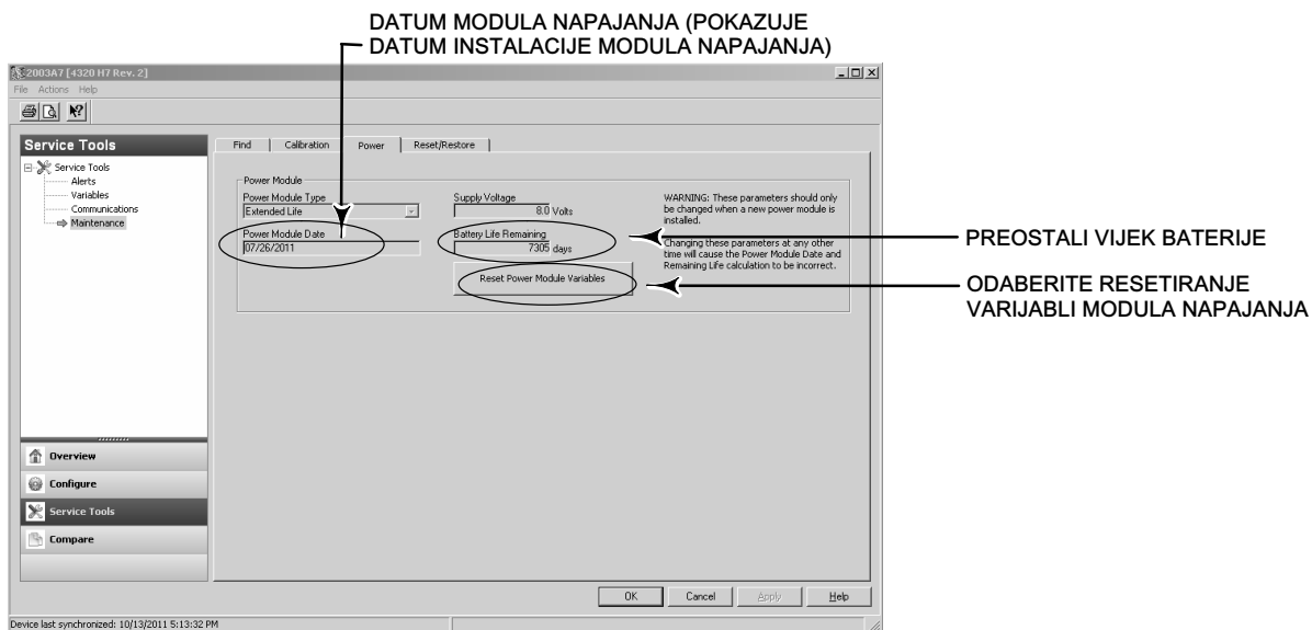
Slika 34. Resetiranje varijabli modula napajanja
