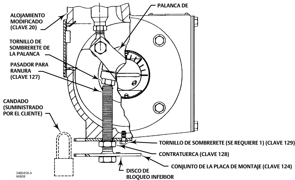
Figura 6. Mecanismo de bloqueo del actuador
