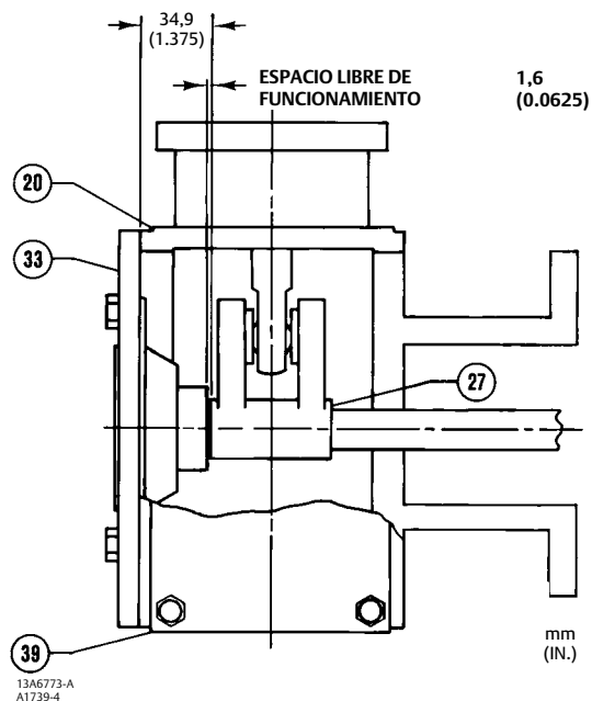
Figura 4. Espacio libre de funcionamiento de la palanca
