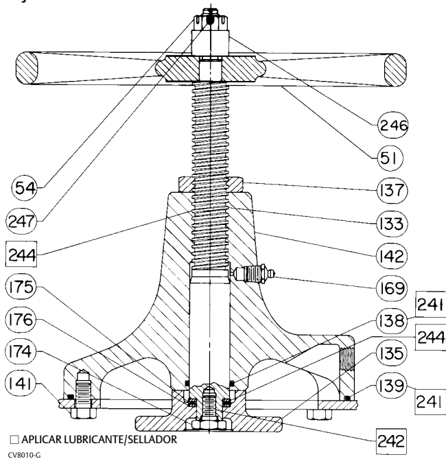
Figura 9. Conjuntos de volante
