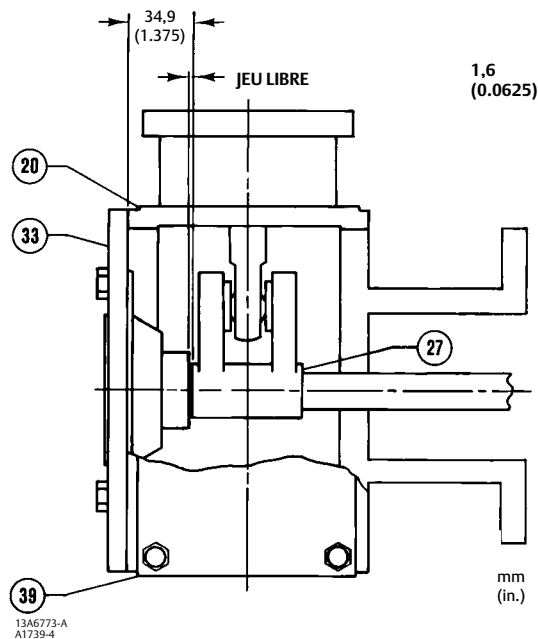
Figure 4. Jeu libre du levier
