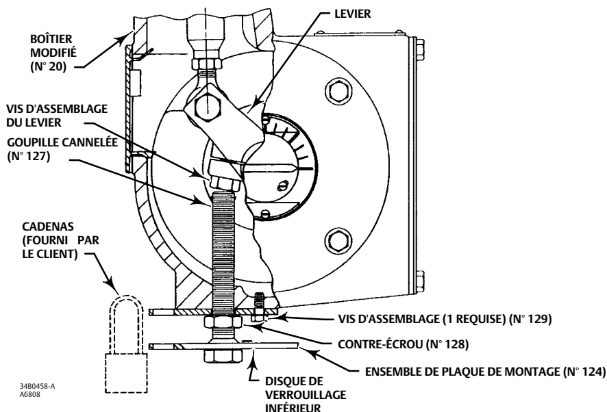
Figure 6. Mécanisme de verrouillage de l'actionneur
