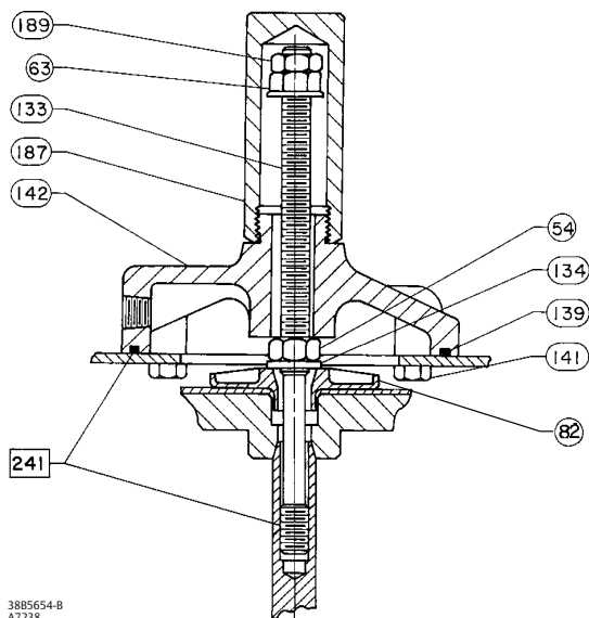
Figure 11. Butée de course basse ajustable
