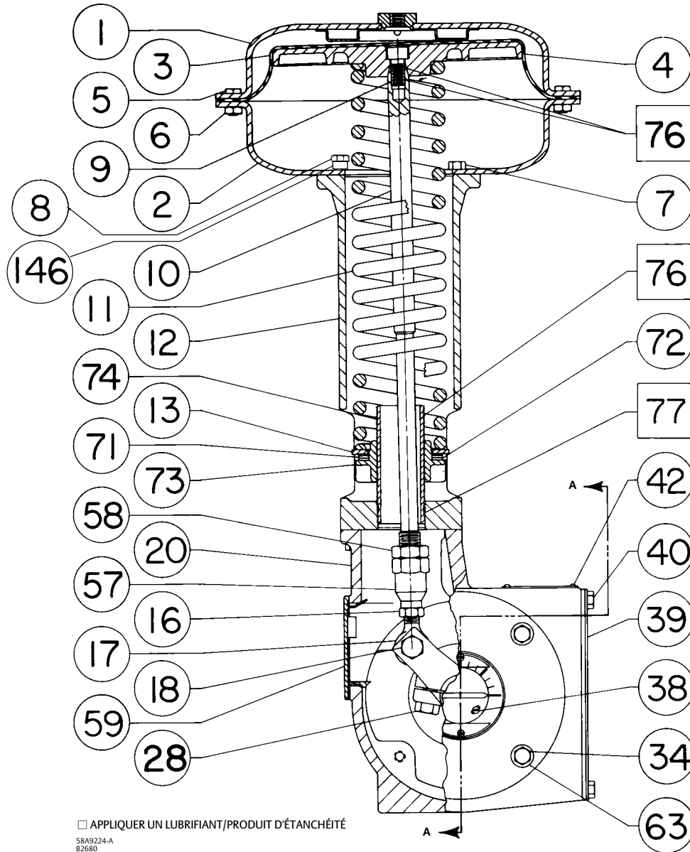
Figure 8. Actionneur 1052 typique
