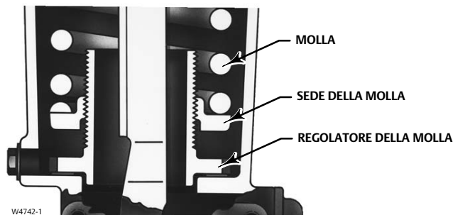
Figura 2. Sede della molla regolabile nell'attuatore tipico 1052
