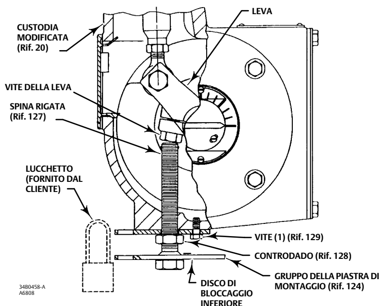
Figura 6. Meccanismo di bloccaggio dell'attuatore
