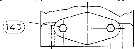
Figura 7. Gruppo dello sfiato a montaggio su staffa
