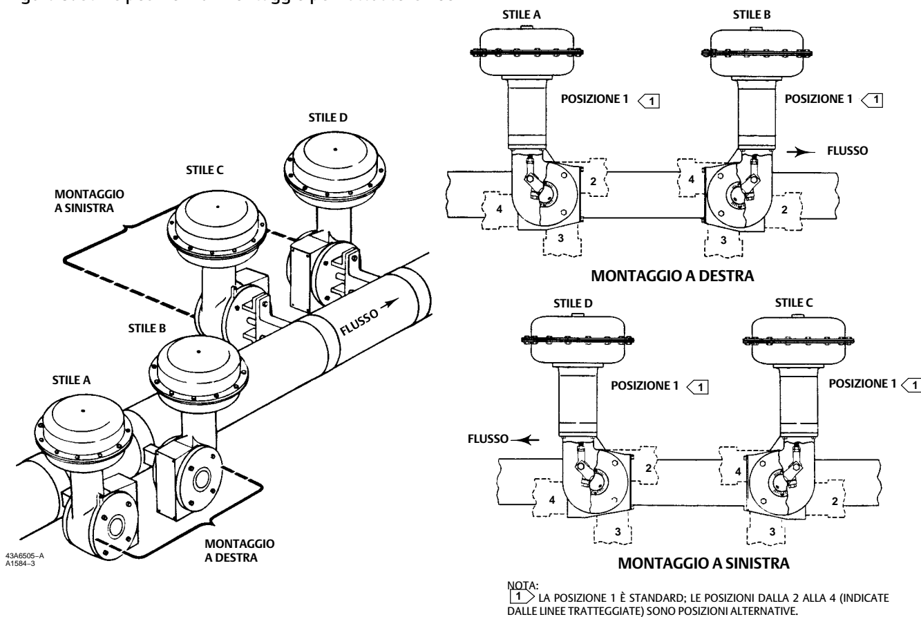
Figura 3. Stili e posizioni di montaggio per l'attuatore 1052
