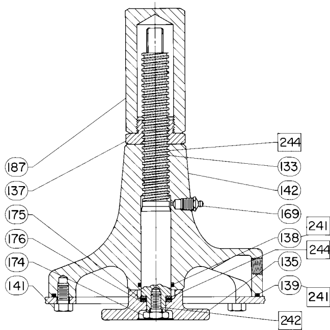
Figura 10. Fermi corsa in alto regolabili
