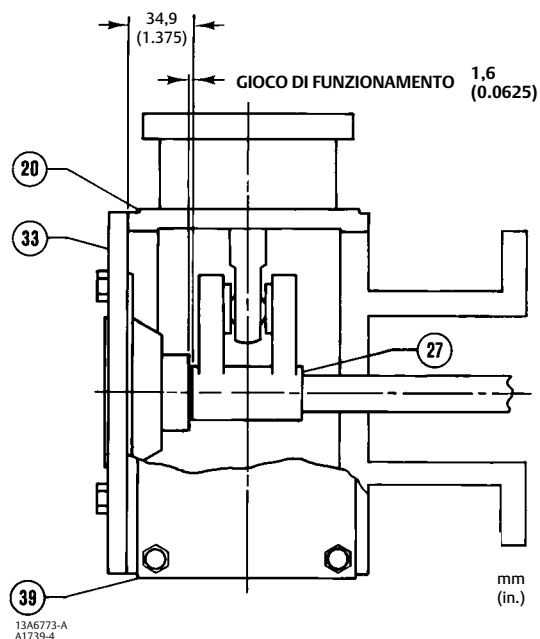
Figura 4. Gioco di funzionamento della leva
