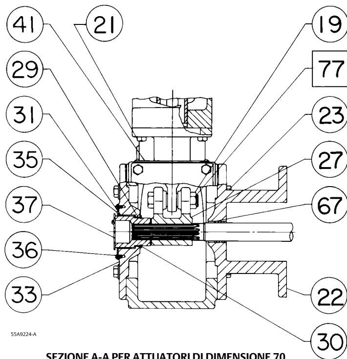
Figura 8. Gruppo 1052 tipico (segue)
