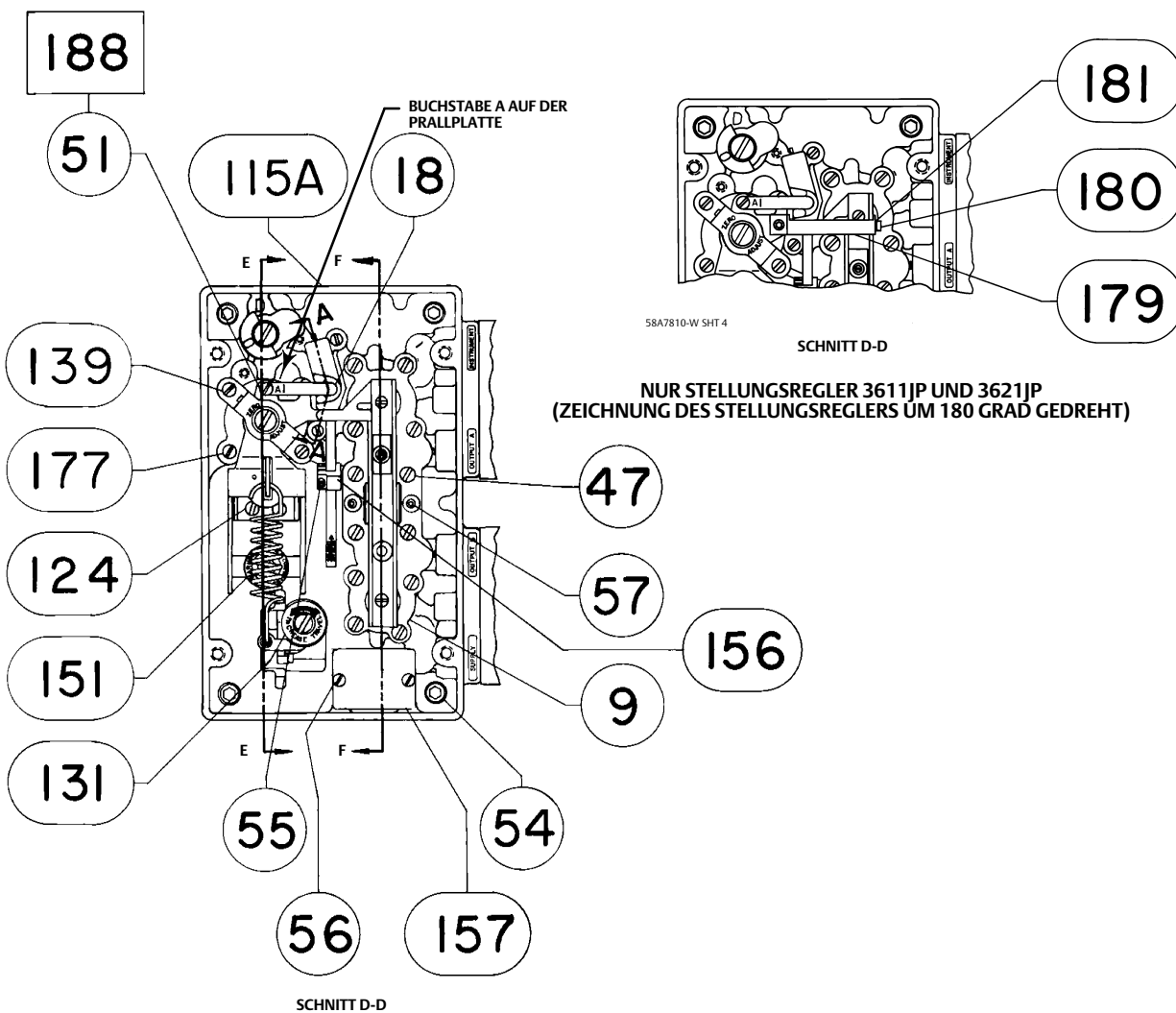
Abbildung 26. Stellungsregler
