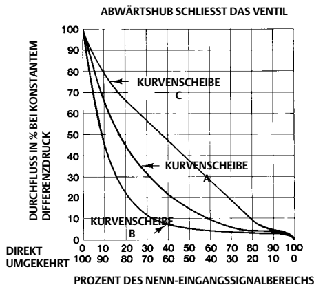
Abbildung 19. Durchflusskennlinien mit verschiedenen Kurvenscheiben bei gleichprozentiger Ventilkennlinie und mit Abwärtshub schließendem Ventil
