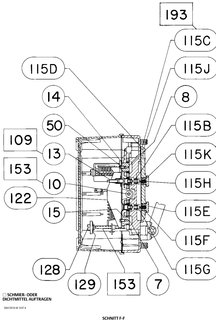
Abbildung 26. Stellungsregler (Fortsetzung)
