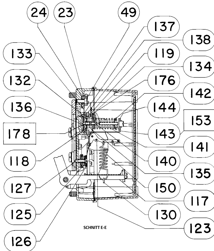
Abbildung 26. Stellungsregler (Fortsetzung)
