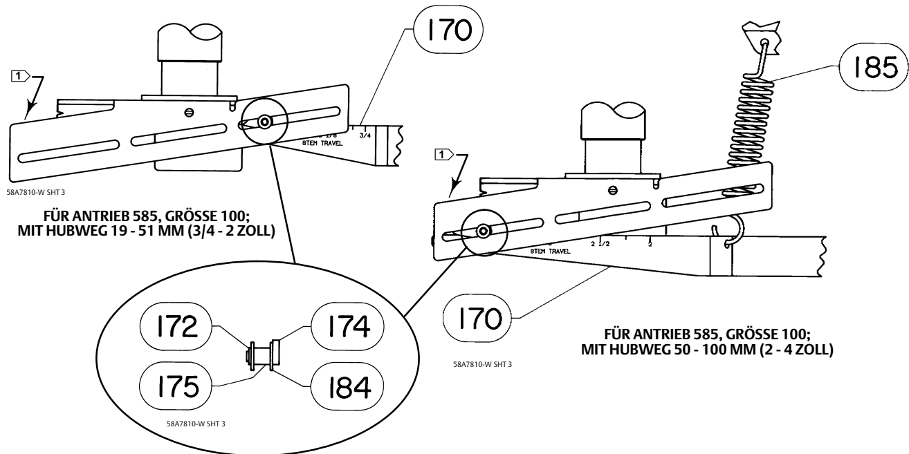
Abbildung 30. Rückführsysteme für Fisher Stellungsregler 3611JP und 3621JP
