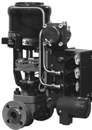
Abbildung 2. Fisher Stellungsregler 3621JP mit Antrieb 585C
