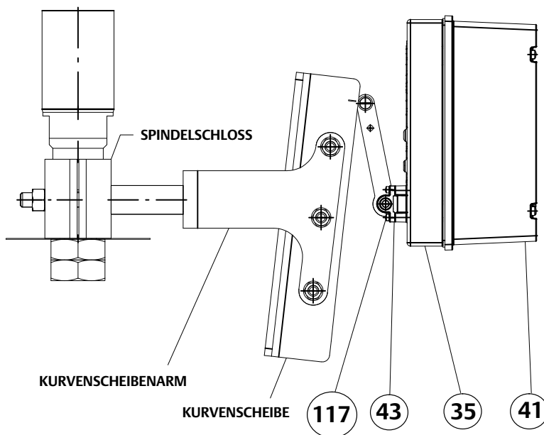
STELLUNGSREGLER 3610JP UND 3620JP FÜR 585C GRÖSSE 60 UND DARÜBER WEITERE INFORMATIONEN ZU ANDEREN STELLUNGSREGLERN FINDEN SIE IN DER SCHNITTZEICHNUNG DES JEWEILIGEN MONTAGESATZES.
