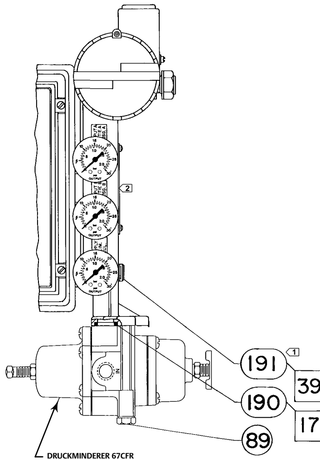
Abbildung 28. Fisher Stellungsregler 3620J mit integriert montiertem Druckminderer
