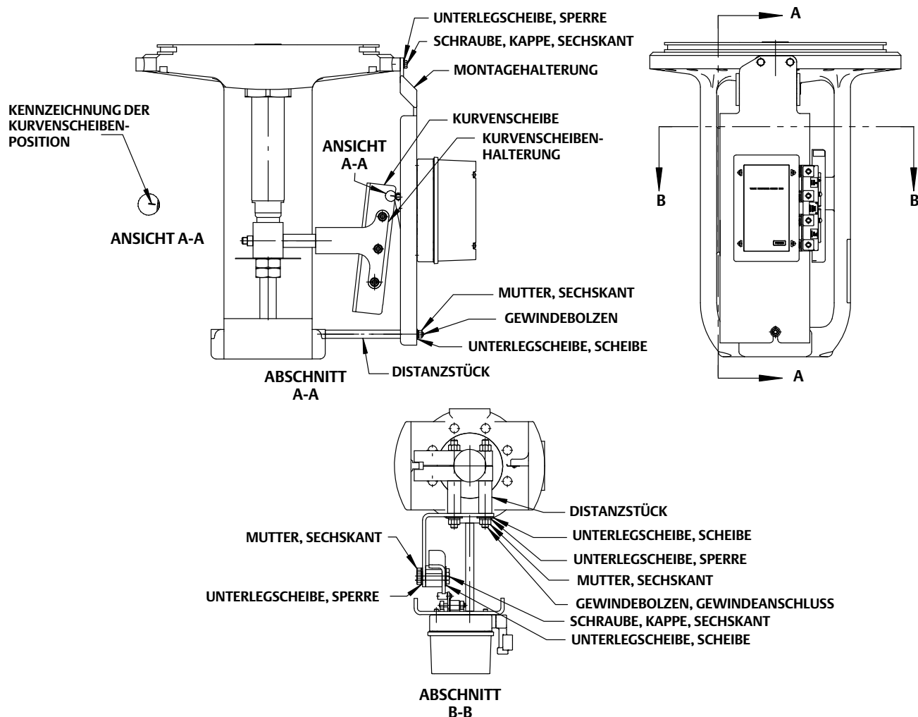
Abbildung 7. Typischer Anbau von Fisher Stellungsreglern 3610JP und 3620JP an Hubantrieben mit langem Hub
