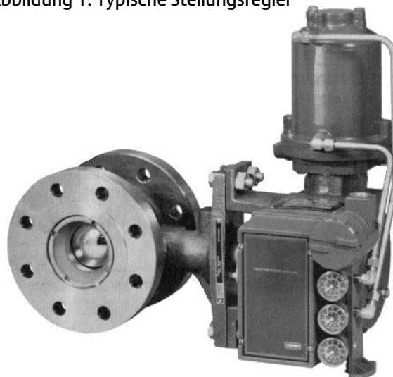
W4920-1 STELLUNGSREGLER 3620JP MIT FISHER ANTRIEB 1061 UND VENTILTYP V500
