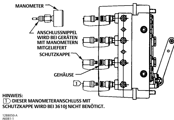
Abbildung 10. Anschlüsse für das FlowScanner™ Diagnosesystem an den Fisher Stellungsreglern 3610J und 3610JP
