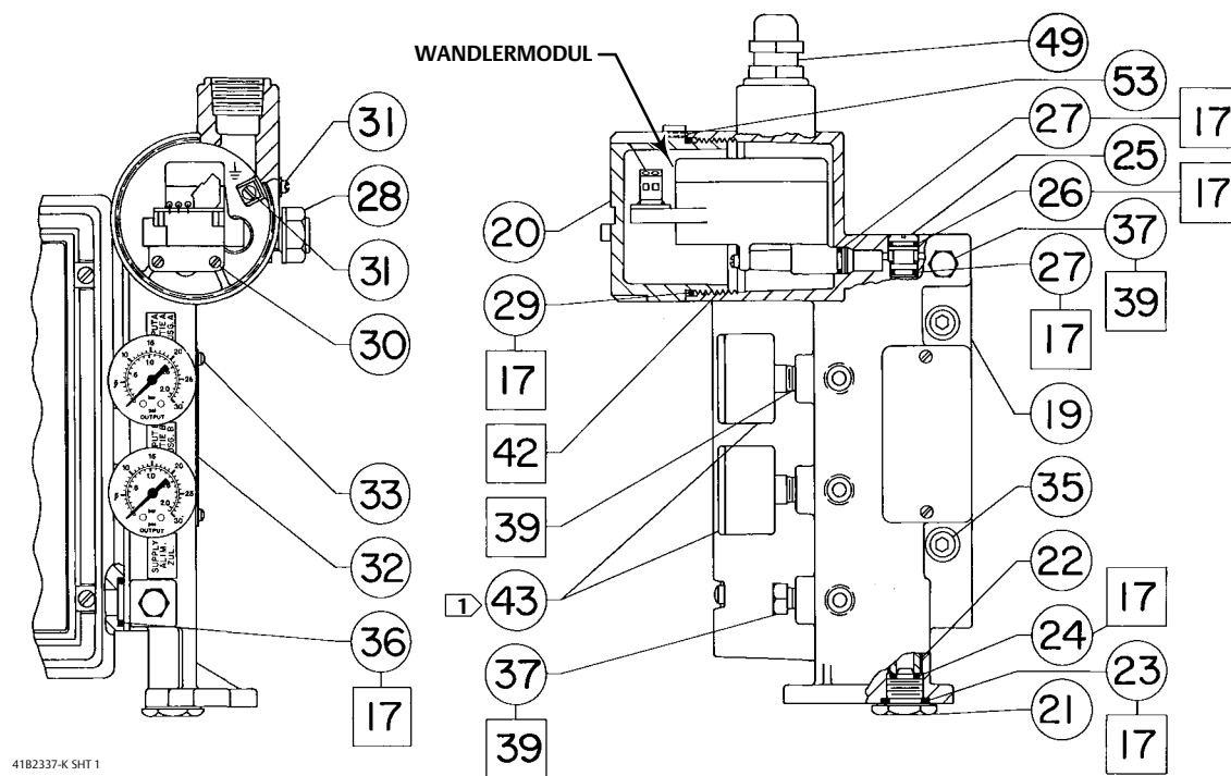
Abbildung 31. Fisher Elektropneumatischer Wandler 3622
