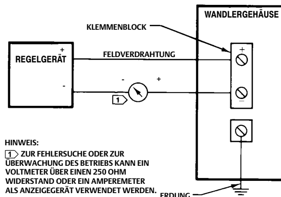
Abbildung 13. Typisches Feldverdrahtungsschema
