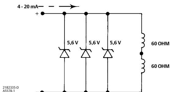
Abbildung 12. Äquivalenter Kreis des Fisher Wandlers 3622
