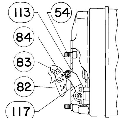
Abbildung 29. Rückführsysteme für die Fisher Stellungsregler 3610J, 3610JP, 3620J und 3620JP
