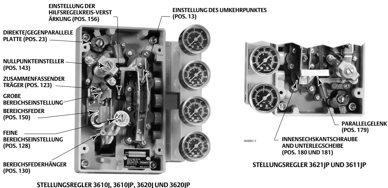
Abbildung 14. Anpassungen der Kalibrierung
