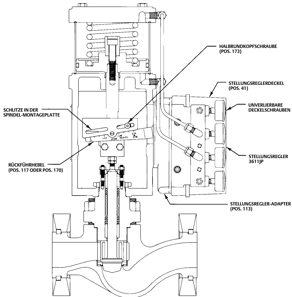
Abbildung 4. Typischer Anbau von Fisher Stellungsreglern 3611JP und 3621JP an Antriebe 585
