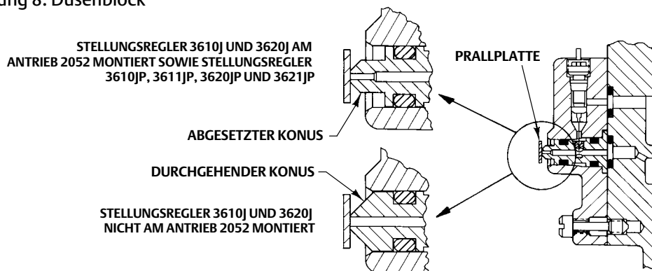
Abbildung 8. Düsenblock
