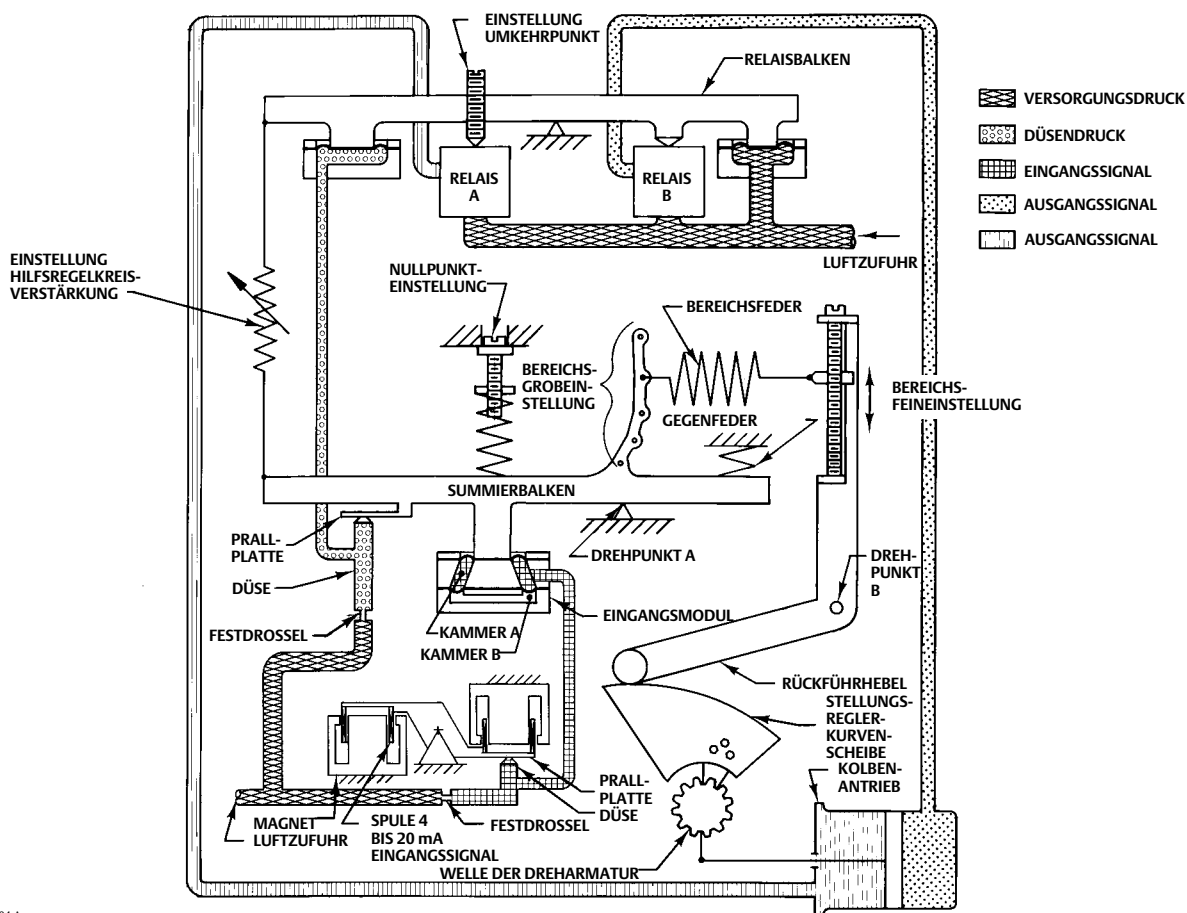
Abbildung 24. Funktionsschema des Fisher Stellungsreglers 3620JP
