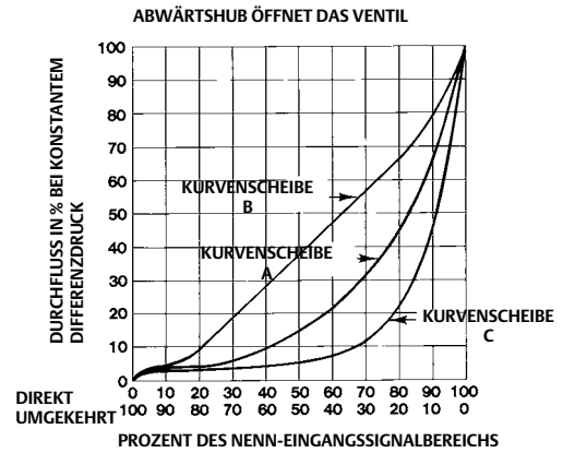
Abbildung 18. Durchflusskennlinien mit verschiedenen Kurvenscheiben bei gleichprozentiger Ventilkennlinie und mit Abwärtshub öffnendem Ventil
