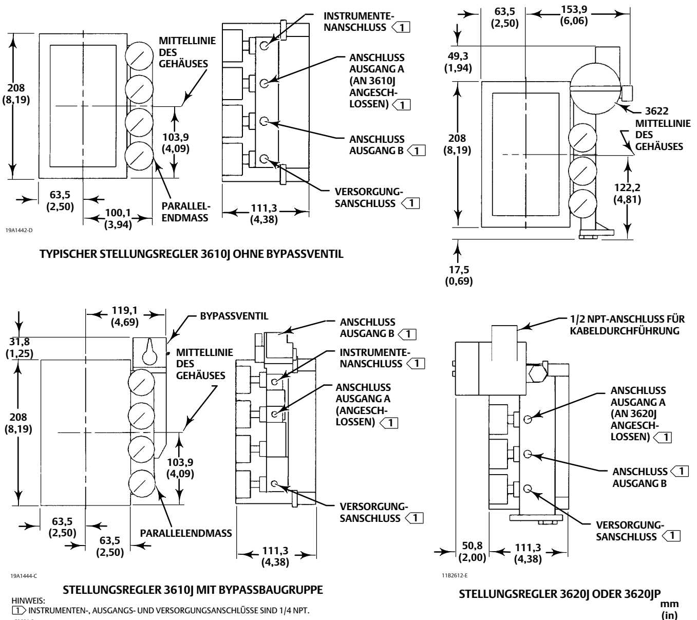
Abbildung 9. Typische Montageabmessungen und Anschlüsse
