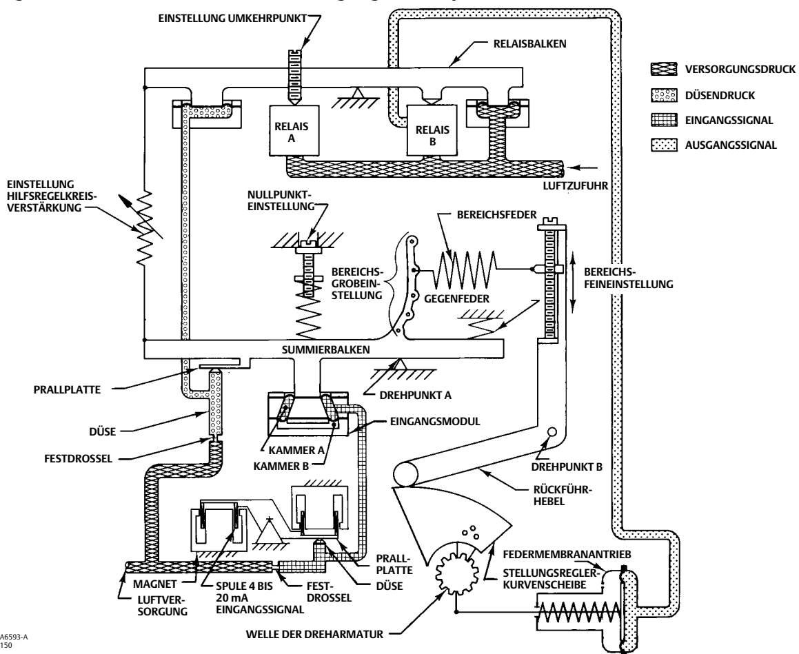
Abbildung 23. Funktionsschema des Fisher Stellungsreglers 3620J
