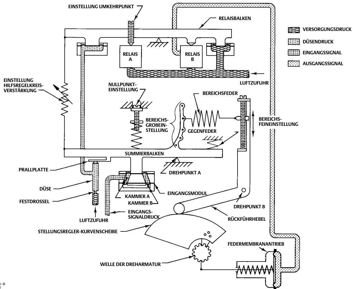
Abbildung 20. Funktionsschema des Fisher Stellungsreglers 3610J
