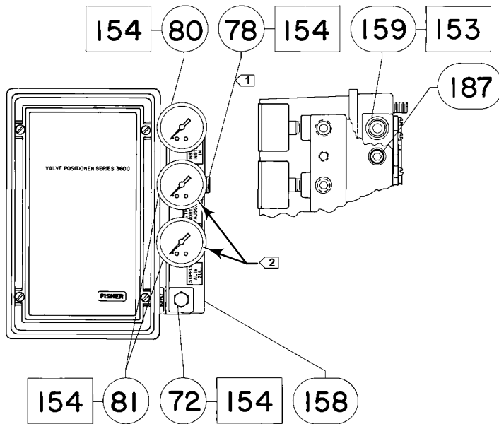
Abbildung 27. Manometerblock und Bypassventil
