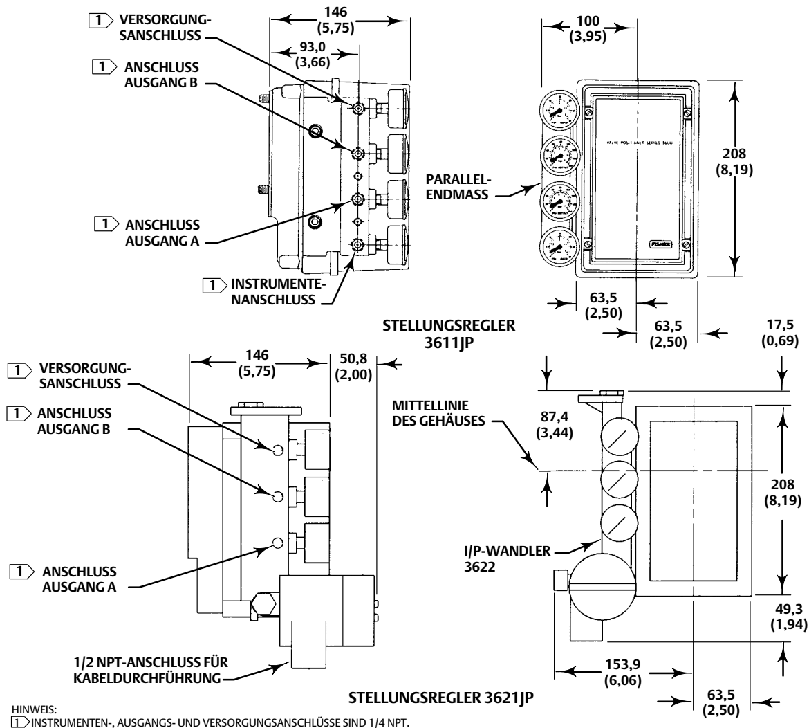
Abbildung 9. Typische Montageabmessungen und Anschlüsse (Fortsetzung)
