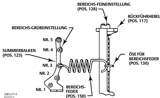
Abbildung 16. Einstellung des Bereichs
