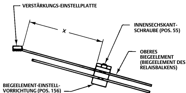
Abbildung 15. Einstellung der Hilfsregelkreis-Verstärkung
