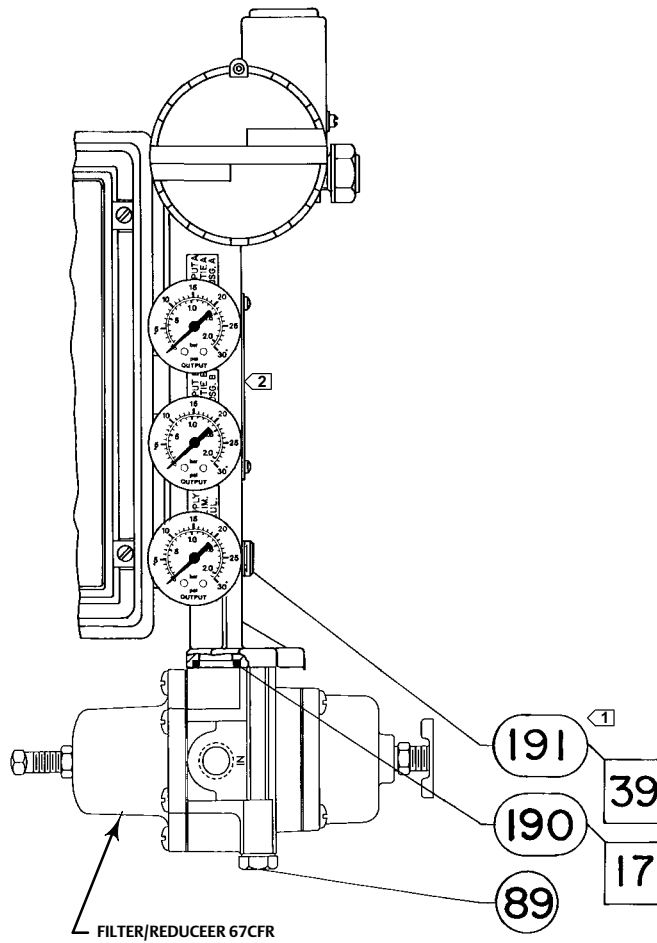
Afbeelding 28. Fisher 3620J-klepstandsteller met integraal gemonteerde filter/reduceer
