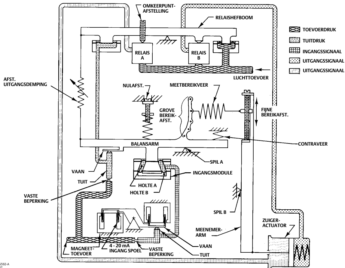
Afbeelding 25. Schema van Fisher 3621JP-klepstandsteller
