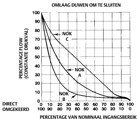
Afbeelding 19. Flowkarakteristieken voor de diverse nokken wanneer gebruikt met klep met gelijk-percentegekarakteristiek die omlaag wordt gedruwd om te sluiten
