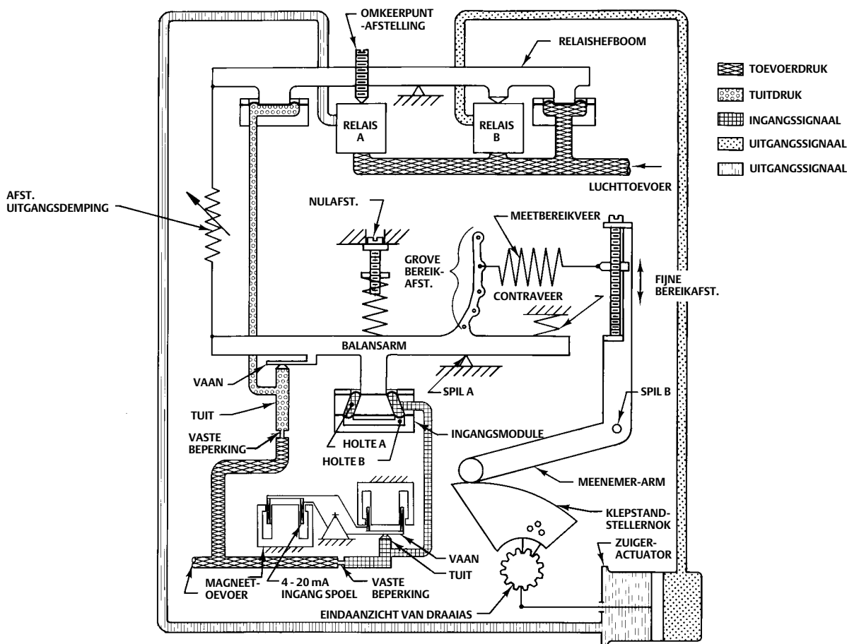
Afbeelding 24. Schema van Fisher 3620JP-klepstandsteller
