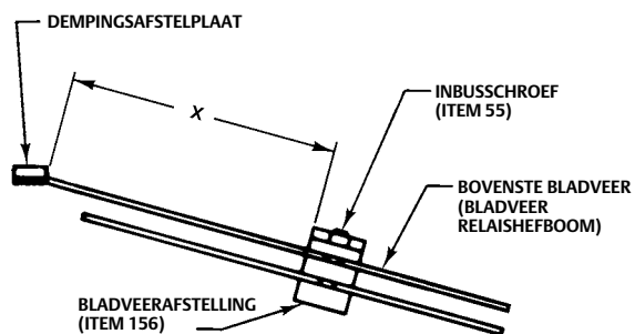
Afbeelding 15. Afstellen van de uitgangsdemping
