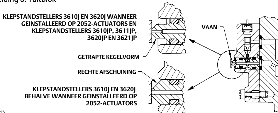
Afbeelding 8. Tuitblok
