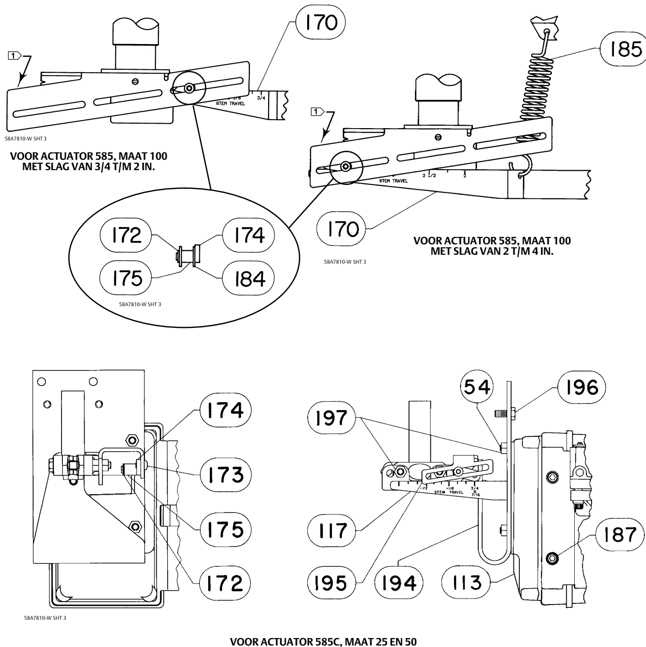
Afbeelding 30. Meenemerconstructies voor Fisher 3611JP- en 3621JP-klepstandsteller
