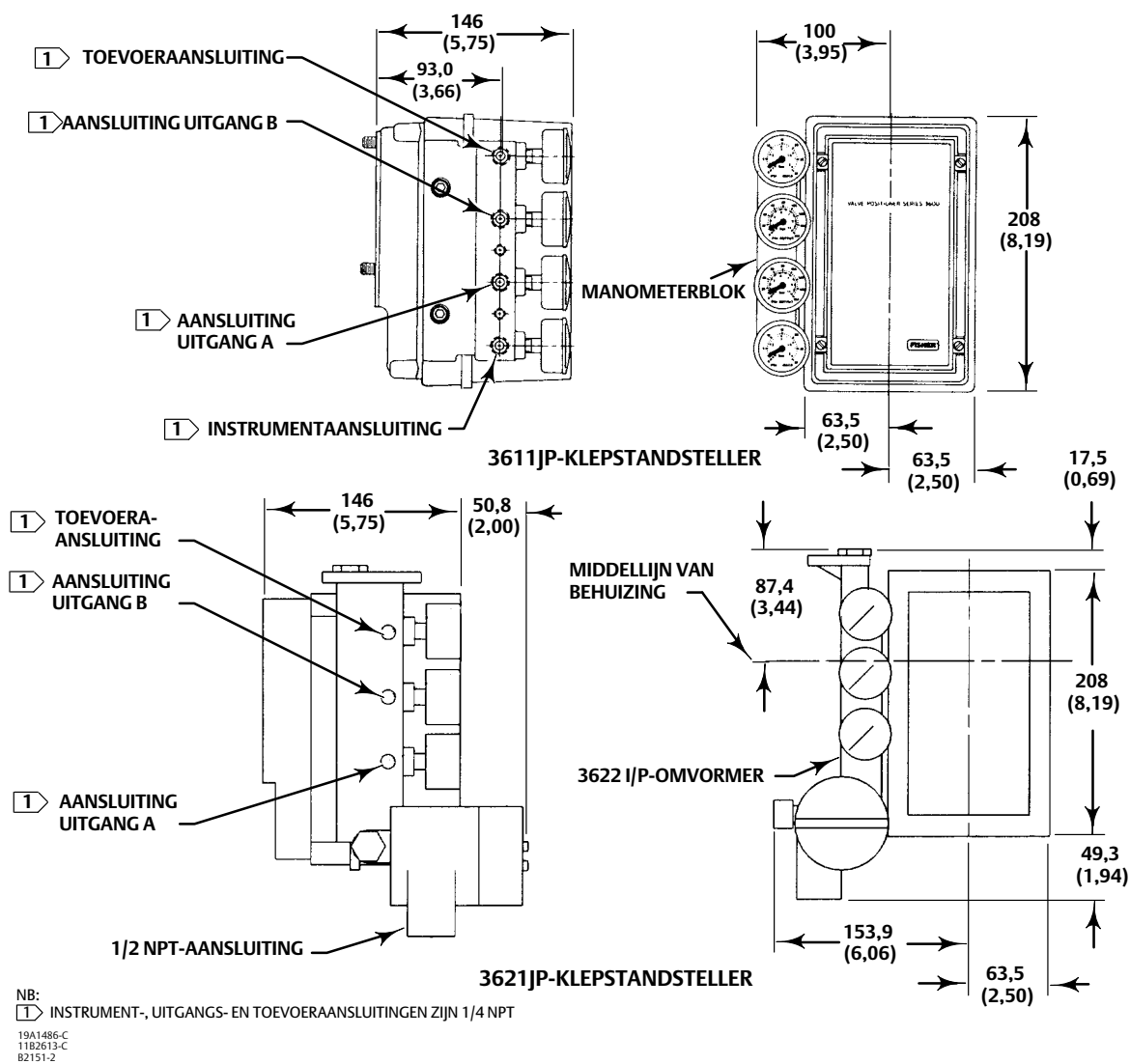
Afbeelding 9. Typische montage-afmetingen en -aansluitingen (vervolg)
