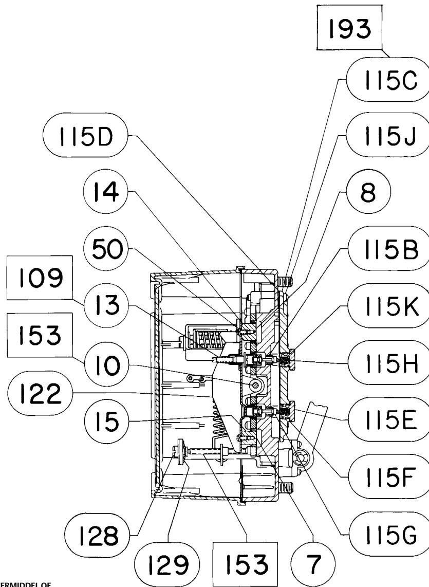
Afbeelding 26. Constructie klepstandstellers (vervolg)
