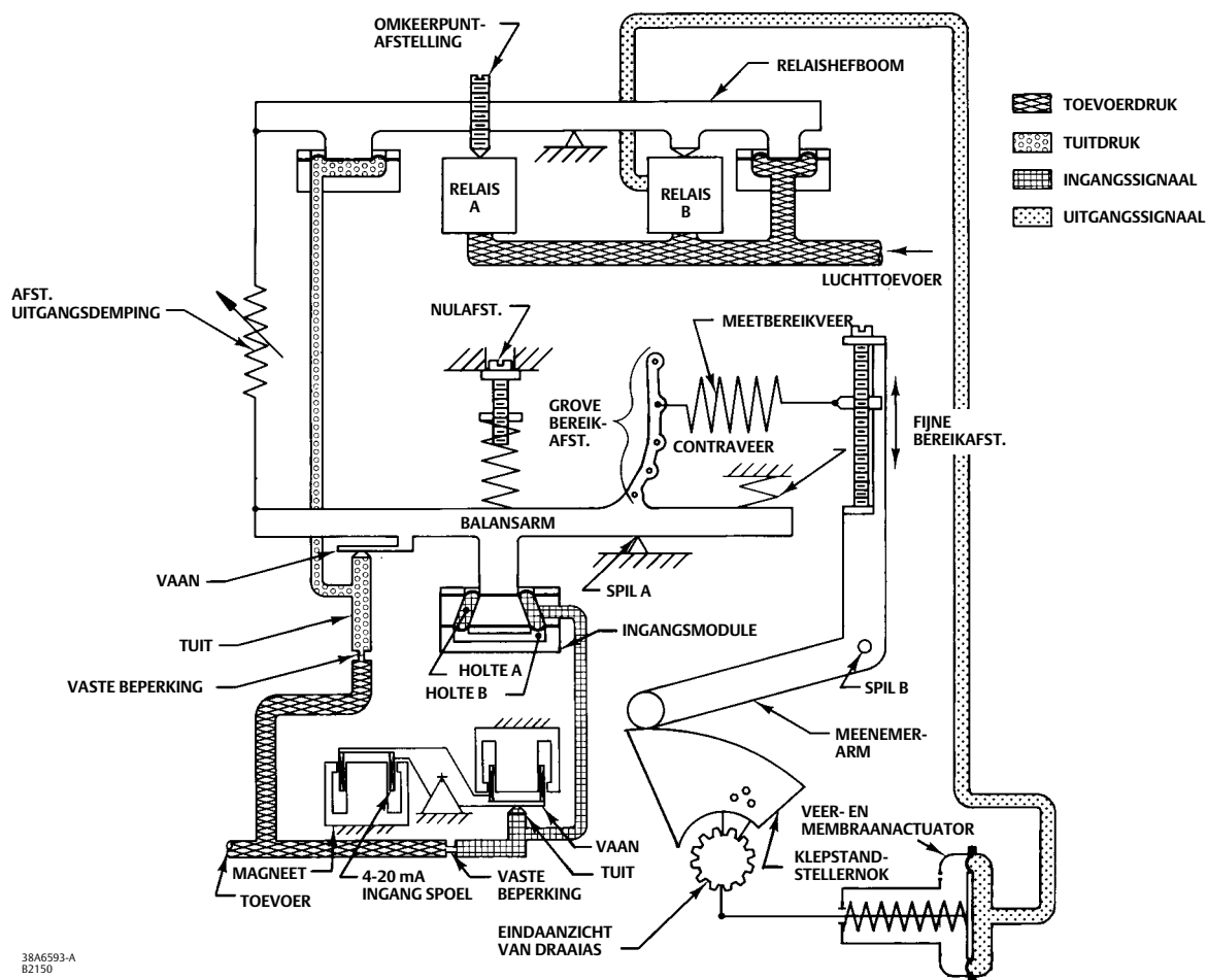
Afbeelding 23. Schema van Fisher 3620J-klepstandsteller
