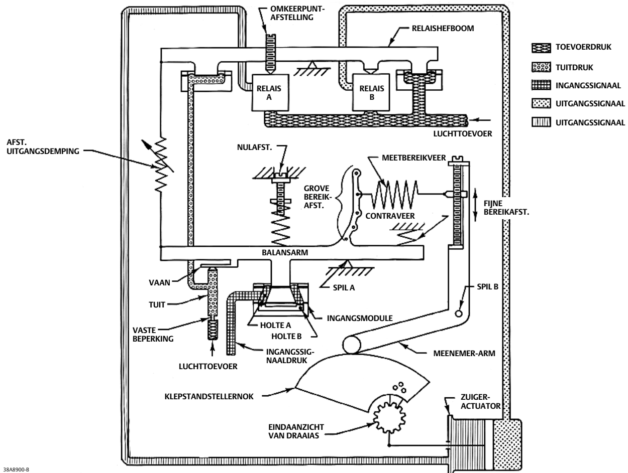
Afbeelding 21. Schema van Fisher 3610JP-klepstandsteller
