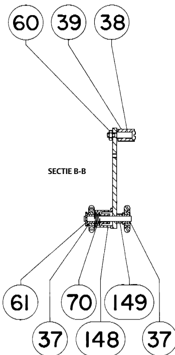
KLEPSTANDSTELLER 3610J EN 3620J VOOR ALLE ACTUATORS 1051 EN 1052 KLEPSTANDSTELLER 3610JP EN 3620JP VOOR ACTUATOR 1061, MAAT 30-60
