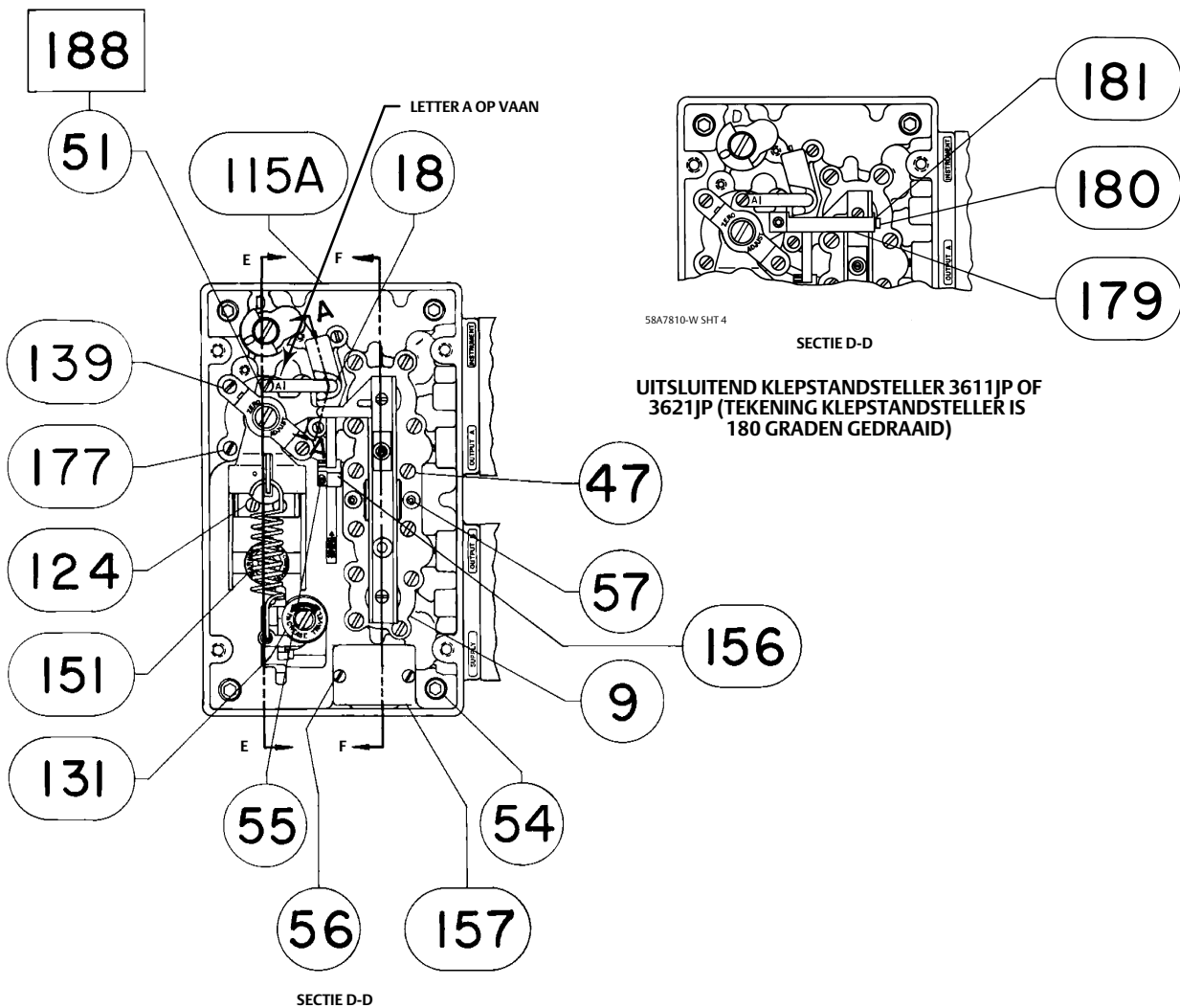
VOORAANZICHT VAN 3610J- EN 3620J-KLEPSTANDSTELLERS WAARBIJ DEKSEL IS VERWIJDERD
