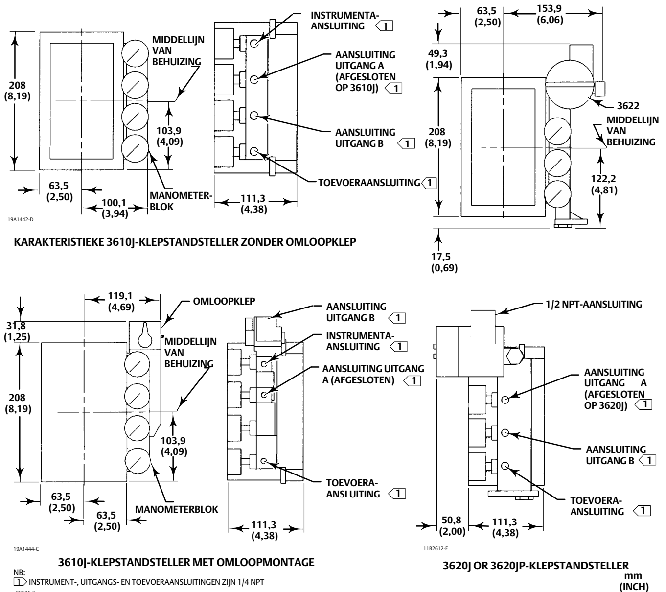
Afbeelding 9. Typische montage-afmetingen en -aansluitingen
