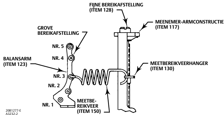
Afbeelding 16. Bereikafstelling
