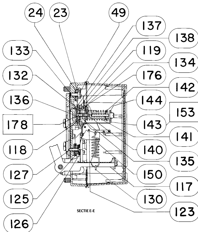
Afbeelding 26. Constructie klepstandstellers (vervolg)
