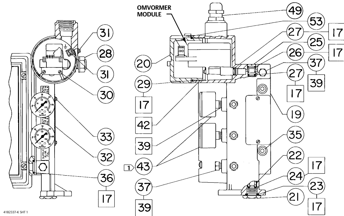
Afbeelding 31. Fisher elektropneumatische 3622-omvormer
