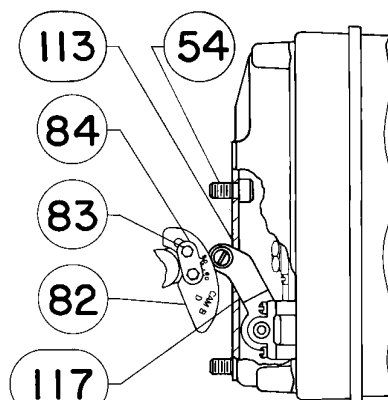
KLEPSTANDSTELLER 3610J EN 3620J VOOR ACTUATOR 1051, MAAT 33 VOOR ACTUATOR 1052, MAAT 20 EN 33
