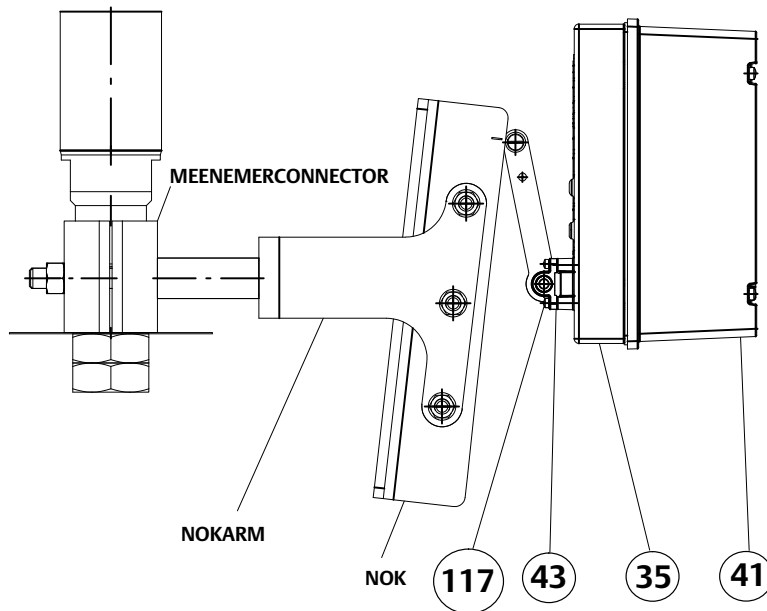
KLEPSTANDSTELLERS 3610JP EN 3620JP VOOR 585C MAAT 60 EN HOGER RAADPLEEG VOOR ANDERE ACTUATORS DE SPECIFIEKE MONTAGEKITTEKENING VOOR MEER INFORMATIE.
