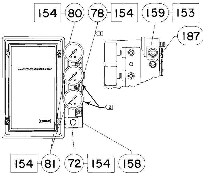
Afbeelding 27. Manometerblok- en omloopklepconstructie
