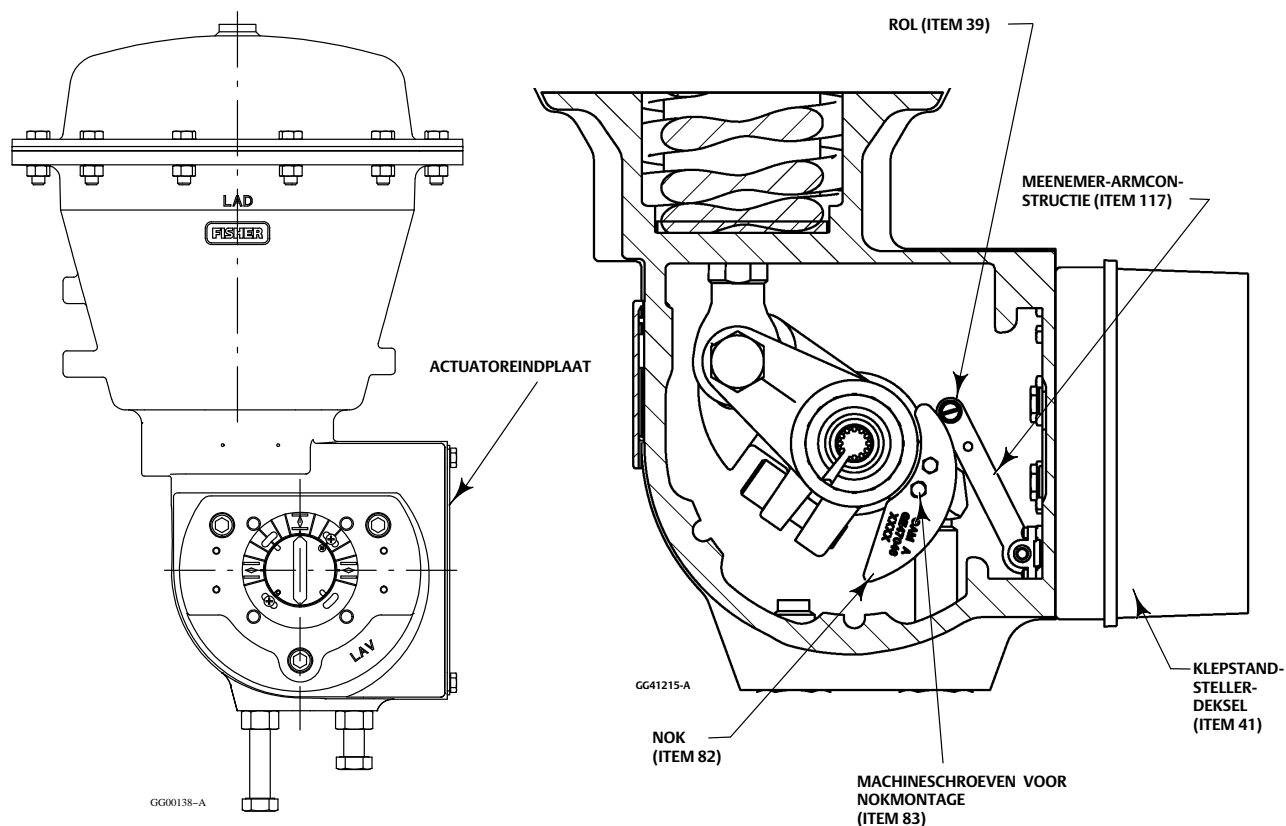
ACTUATOR ZONDER KLEPSTANDSTELLER
