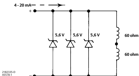
Afbeelding 12. Vervangingscircuit voor Fisher 3622-omvormer
