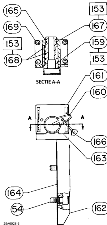
OMLOOPKLEPCONSTRUCTIE VOOR KLEPSTANDSTELLER 3610J
