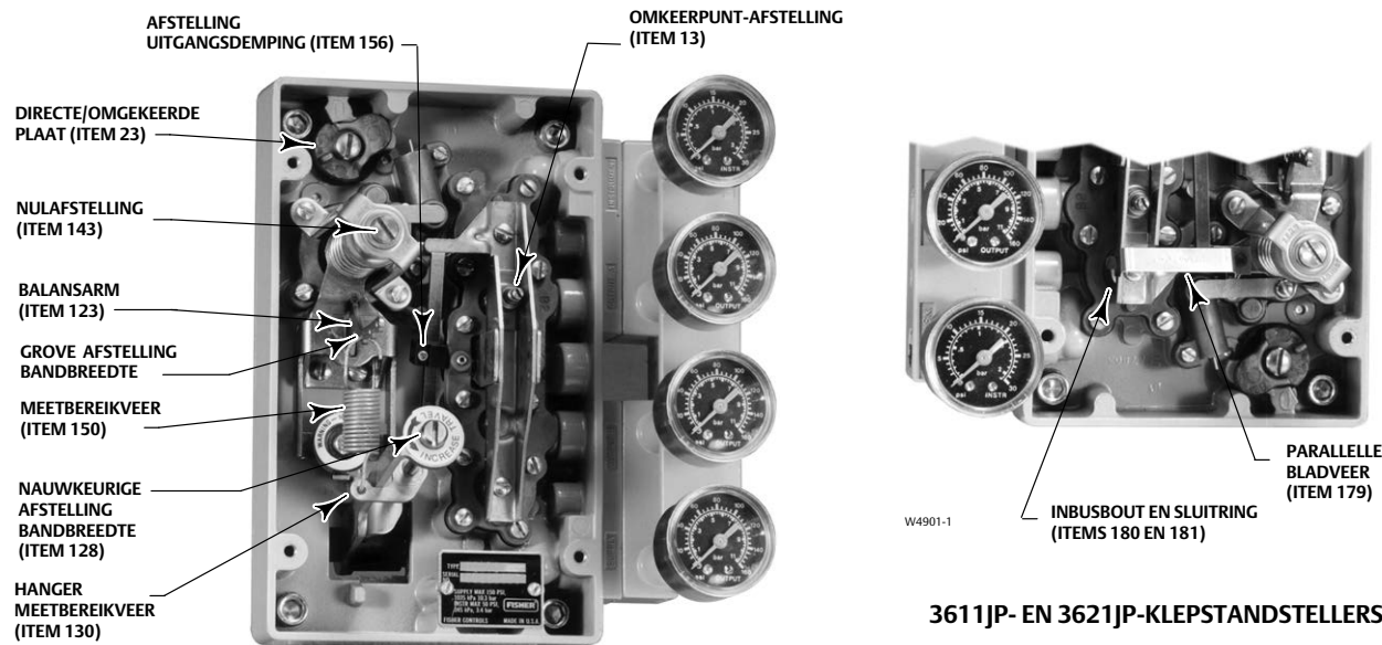
3610J-, 3610JP-, 3620J- EN 3620JP-KLEPSTANDSTELLERS
