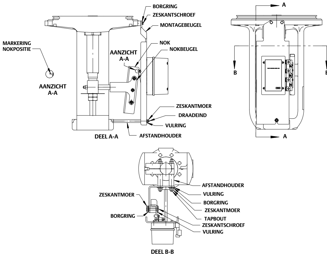
Afbeelding 7. Typische montagegegevens voor Fisher 3610JP- en 3620JP-klepstandstellers op actuators met schuivende steel met lange slag
