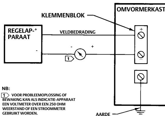
Afbeelding 13. Karakteristiek veldbedradingscircuit
