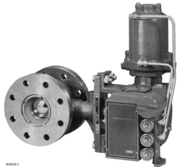
KLEPSTANDSTELLER 3620JP MET FISHER-ACTUATOR 1061 EN KLEP V500
