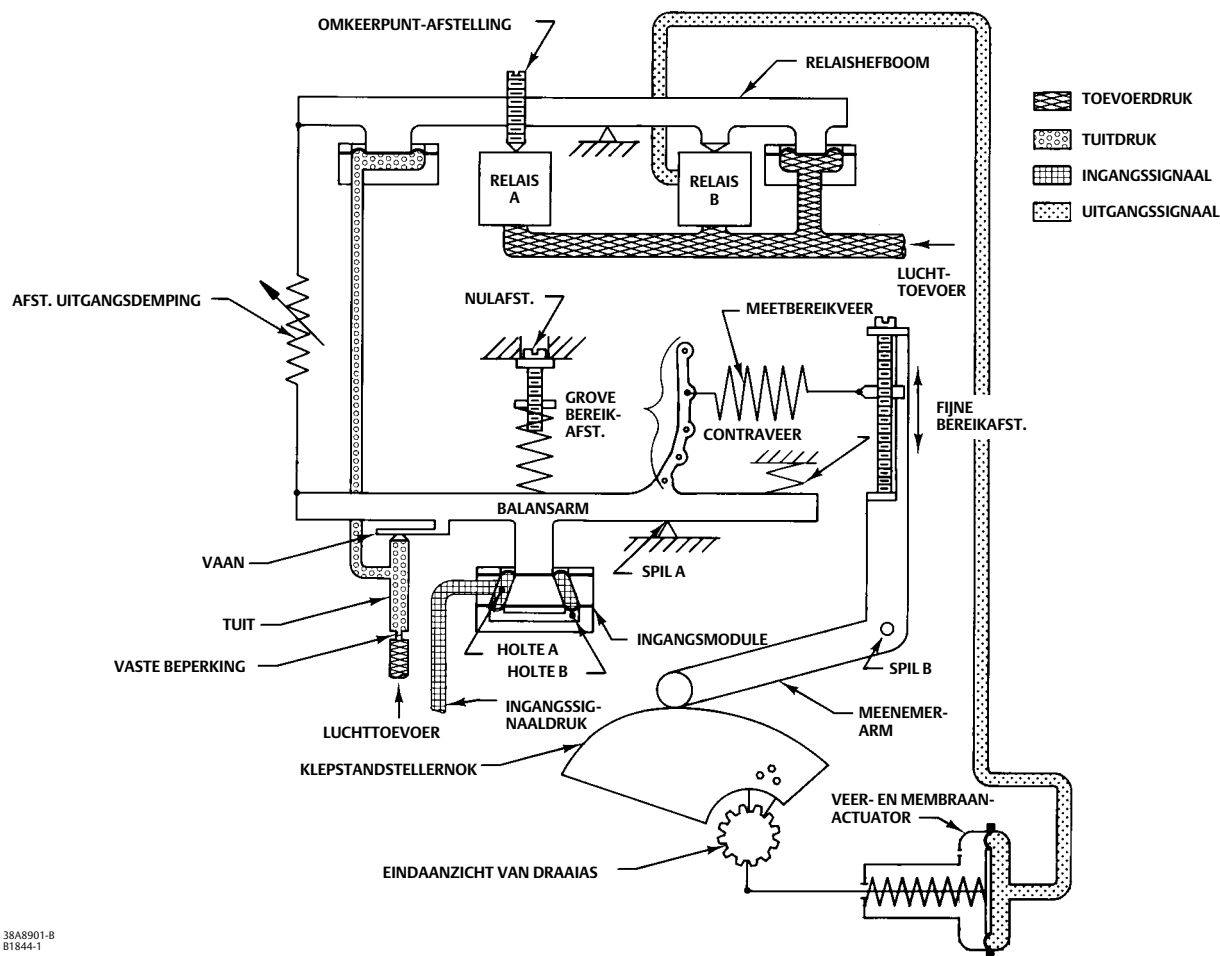
Afbeelding 20. Schema van Fisher 3610J-klepstandsteller
