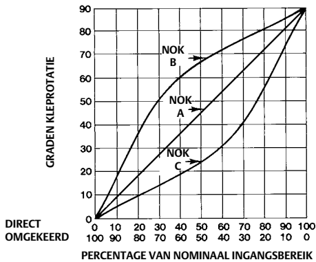
Afbeelding 19. Flowkarakteristieken voor de diverse nokken wanneer gebruikt met klep met gelijk-percentegekarakteristiek die omlaag wordt gedruwd om te sluiten
