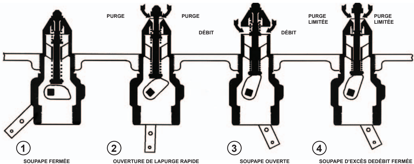
Figure 3. Schéma de Fonctionnement
