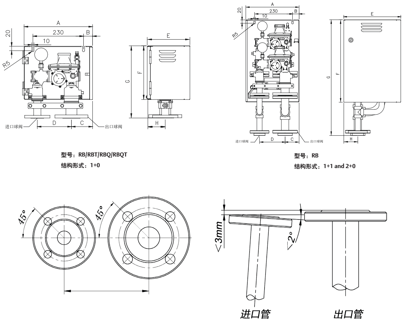
图4. 安装尺寸图
